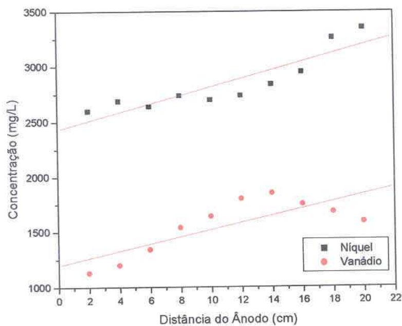
Figura 35: EXPERIMENTO 8 - Concentração de Metais (mg/L) em função do Distância (cm) para C_{H_2SO_4} = 2,0 Mol/L na Condição de Potencial Elétrico para um Tempo de Experimento de 96 h Analisados por FRX.
