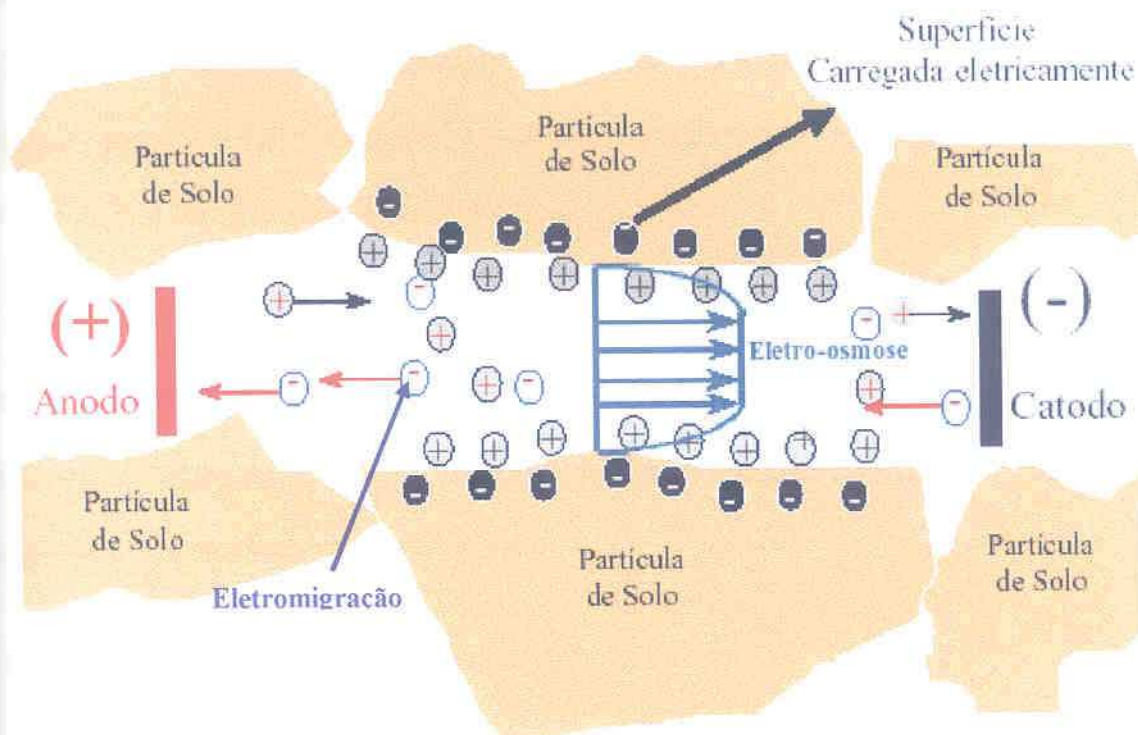
Figura 11: Eletroosmose e Eletromigração de Íons (Acar e Alshawabkeh, 1996)
