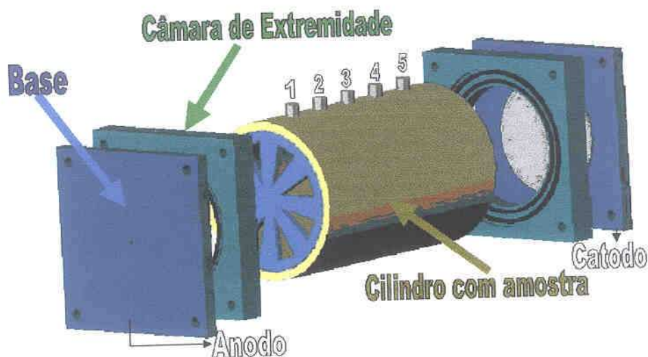
Figura 16: Representação Esquemática do Reator Eletrocínético Utilizado
