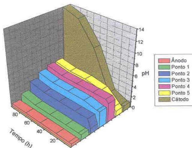
Figura 32: EXPERIMENTO 2 - pH em função do Tempo (h) para C_{H_2SO_4} = 0,5 Mol/L para Potencial Elétrico
