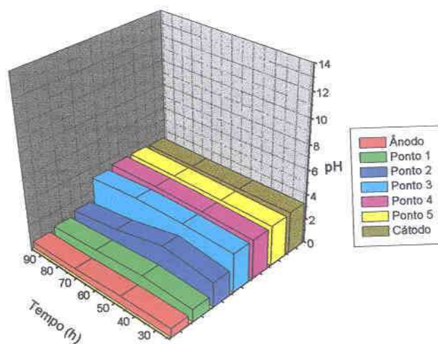
Figura 26: EXPERIMENTO 1 - pH em função do Tempo (h) para C_{H_2SO_4} = 0,5 Mol/L para Lavagem Ácida
