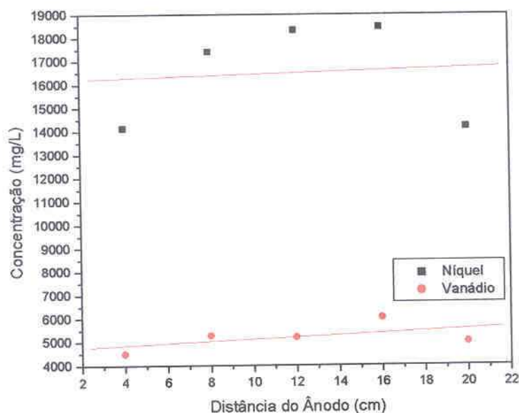
Figura 31: EXPERIMENTO 2 - Concentração de Metais (mg/L) em função da Distância (cm) para C_{H_2SO_4} = 0,5 \text{ Mol/L} na Condição de Potencial Elétrico para um Tempo de Experimento de 96 h Analisados por FRX
