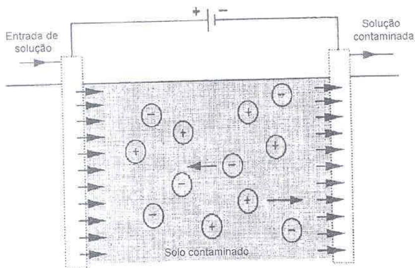
Figura 14: Conceito da extração eletrocinética de contaminantes (YEUNG, 1997)
