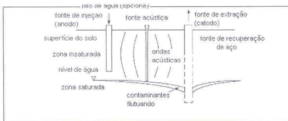
Figura 4: Processo eletroacústico de descontaminação do solo (Innovative in situ cleanup process, 1992 in EPA, 1997)
