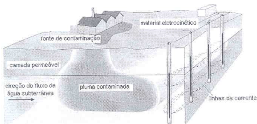
Figura 1: Esquema da pluma contaminada e estacionada por um material eletrocinético (Gill in EPA, 1997)
