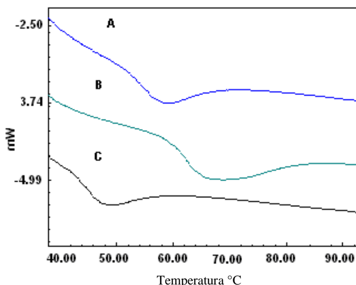
Figura 11- DSC Endotermas de gelatinização de diferentes amidos: (A) mandioquinha; (B) mandioca e (C) maca.
