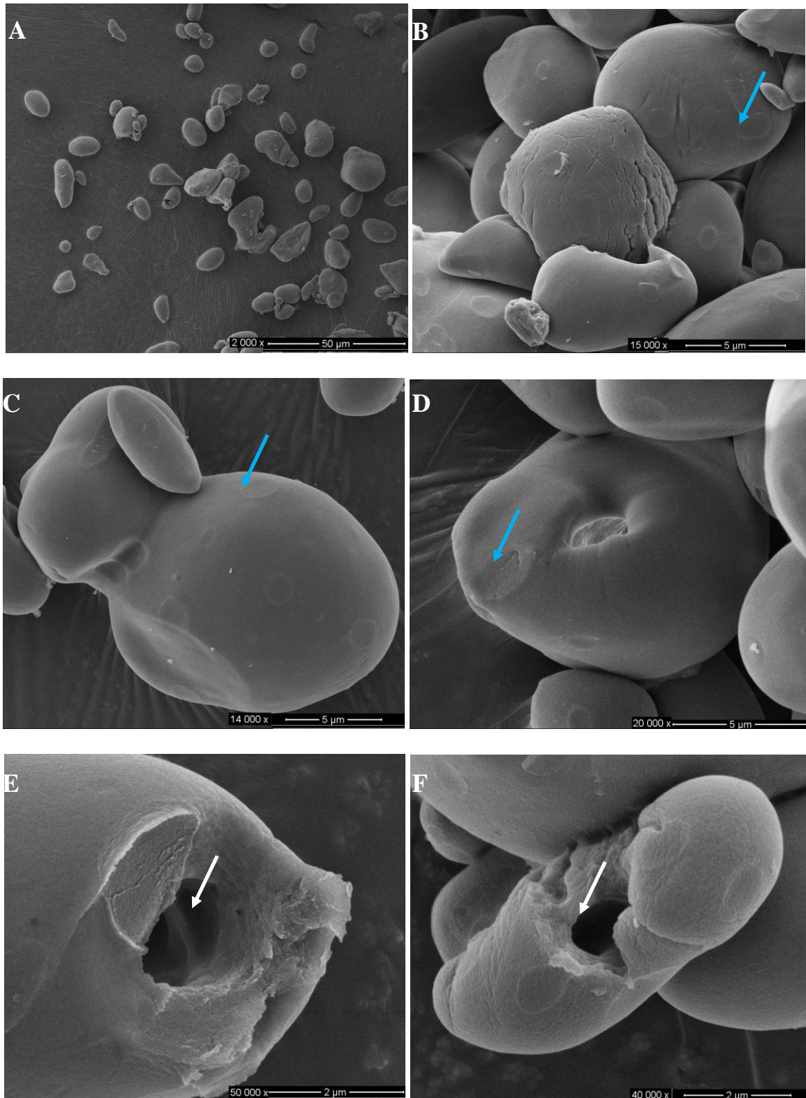
Figura 28 – Micrografias em MEV do amido nativo de maca hidrolisados com o extrato bruto da própria raiz (1mL de extrato bruto/g de amido) em tampão fosfato 0,01 M pH 6,0 durante 2 horas a 30
