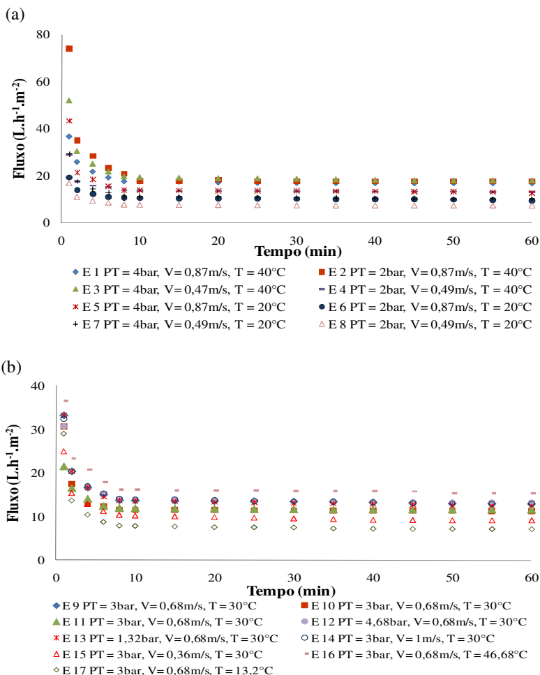
Figura 3 Comportamento do fluxo do permeado ( J ) durante a microfiltração de caldo de cana adicionado de polpa de maracujá (a) para os ensaios 1 a 8; (b) para os ensaios 9 a 17.
