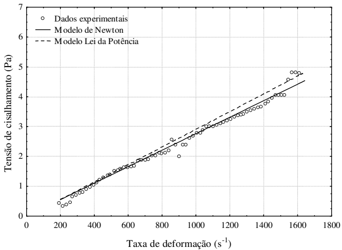
Figura 2 Representação gráfica do ajuste aos modelos de Newton e da Lei da Potência para os dados de tensão de cisalhamento em função da taxa de deformação para: (a) o caldo microfiltrado , (b) caldo pasteurizado P1 e (c) caldo pasteurizado P2 na temperatura de 10 °C
