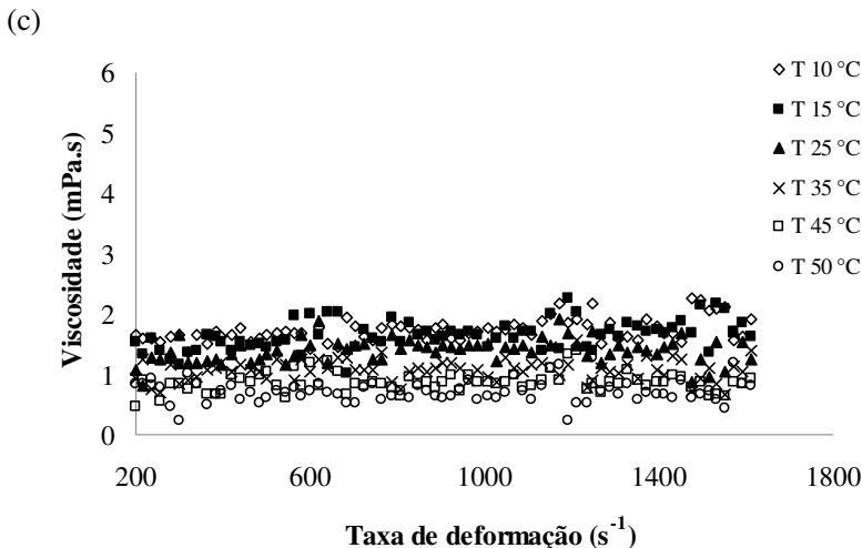
Figura 1 Comportamento reológico do (a) caldo de cana pasteurizado P1 (90 °C/30 s); (b) caldo de cana pasteurizado P2 (95 °C/30 s) e (c) caldo de cana microfiltrado nas diferentes temperaturas estudadas.
