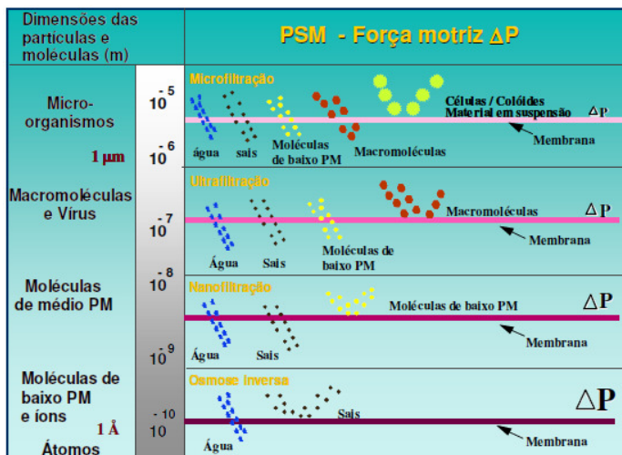
Figura 2 Classificação dos Processos de Separação com Membranas quanto a sua seletividade.
