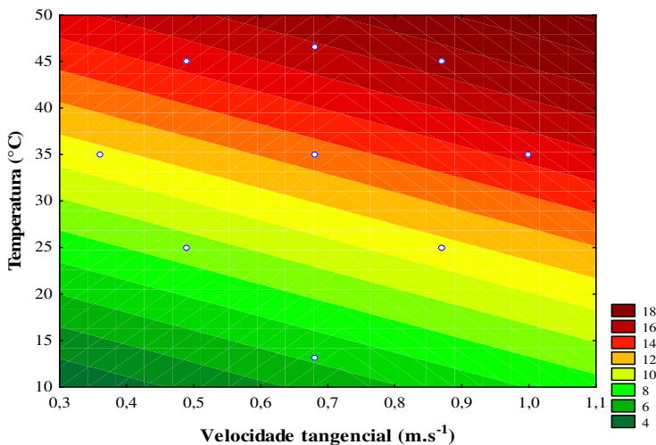
Figura 6 (a) superfície de resposta - influência dos fatores (temperatura e velocidade) na microfiltração de caldo de cana acidificado; (b) superfície de contorno com vista superior.
