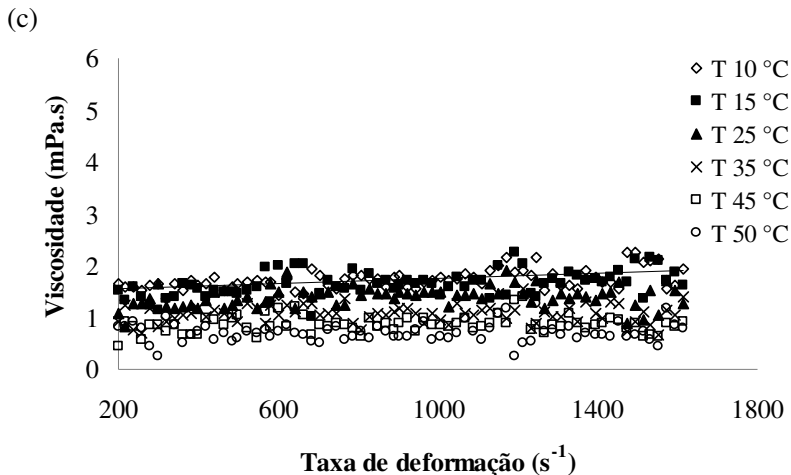
Figura 10 Relação da viscosidade aparente versus taxa de deformação nas temperaturas de 10, 15, 25, 35, 45 e 55 °C, para o (a) caldo de cana in natura ; (b) caldo de cana acidificado e (c) caldo de cana microfiltrado.
