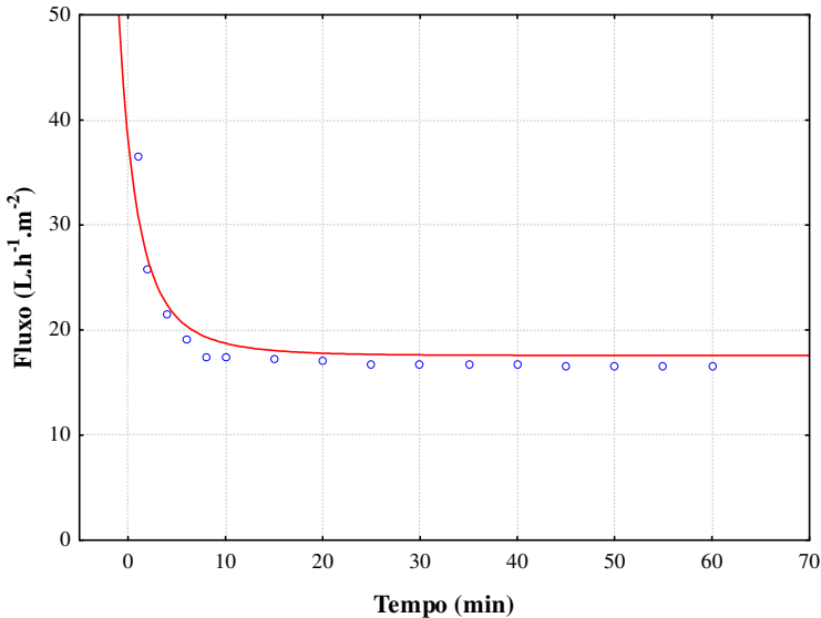
Figura 9 Ajuste da curva de fluxo de permeado ao modelo de: Constenla e Lozano (1997) para o experimento 1 [dados experimentais (o), valores calculados (-)].
