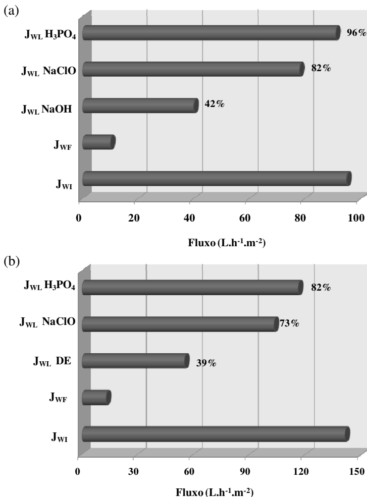
Figura 7 (a) Recuperação de fluxo após cada etapa de limpeza para o Procedimento 1 [NaOH (1 %), NaClO (200 ppm) e H_3PO_4 (200 ppm)];
