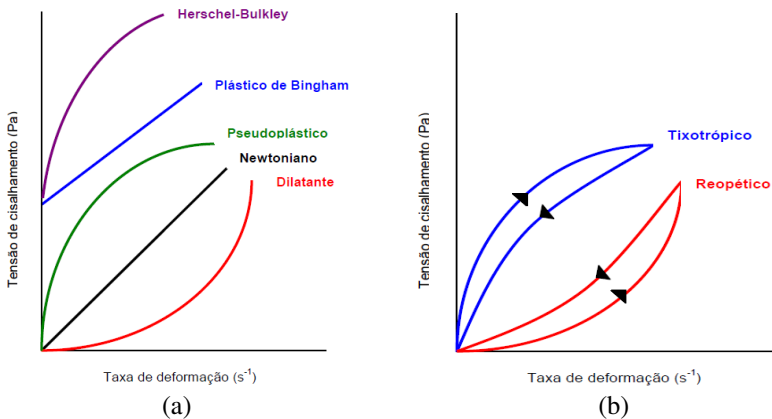
Figura 6 Curva de fluxo de alguns tipos de fluidos (a) independentes do tempo e (b) dependentes do tempo.
