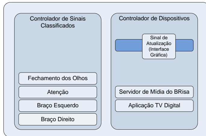
Figura 3.21: Representação do cenário em que o componente relativo ao dispositivo selecionado mapeia o evento recebido em um sinal de atualização para a interface gráfica usada para realimentar o usuário
