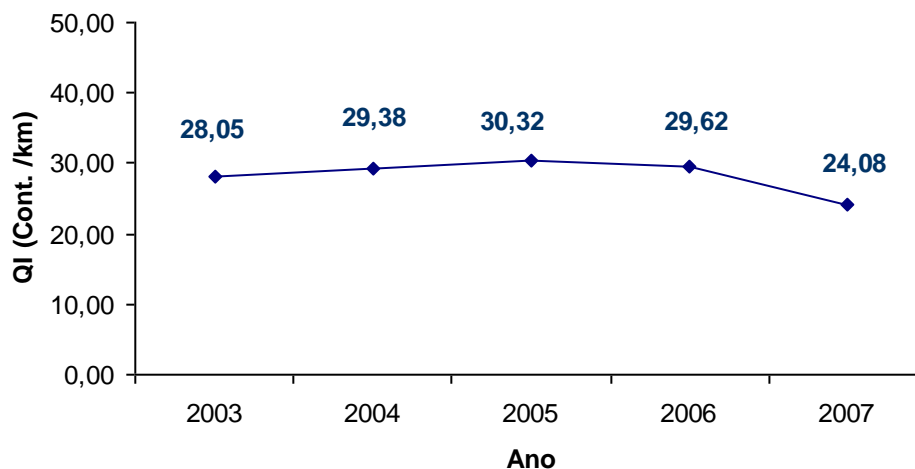
Figura 152 – Evolução QI, “Queiroz B”, Trecho 04
