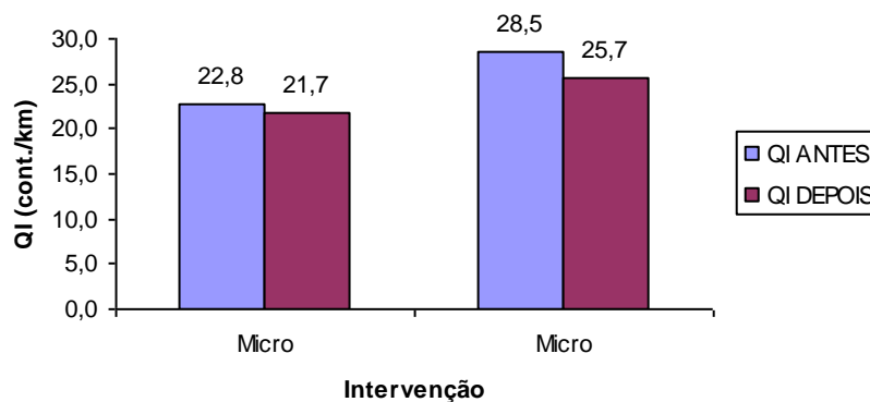
Figura 162 – QI após intervenção, Trecho 03
