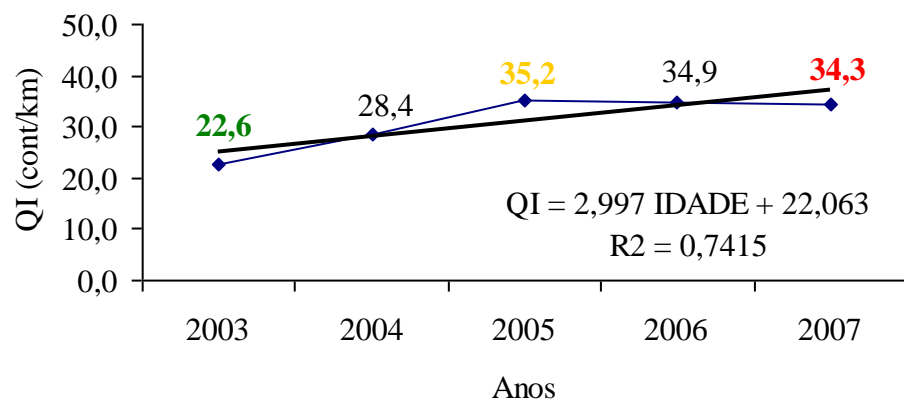
Figura 21 – Evolução irregularidade longitudinal – Trecho 01
