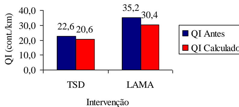
Figura 31 – QI após intervenção, Trecho 01.
