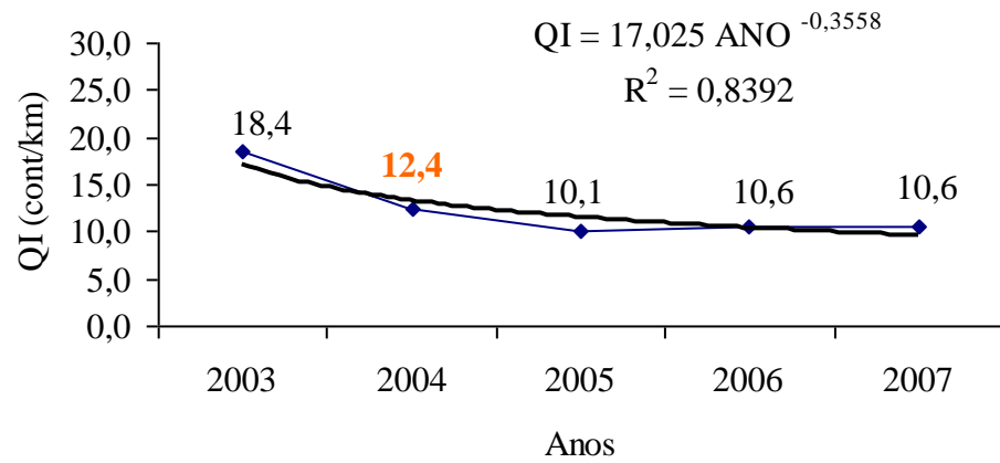
Figura 22 – Evolução Irregularidade longitudinal – Trecho 02
