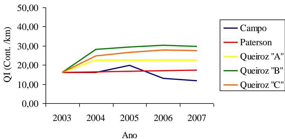
Figura 47– Evolução da irregularidade longitudinal prevista e real – Trecho 04
