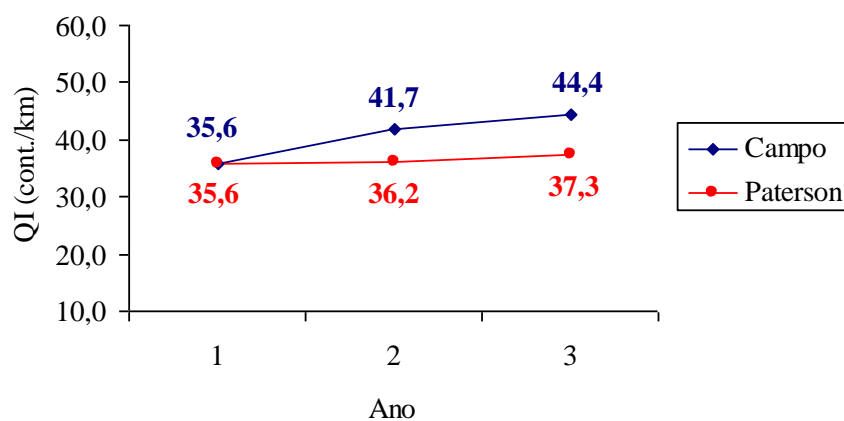
Figura 43 – Evolução irregularidade, escala real e Paterson, 1987 – Trecho 06
