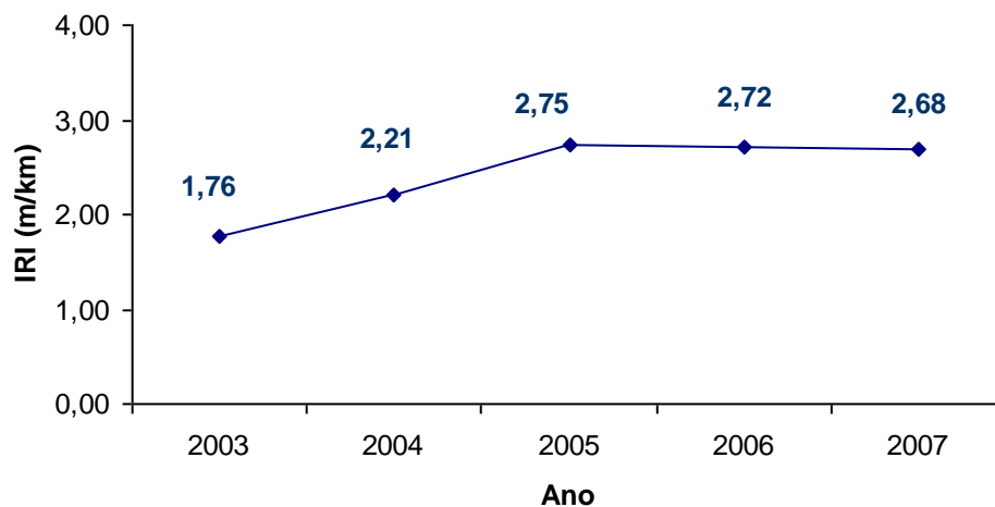
Figura 136 – Evolução da IRI, Trecho 01
