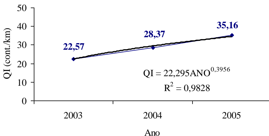
Figura 34 - Evolução do QI com Tratamento Superficial Duplo, Trecho 01
