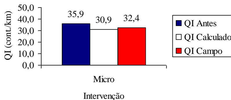
Figura 51 – QI antes da restauração, QI calculado e calculado e QI médio - Trecho 05
