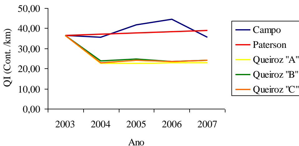
Figura 49 – Evolução da irregularidade longitudinal prevista e real – Trecho 05
