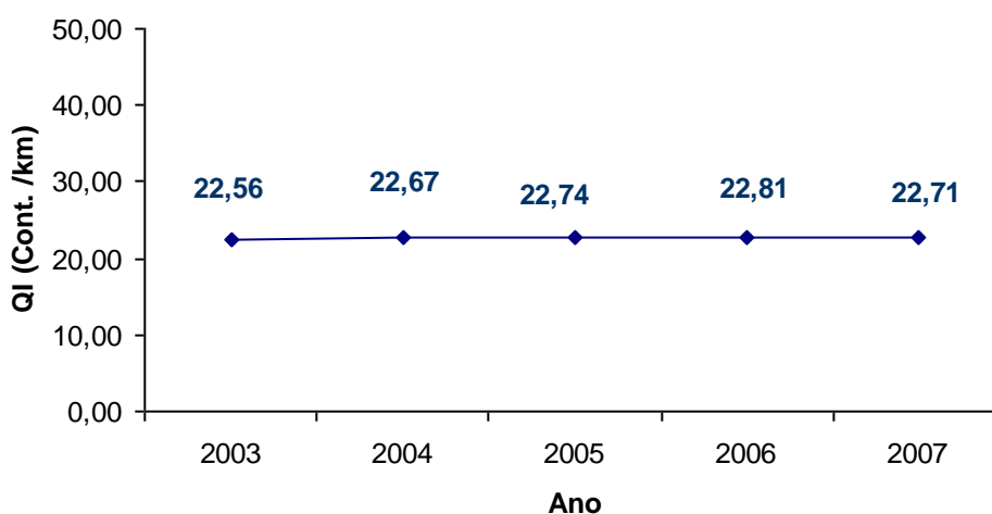
Figura 157 – Evolução QI, “Queiroz A”, Trecho 06
