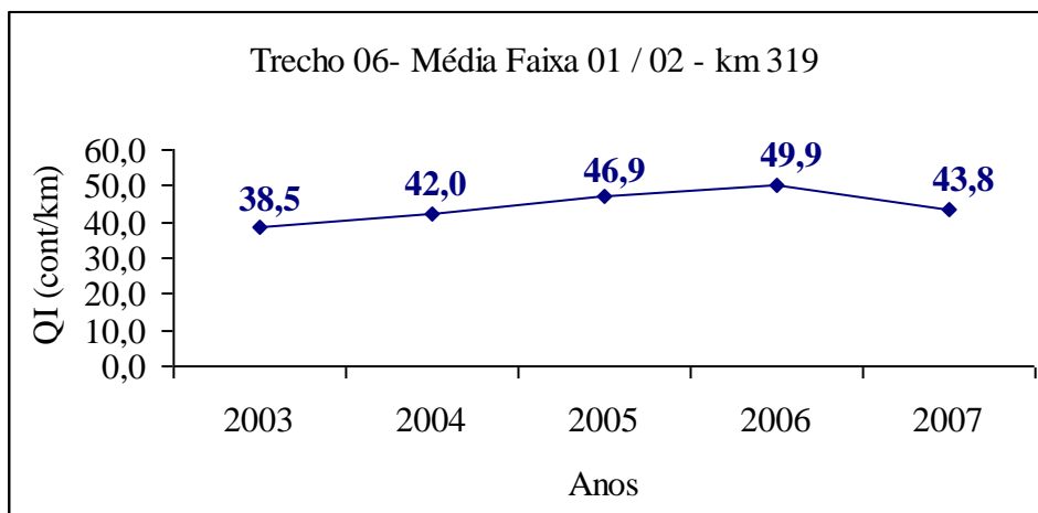
Figura 132 - Trecho 06, Média Faixa 01 / 02 - Km 319
