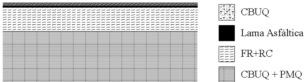
Figura 14 - Detalhamento estrutura do pavimento - Trecho 05
