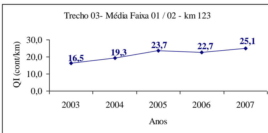
Figura 101 - Trecho 03, Média Faixa 01 / 02 - Km 123
