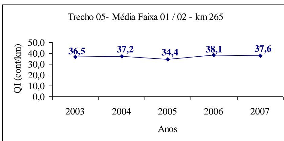
Figura 125 - Trecho 05, Média Faixa 01 / 02 - Km 265
