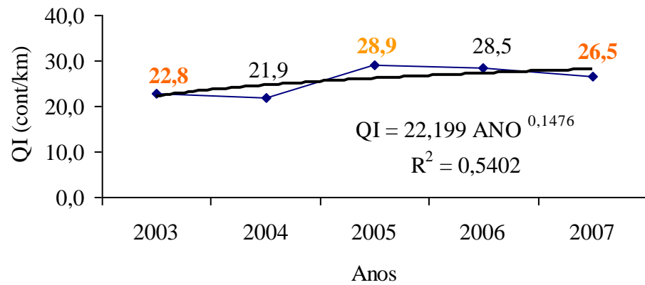
Figura 23 – Evolução Irregularidade longitudinal – Trecho 03
