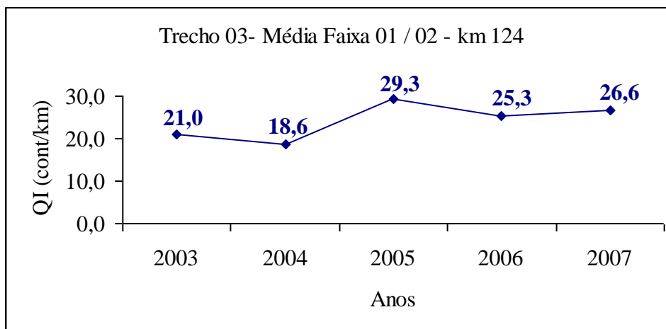
Figura 102 - Trecho 03, Média Faixa 01 / 02 - Km 124
