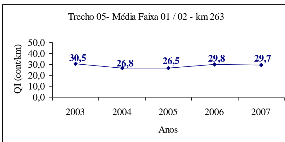
Figura 123 - Trecho 05, Média Faixa 01 / 02 - Km 263
