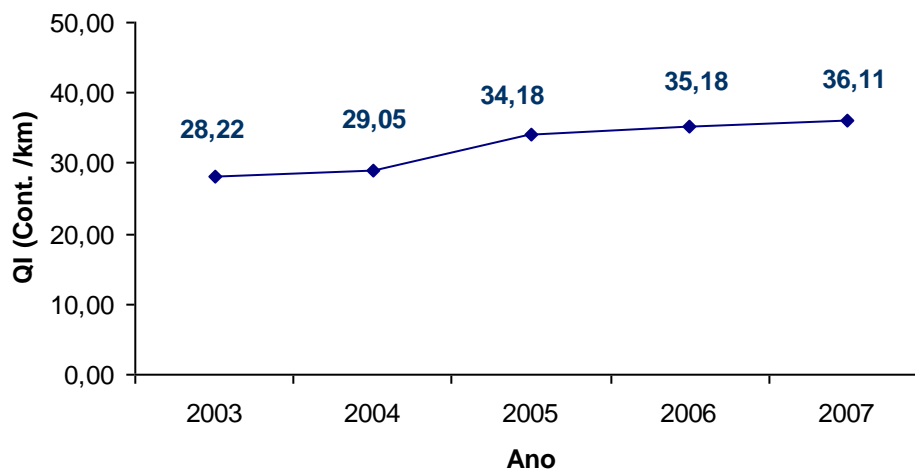
Figura 146 – Evolução QI, “Queiroz B”, Trecho 02
