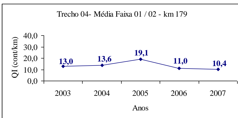
Figura 114 - Trecho 04, Média Faixa 01 / 02, Km 179
