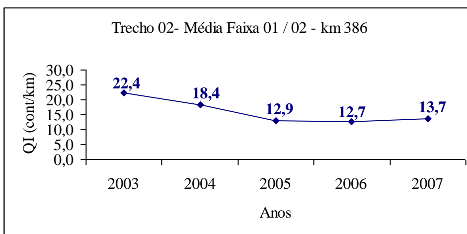
Figura 95 - Trecho 02, Média Faixa 01 / 02 - Km 386
