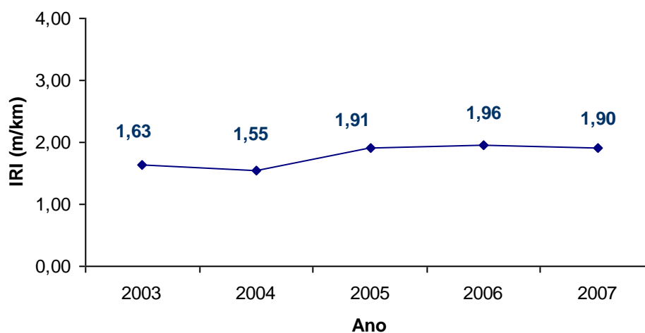
Figura 138 – Evolução IRI, Trecho 03
