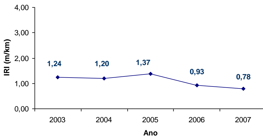
Figura 139 – Evolução IRI, Trecho 04.
