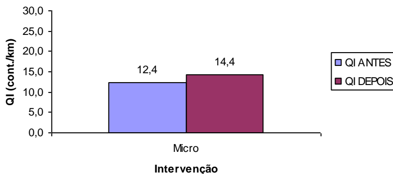
Figura 161 – QI após intervenção, Trecho 02
