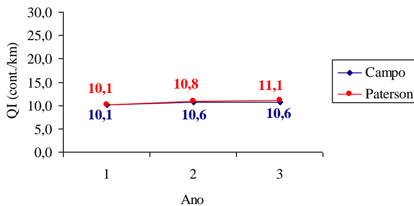
Figura 41 – Evolução irregularidade, escala real e Paterson, 1987 – Trecho 02
