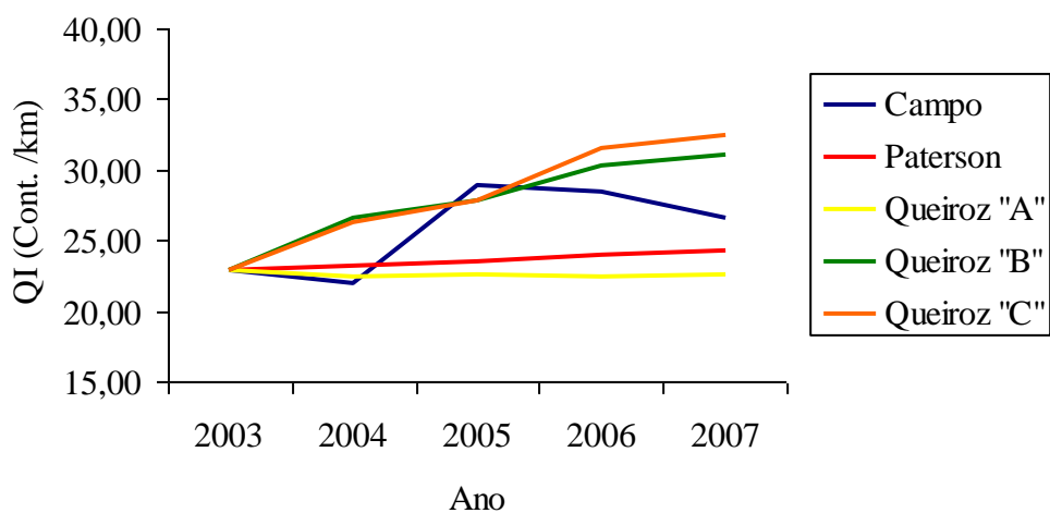
Figura 46 – Evolução da irregularidade longitudinal prevista e real – Trecho 03
