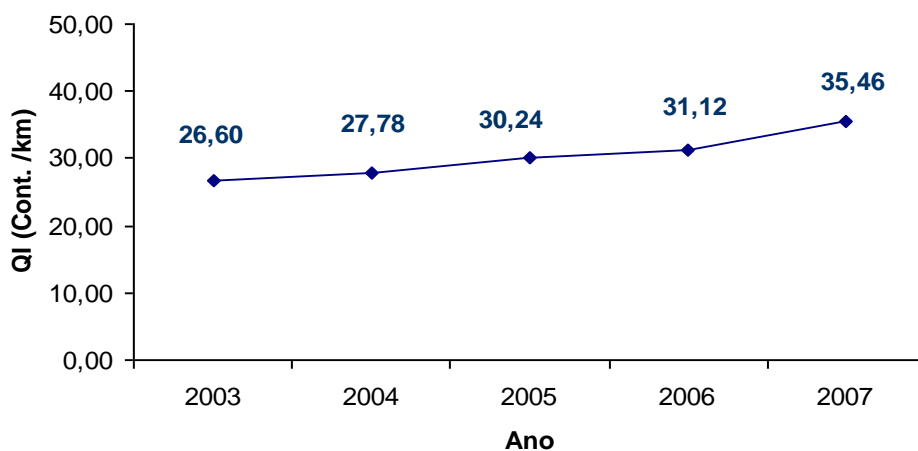
Figura 149 – Evolução QI, “Queiroz B”, Trecho 03
