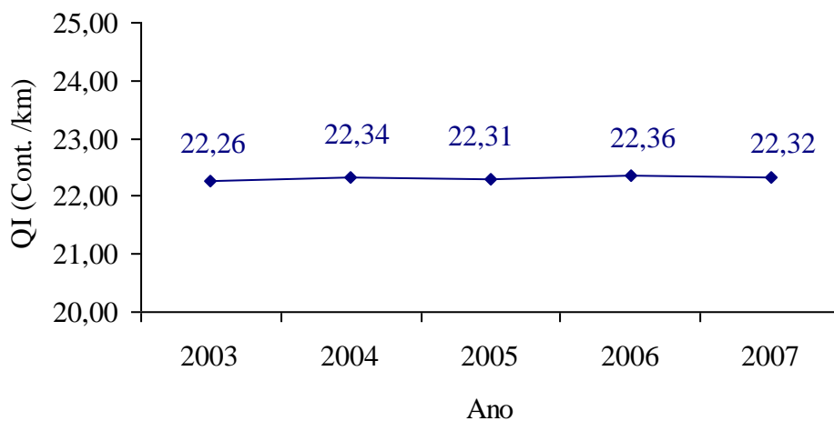
Figura 28 – Evolução da Irregularidade longitudinal “Queiroz A” – Trecho 01
