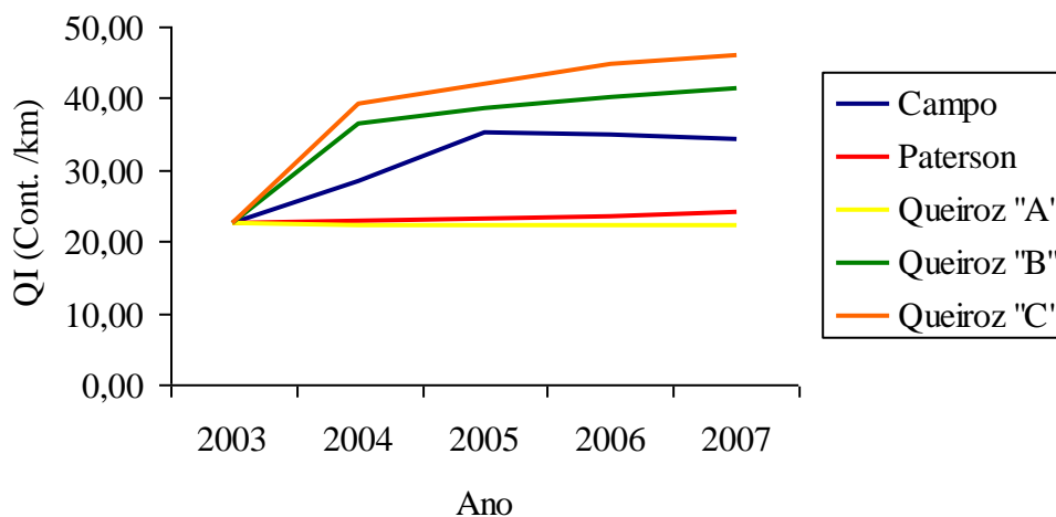
Figura 44 – Evolução da irregularidade longitudinal prevista e real – Trecho 01
