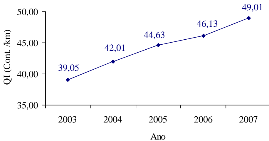
Figura 30 – Evolução da irregularidade longitudinal “Queiroz C”– Trecho 01
