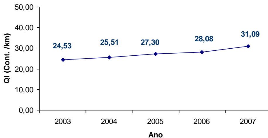
Figura 155 – Evolução QI, “Queiroz B”, Trecho 05
