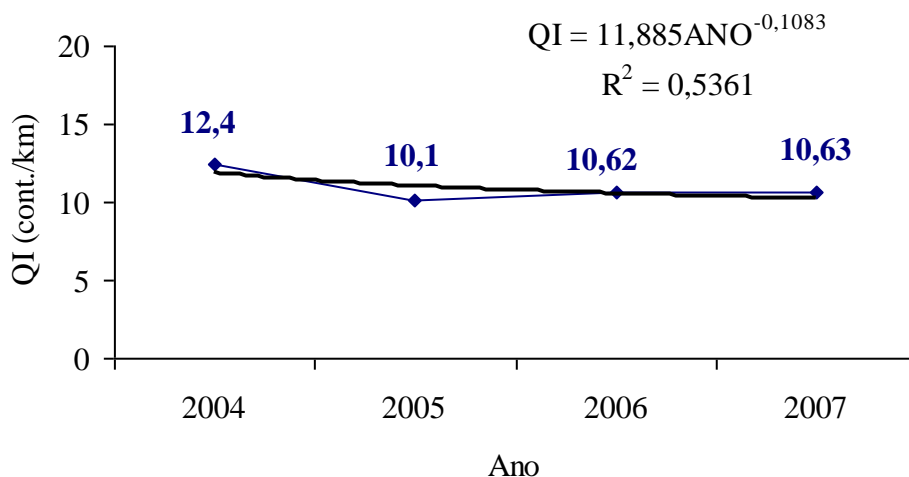
Figura 36 - Evolução do Micro Concreto Asfáltico, Trecho 02
