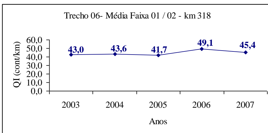
Figura 131 - Trecho 06, Média Faixa 01 / 02 - Km 318
