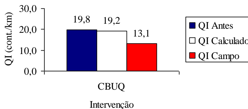
Figura 54 – QI antes da restauração, QI calculado e calculado e QI médio - Trecho 04
