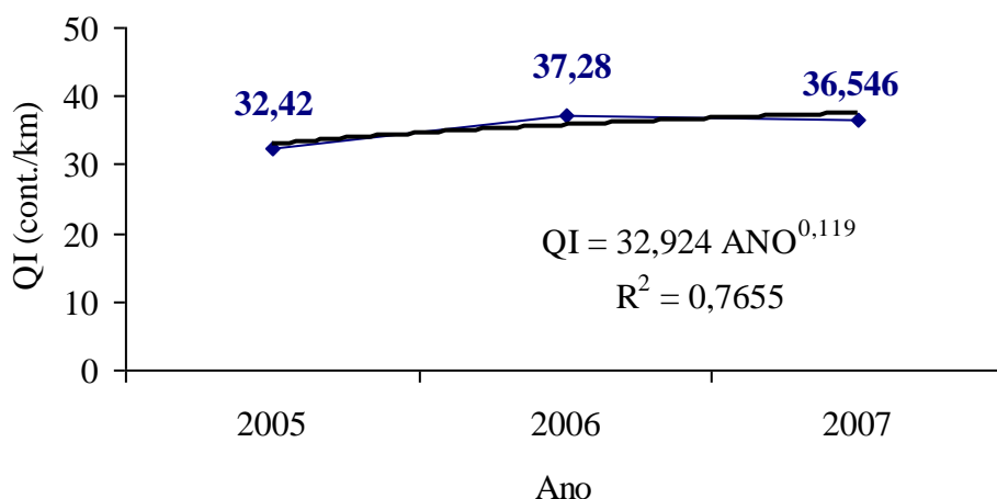
Figura 38 - Evolução do Micro Concreto Asfáltico, Trecho 05
