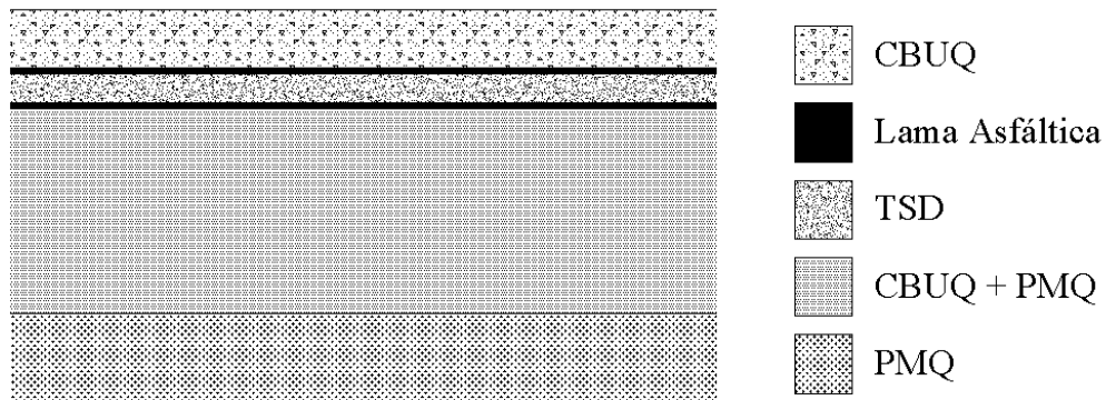
Figura 10 – Detalhamento estrutura do pavimento - Trecho 01
