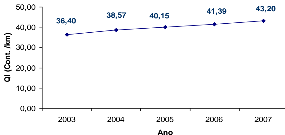
Figura 143 – Evolução QI, “Queiroz B”, Trecho 01
