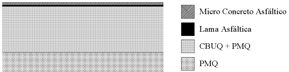
Figura 11 - Detalhamento estrutura do pavimento - Trecho 02
