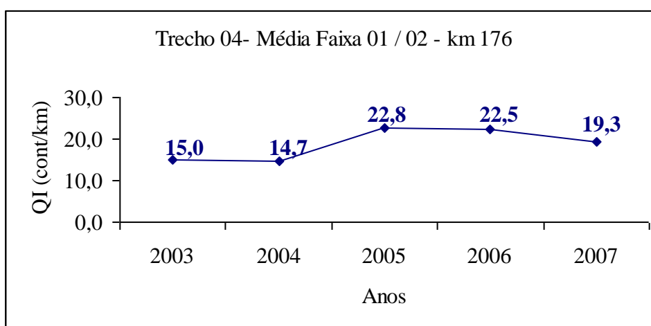
Figura 111 - Trecho 04, Média Faixa 01 / 02, Km 176
