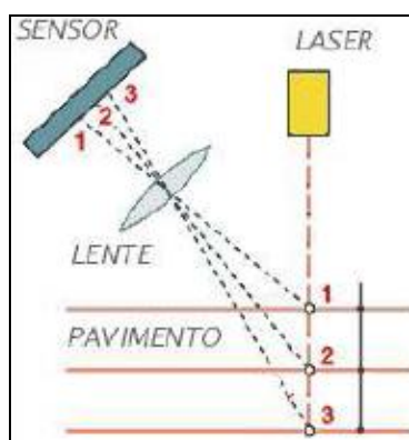
Figura 2 - Desenho esquemático do medidor a laser
