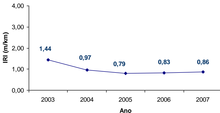
Figura 137 – Evolução IRI, Trecho 02
