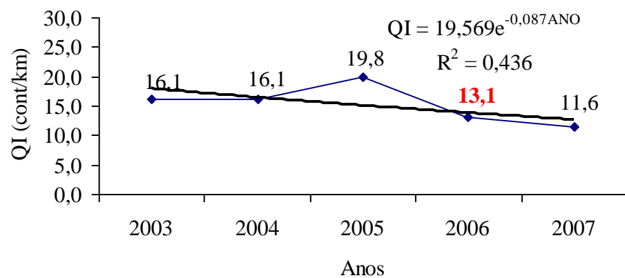
Figura 24 – Evolução Irregularidade longitudinal – Trecho 04
