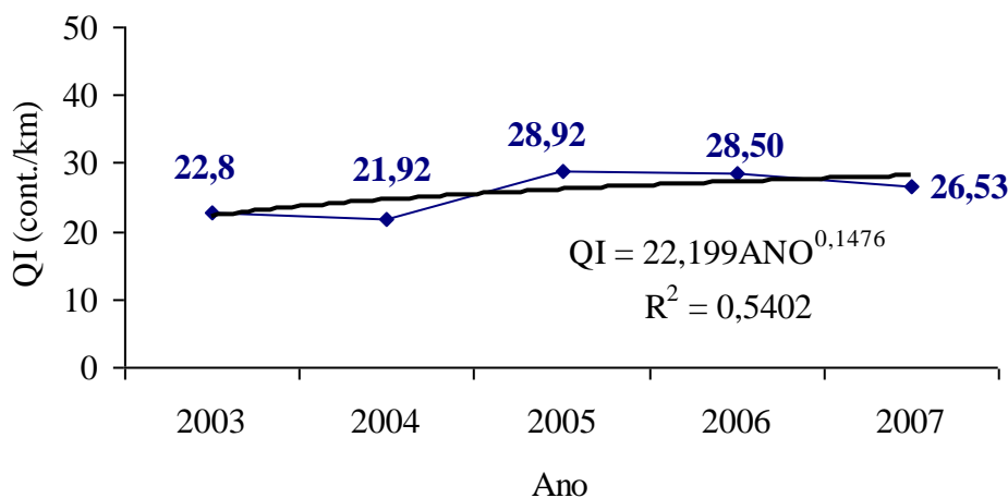
Figura 37 - Evolução das intervenções de micro concreto asfáltico, Trecho 03
