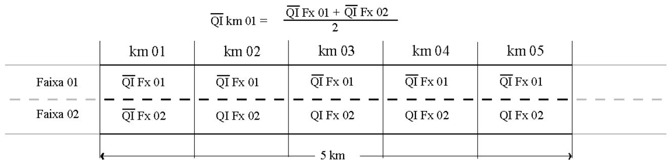
Figura 19 – Médias de QI entre as faixas de rolagem
