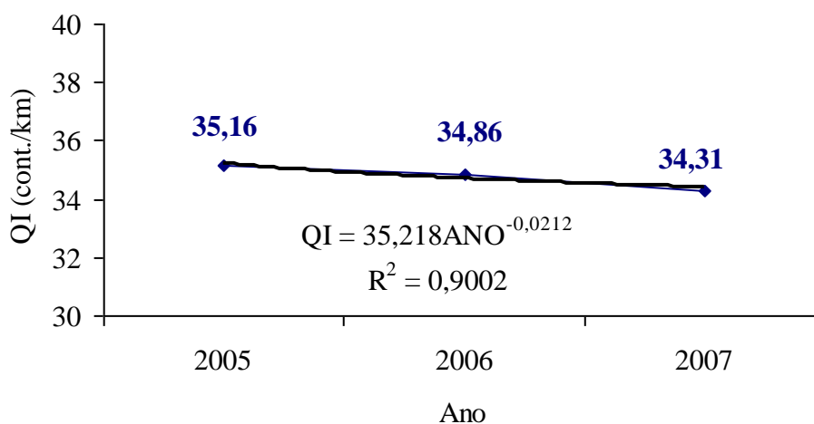
Figura 35 - Evolução da Lama Asfáltica, Trecho 01
