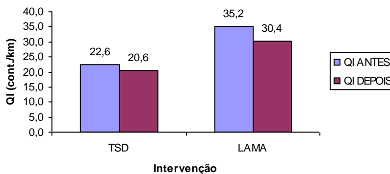
Figura 160 – QI após intervenção, Trecho 01
