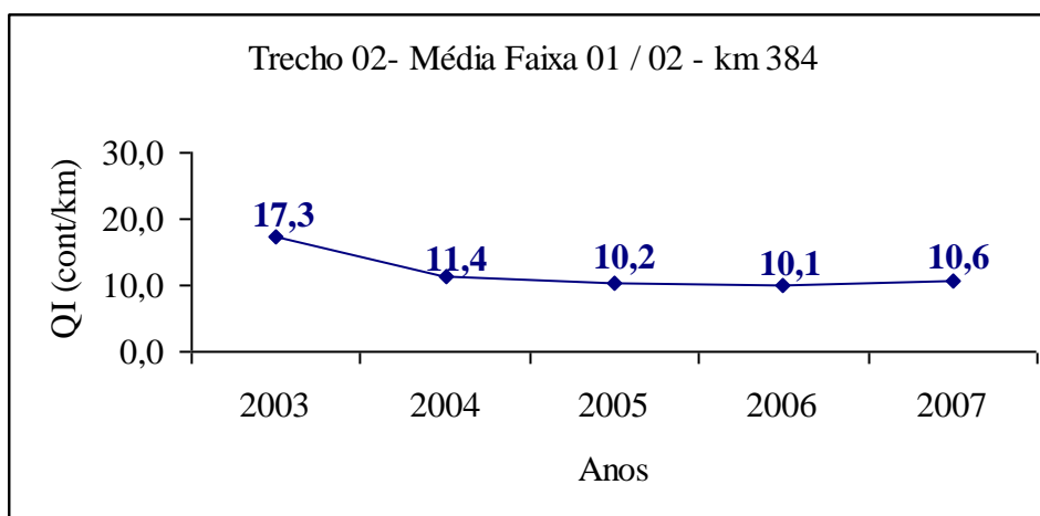
Figura 93 - Trecho 02, Média Faixa 01 / 02 - Km 384
