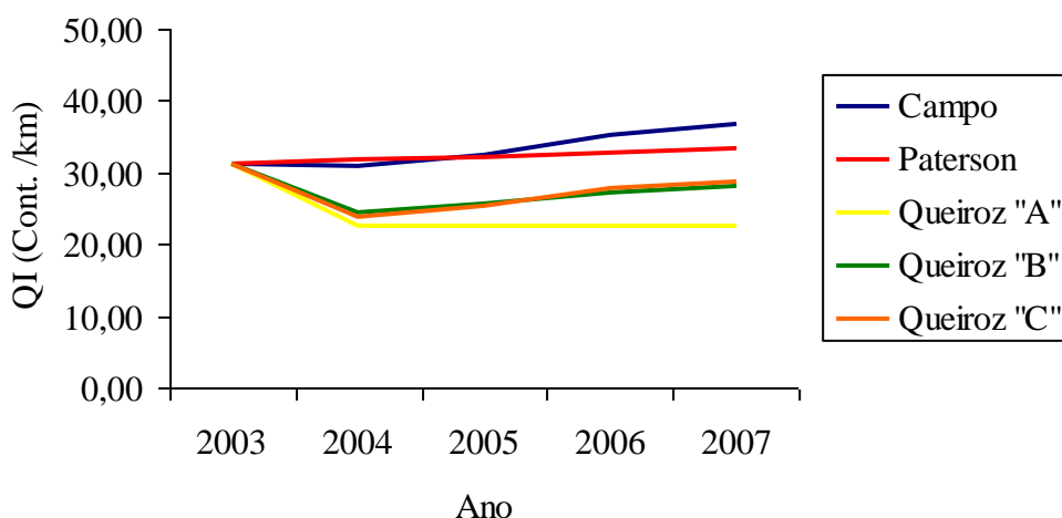
Figura 48 – Evolução da irregularidade longitudinal prevista e real – Trecho 05
