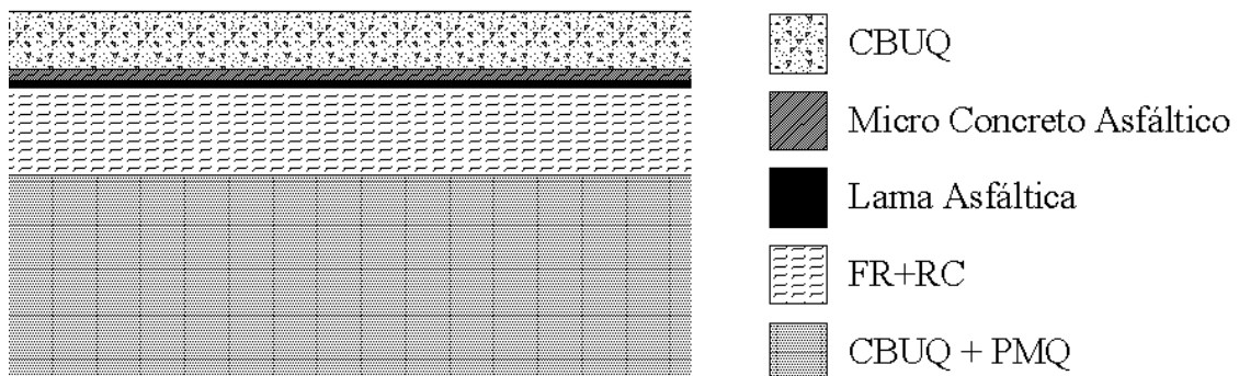
Figura 15 - Detalhamento estrutura do pavimento - Trecho 06
