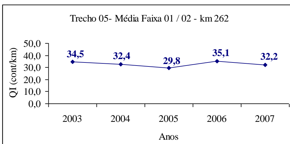
Figura 122 - Trecho 05, Média Faixa 01 / 02 - Km 262
