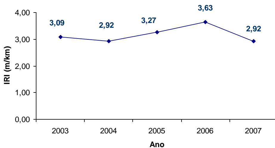
Figura 141 – Evolução IRI, Trecho 06
