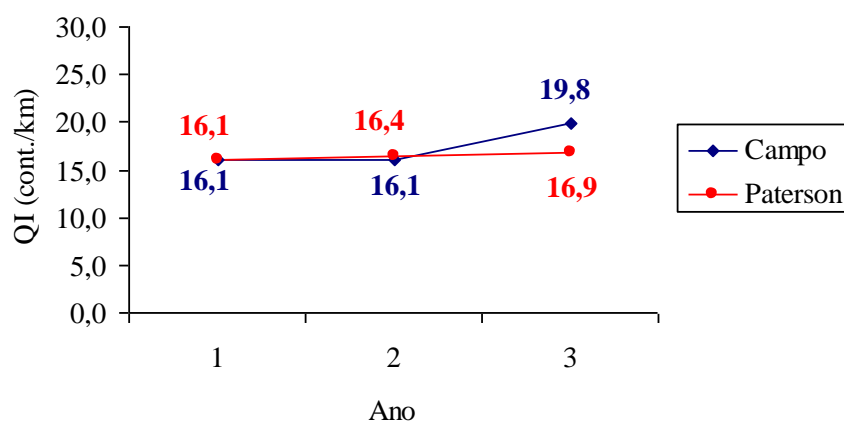
Figura 42 – Evolução irregularidade, escala real e Paterson, 1987 – Trecho 04
