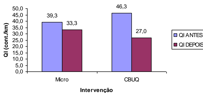
Figura 165 – QI após intervenção, Trecho 06
