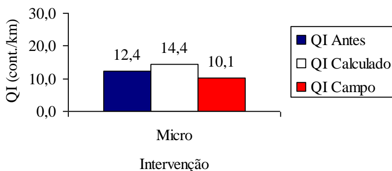
Figura 53 – QI antes da restauração, QI calculado e calculado e QI médio - Trecho 02
