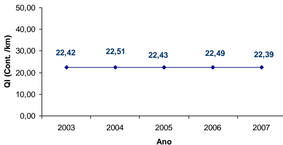
Figura 148 – Evolução QI, “Queiroz A”, Trecho 03
