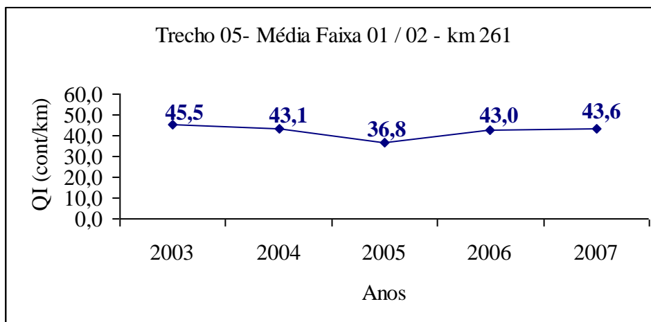
Figura 121 - Trecho 05, Média Faixa 01 / 02 - Km 261
