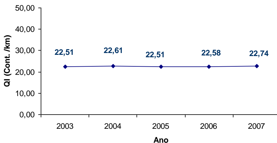
Figura 154 – Evolução QI, “Queiroz A”, Trecho 05
