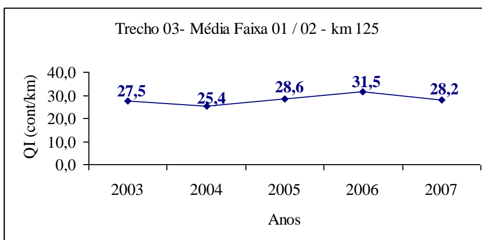
Figura 103 - Trecho 03, Média Faixa 01 / 02 - Km 125
