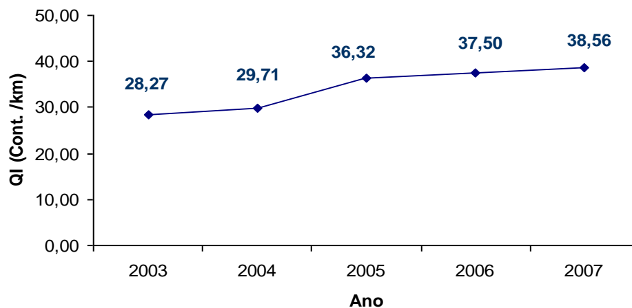
Figura 147 – Evolução QI, “Queiroz C”, Trecho 02
