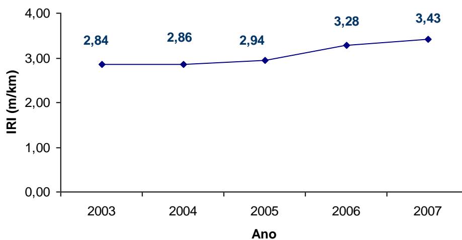
Figura 140 – Evolução IRI, Trecho 05
