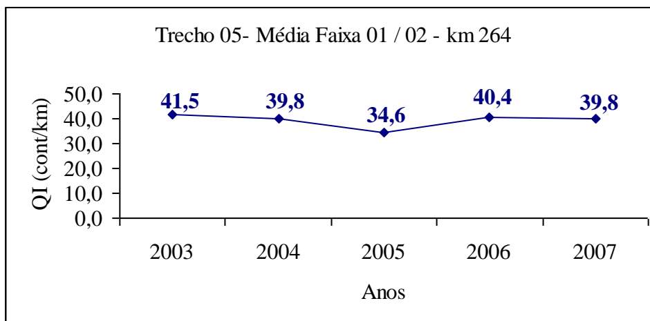
Figura 124 - Trecho 05, Média Faixa 01 / 02 - Km 264
