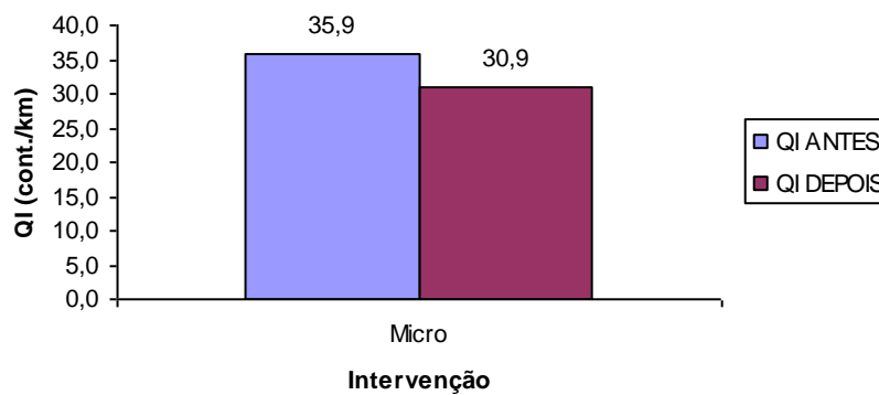
Figura 164 – QI após intervenção, Trecho 05
