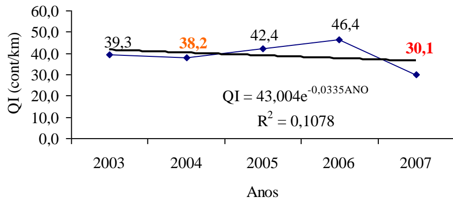
Figura 26 – Evolução Irregularidade longitudinal – Trecho 06
