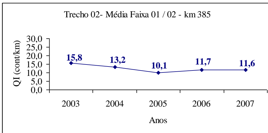
Figura 94 - Trecho 02, Média Faixa 01 / 02 - Km 385
