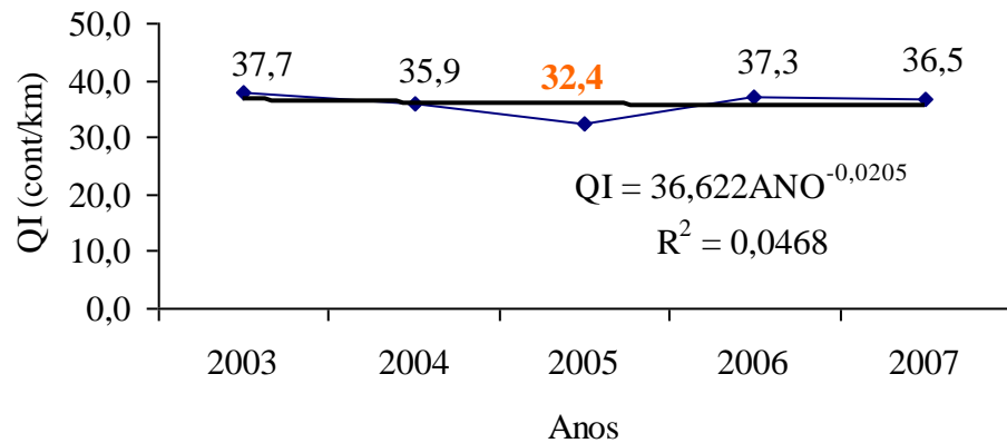
Figura 25 – Evolução Irregularidade longitudinal – Trecho 05
