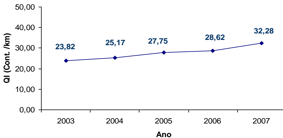
Figura 156 – Evolução QI, “Queiroz C”, Trecho 05
