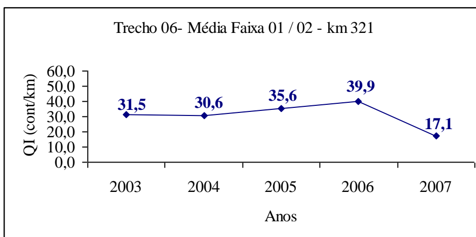
Figura 134 - Trecho 06, Média Faixa 01 / 02 - Km 321
