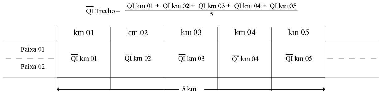
Figura 20 – Média de QI por km e trecho
