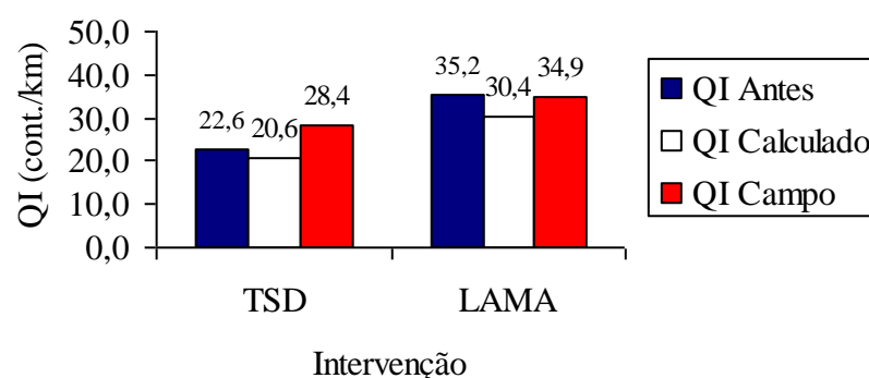
Figura 52 – QI antes da restauração, QI calculado e calculado e QI médio - Trecho 01
