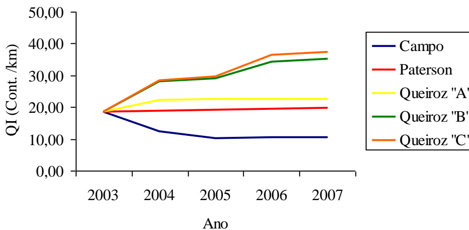
Figura 45 – Evolução da irregularidade longitudinal prevista e real – Trecho 02
