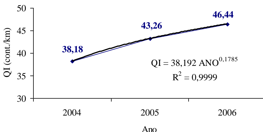
Figura 39 - Evolução de Micro Concreto Asfáltico, Trecho 06
