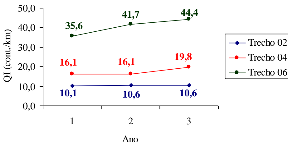
Figura 40 – Evolução Irregularidade a campo em pavimentos sem intervenções
