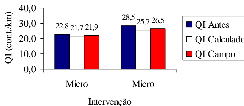
Figura 50 – QI antes da restauração, QI calculado e calculado e QI médio - Trecho 03
