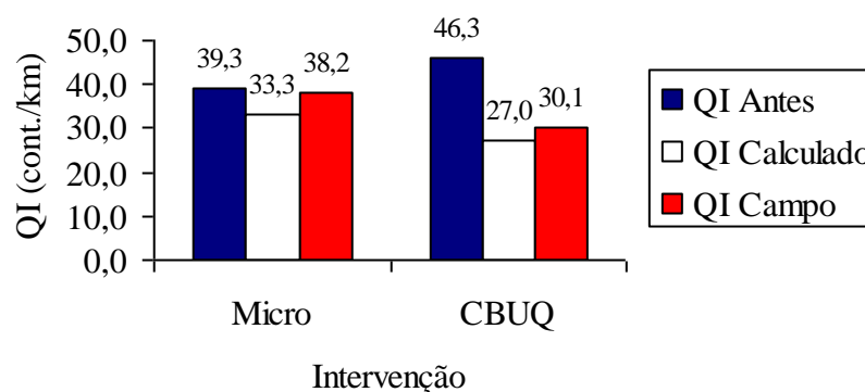
Figura 55 – QI antes da restauração, QI calculado e calculado e QI médio - Trecho 06
