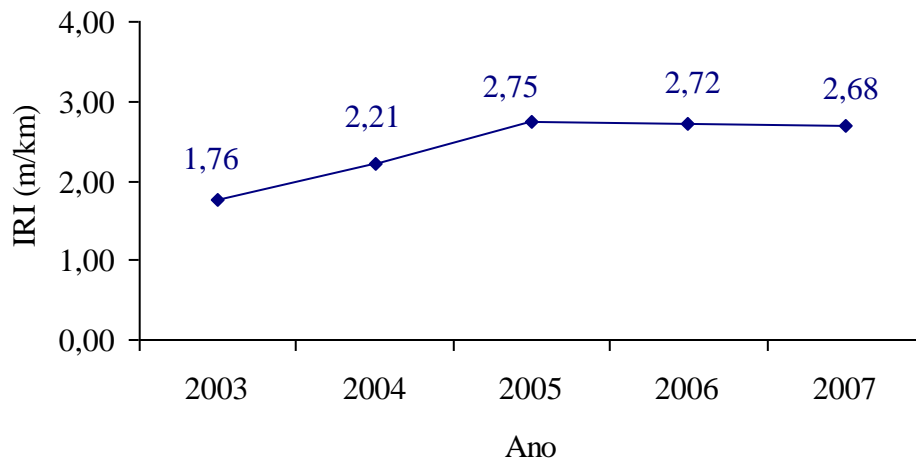
Figura 27 – Evolução Irregularidade longitudinal – Trecho 01
