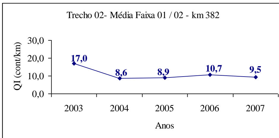
Figura 91 - Trecho 02, Média Faixa 01 / 02 - Km 382
