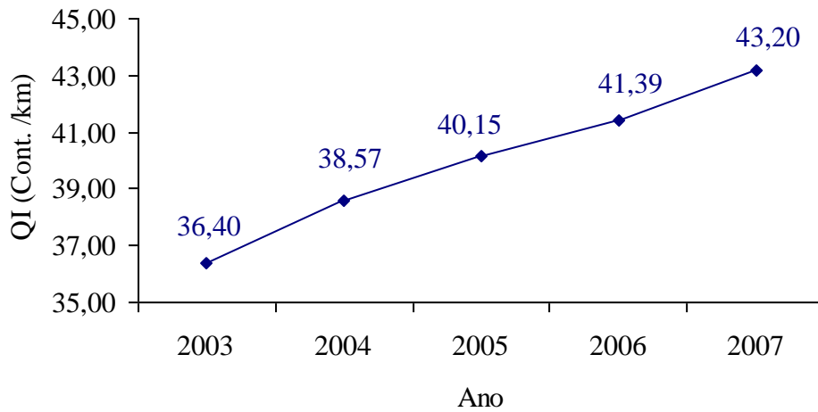
Figura 29 – Evolução da irregularidade longitudinal “Queiroz B”– Trecho 01
