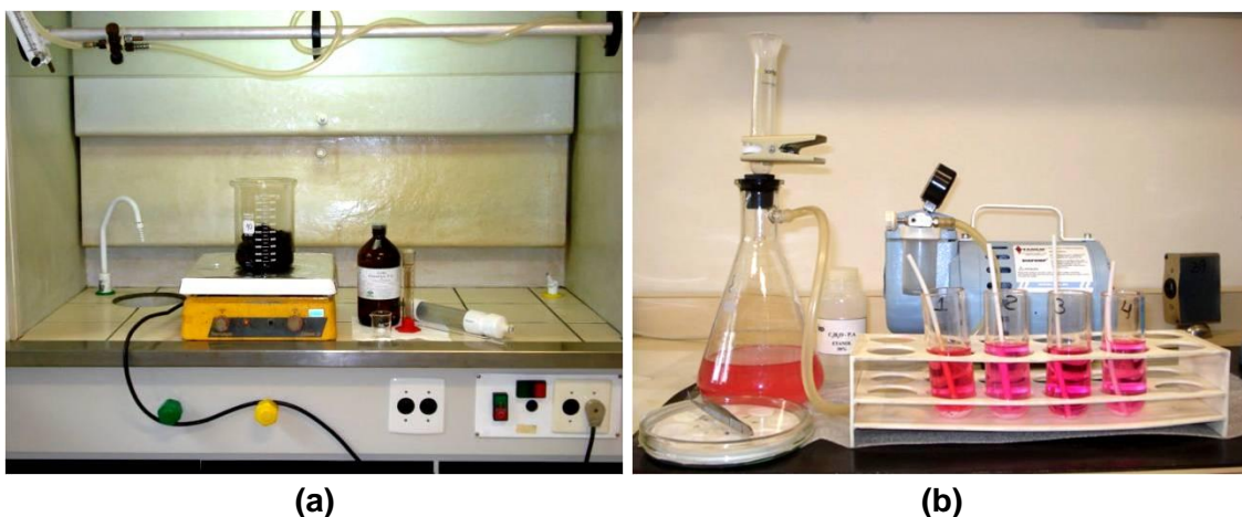
Figura 21 – (a) Lixiviação da fibra de manganês e (b) Sistema de filtração
