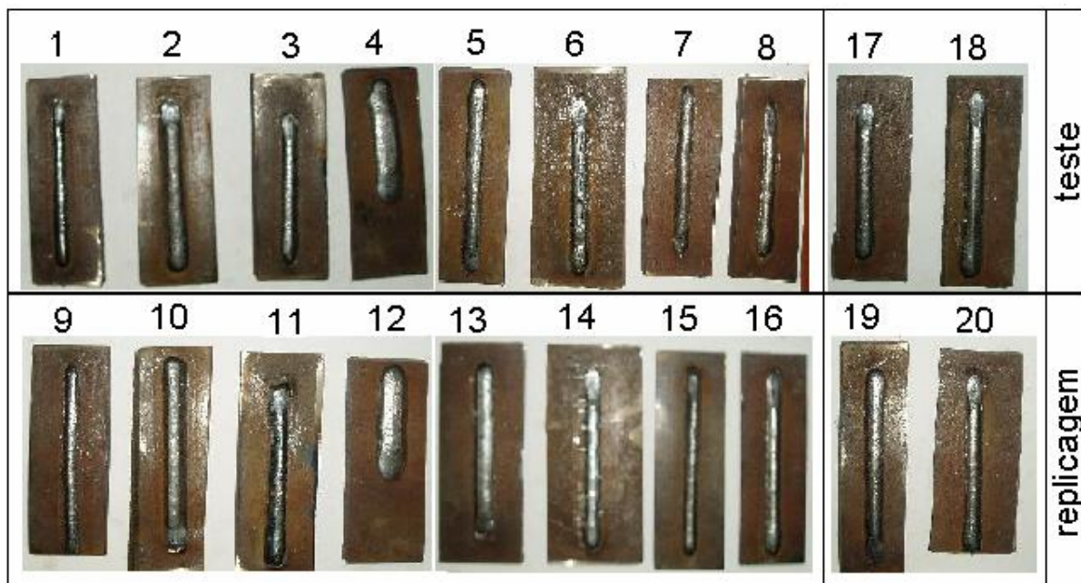
Figura 4.2 – Cordões de solda obtidos no fatorial fracionário.
