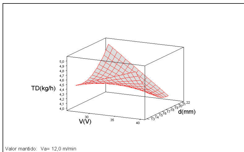
Figura 4.10 – Superfície de resposta V \cdot d para a taxa de deposição.
