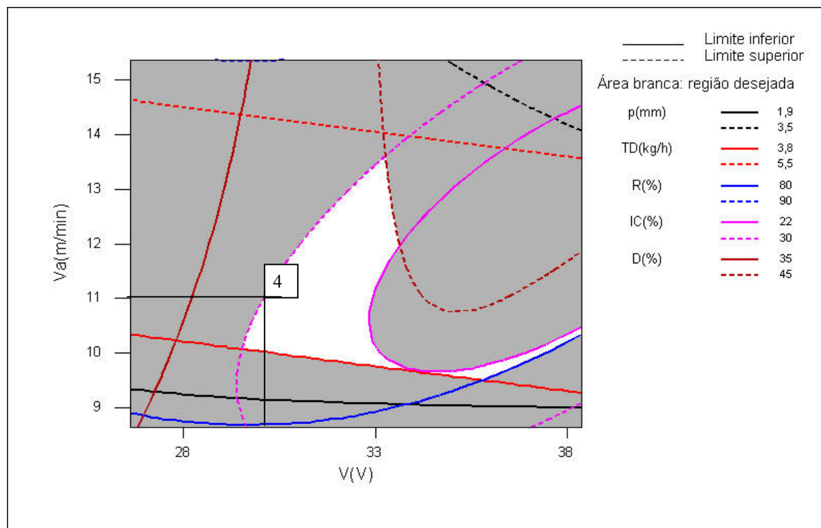
Figura 4.22 – Linhas de contorno das respostas combinadas, d=13,4\text{mm} .
