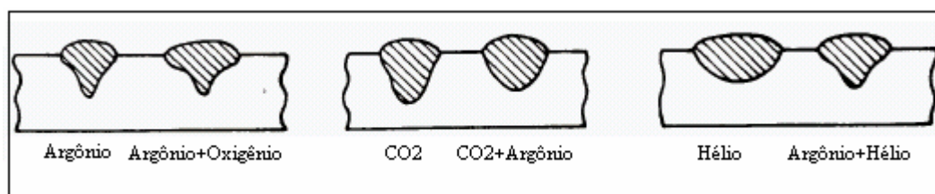
Figura 2.2 – Efeito do gás de proteção no perfil do cordão de solda com eletrodo tubular, Bracarense (2000).
