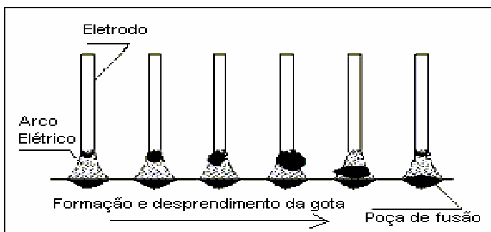
Figura 2.7 - Transferência globular.
