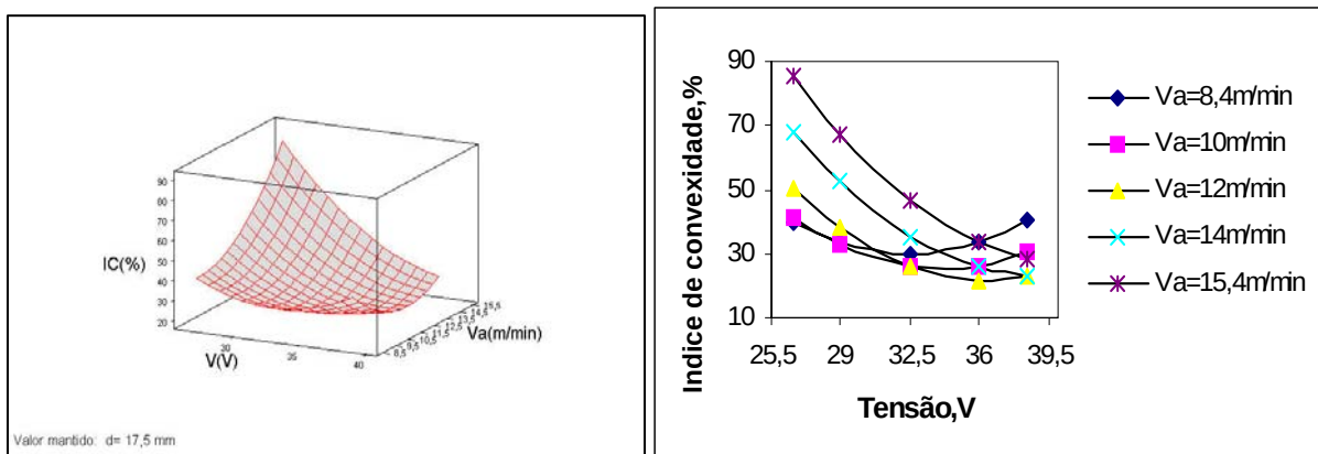
Figura 4.16 – Efeito da interação V*Va no índice de convexidade, d=17,5\text{mm} .
