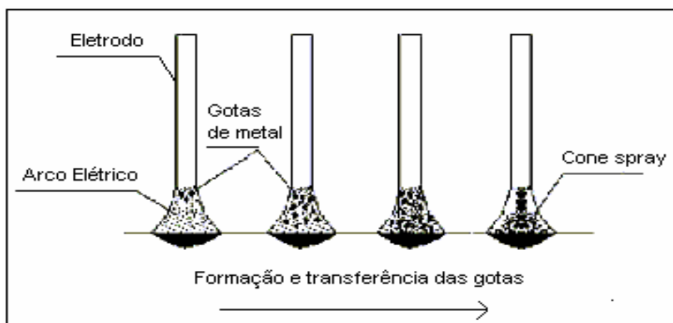
Figura 2.8 - Transferência por spray.
