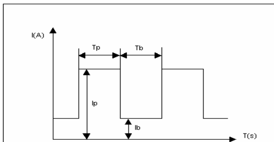
Figura 2.9 - Esquema de uma onda pulsada.
