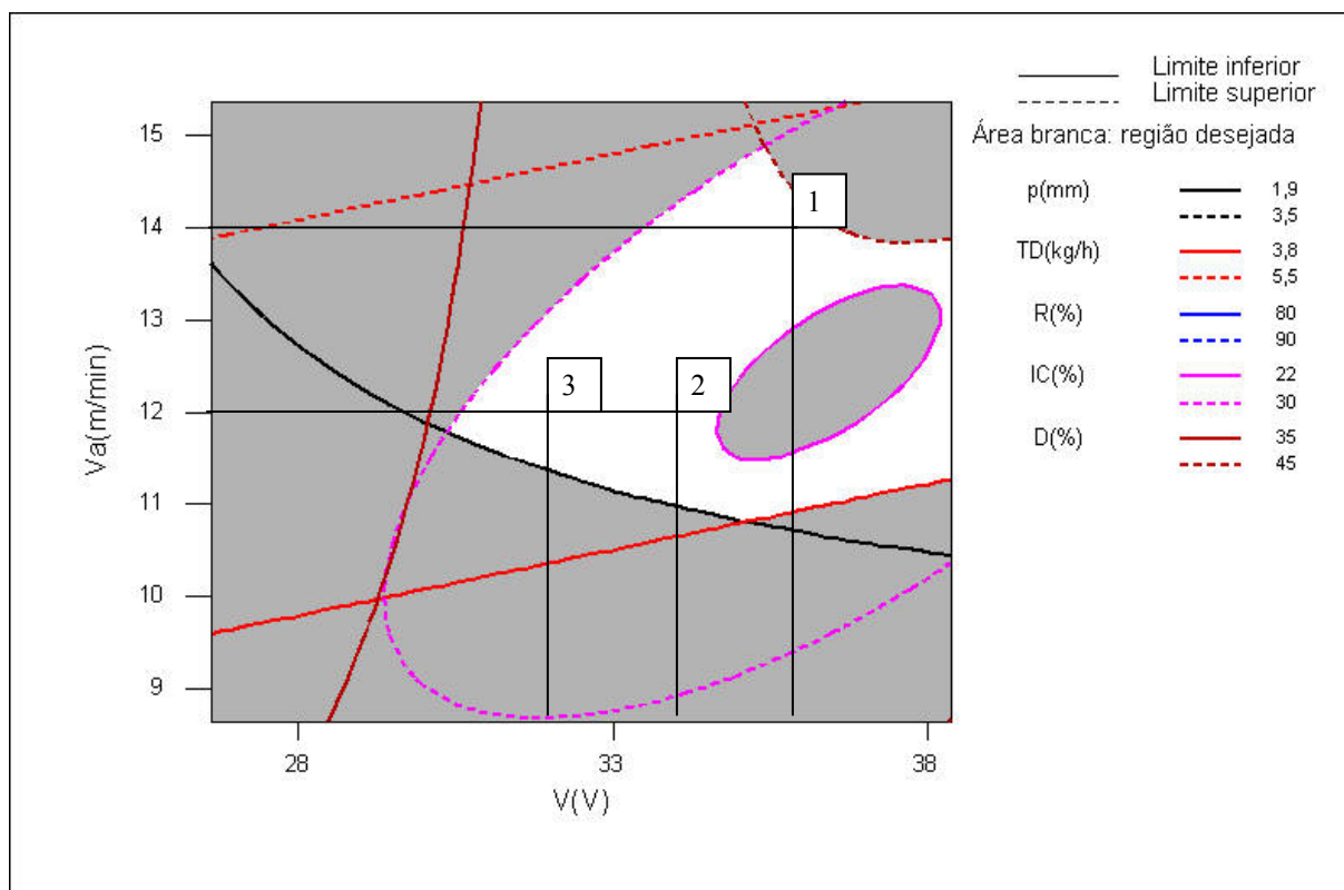
Figura 4.23 – Linhas de contorno das respostas combinadas, d=20\text{mm} .
