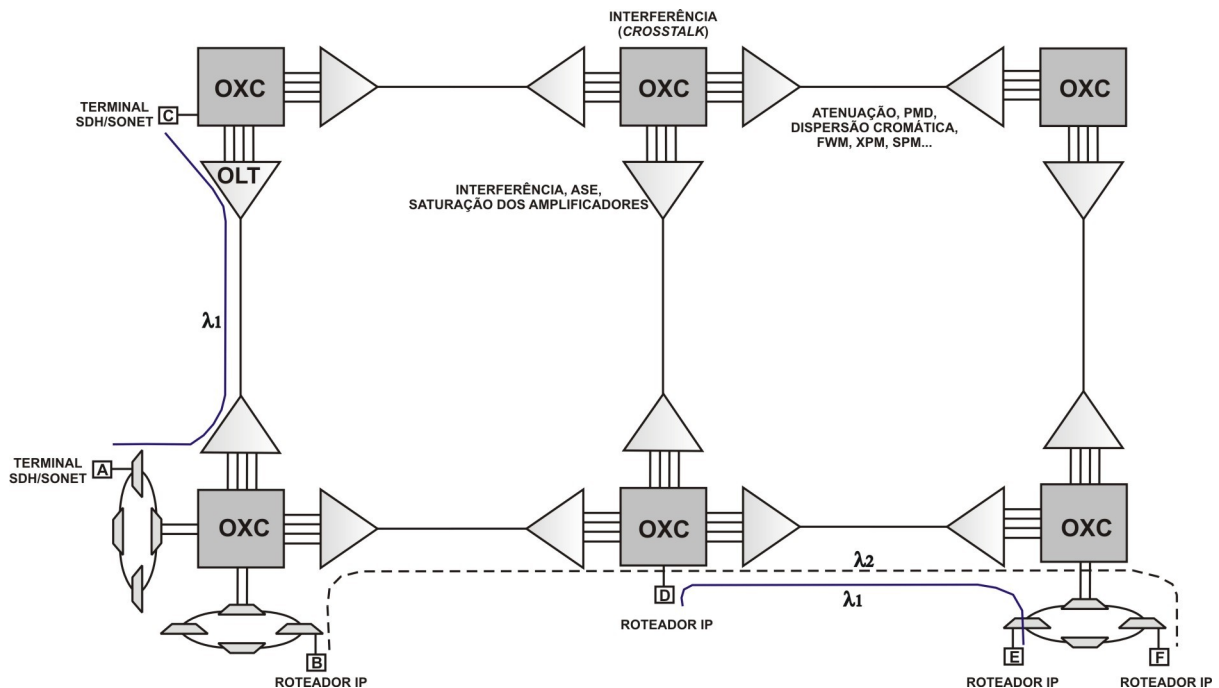
Figura 2.2: Interligação de clientes IP e SONET/SDH com a rede óptica com uma representação física dos elementos da rede óptica.
