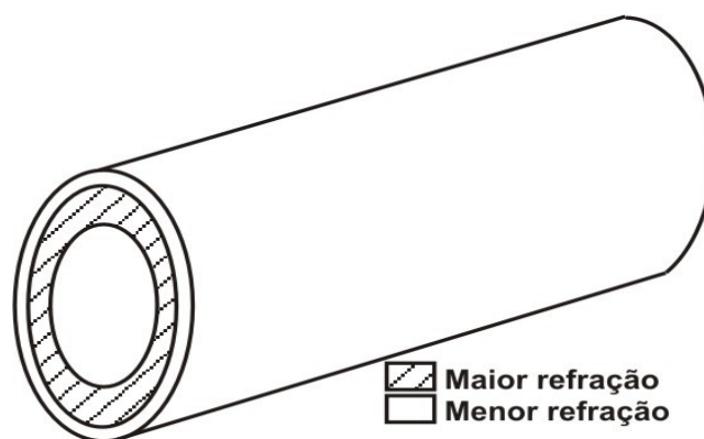
Figura 2.6: Fibra de grande área efetiva.
