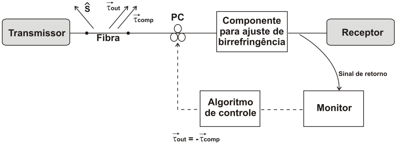
Figura 3.6: Anulação de PMD.
