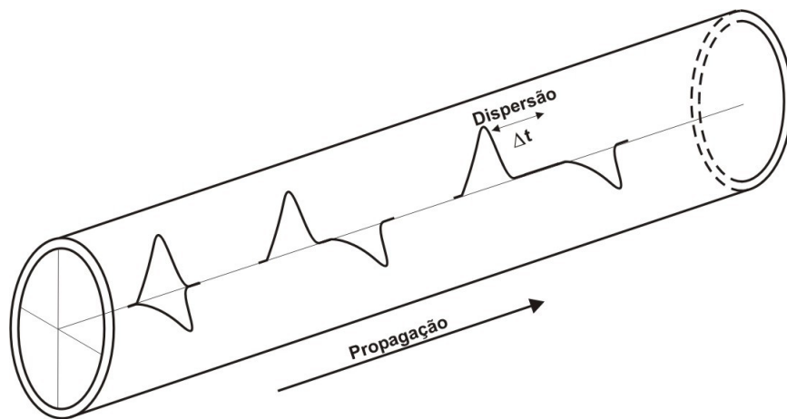
Figura 3.1: Dispersão de Modo de Polarização.
