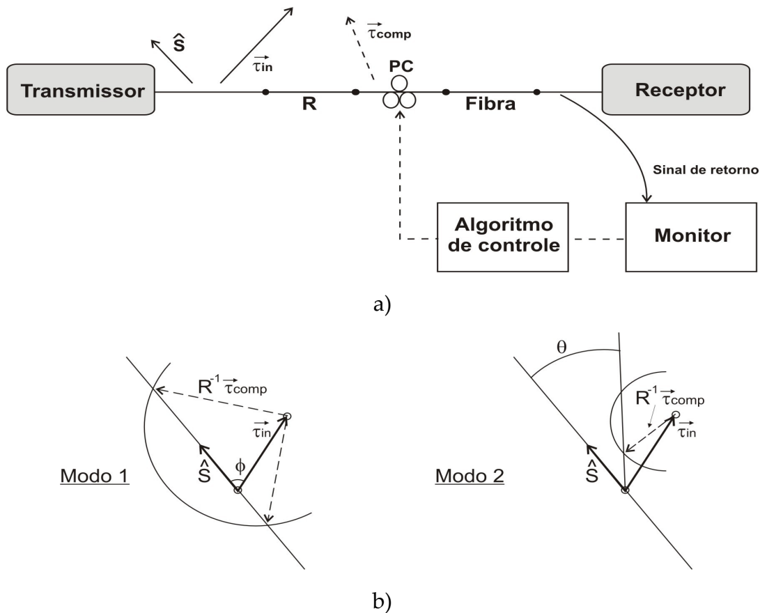
Figura 3.7: a) Atenuação de PMD utilizando um compensador DGD fixo. (b) Os dois modos de operação são indicados por diagramas vetor PMD.
