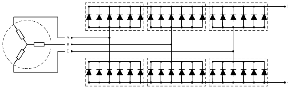
Figura 2.6 - Diagrama Esquemático do Conjuntos de Diodos.
