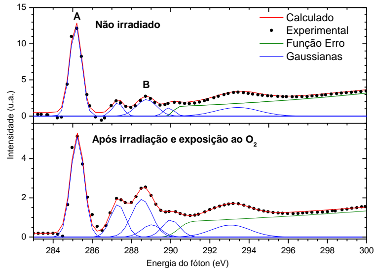
Figura 49: Espectros NEXAFS de Carbono 1s de filmes de PS sem e com tratamento por radiação SR por 15 min a 293,5 eV. Os espectros NEXAFS na borda K foram obtidos após recuperar as condições de UAV.
