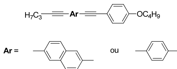
Figura 11: Estrutura molecular dos cristais líquidos derivados dos fenil ou naftiltolanos. 13
