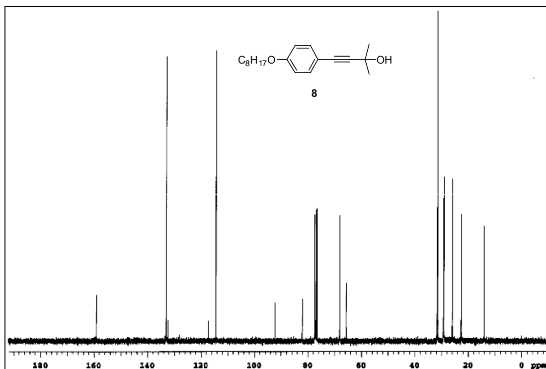
Espectro de RMN ^{13}\text{C} do alcinol 8 ( \text{CDCl}_3 , 75,5 MHz).
