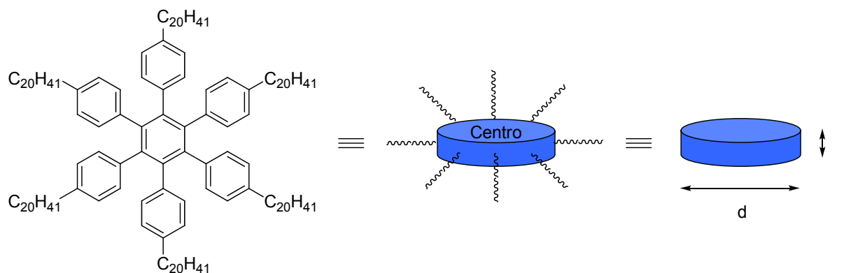
Figura 7: Exemplo de uma molécula de cristal líquido discótico 8 e representações ilustrativas, onde d \gg l .
