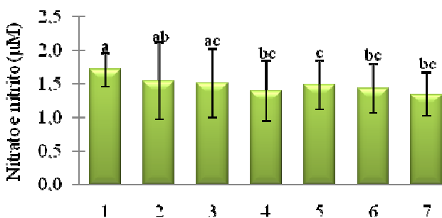
Figura 9 – Concentração ( \mu\text{M} ) de nitrato e nitrito ( \text{NO}_3^- + \text{NO}_2^- ) em amostras de água coletada em 7 pontos da região de Sambaqui no grupo intermediário. Valores apresentados em médias sazonais. As barras verticais apresentam o intervalo de confiança, considerando p < 0,05 . As letras representam as diferenças significativas de acordo com teste a posteriori de Tukey.
