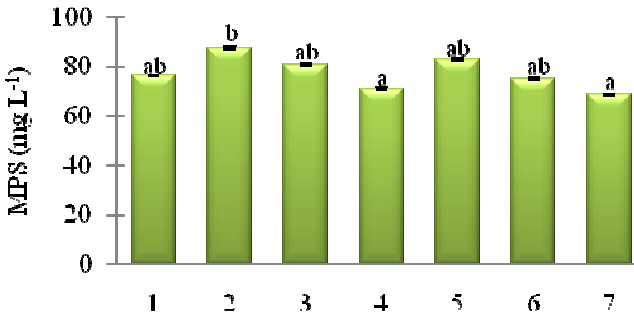
Figura 7 – Quantidade ( \text{mg L}^{-1} ) de material particulado em suspensão (MPS) em amostras de água coletada em 7 pontos da região de Sambaqui no grupo do verão. Valores apresentados em médias sazonais. As barras verticais apresentam o intervalo de confiança, considerando p < 0,05 . As letras representam as diferenças significativas de acordo com teste a posteriori de Tukey.
