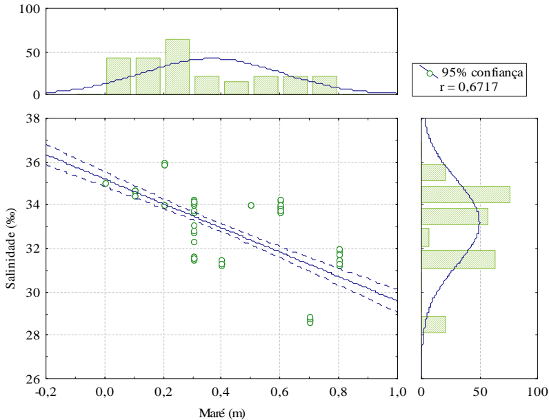
Figura 4 – Correlação da salinidade e maré incluindo as 12 coletas, evidenciando a alta relação entre os dois parâmetros.
