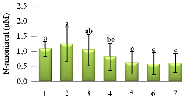
Figura 8 – Concentração ( \mu\text{M} ) de N-amoniacoal ( \text{NH}_4^+ ) em amostras de água coletada em 7 pontos da região de Sambaqui no grupo intermediário. Valores apresentados em médias sazonais. As barras verticais apresentam o intervalo de confiança, considerando p < 0,05 . As letras representam as diferenças significativas de acordo com teste a posteriori de Tukey.
