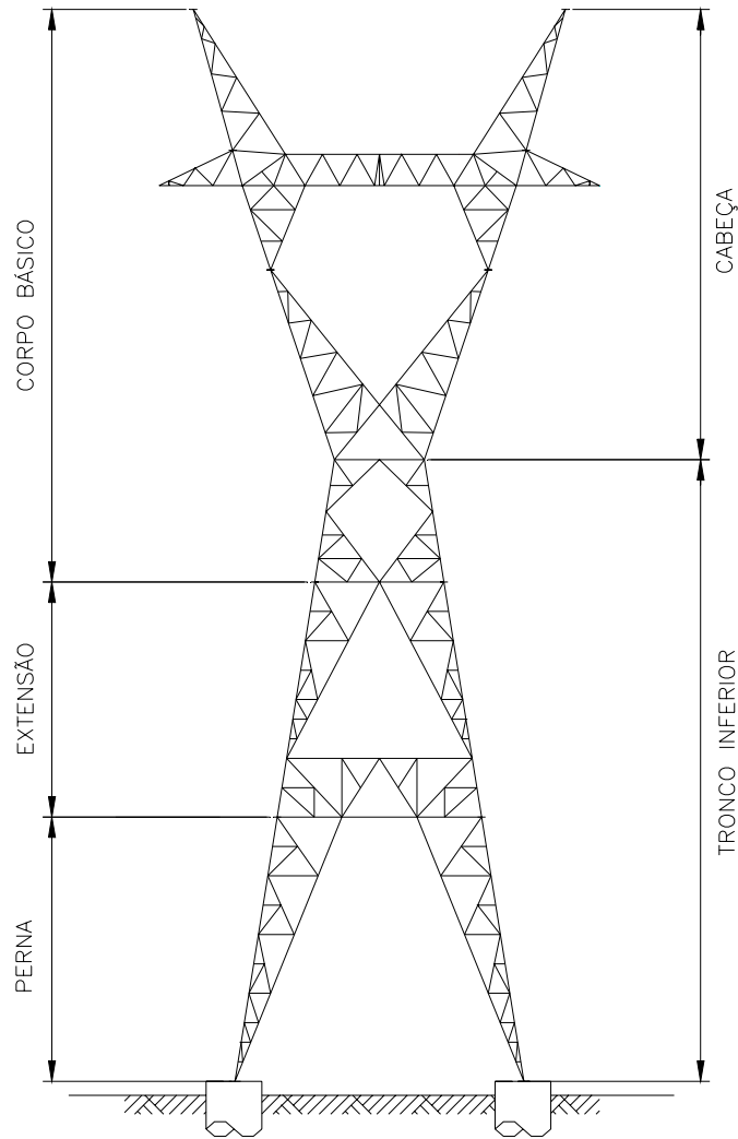
FIGURA 3.1 – Silhueta de Torre Autoportante de LT
