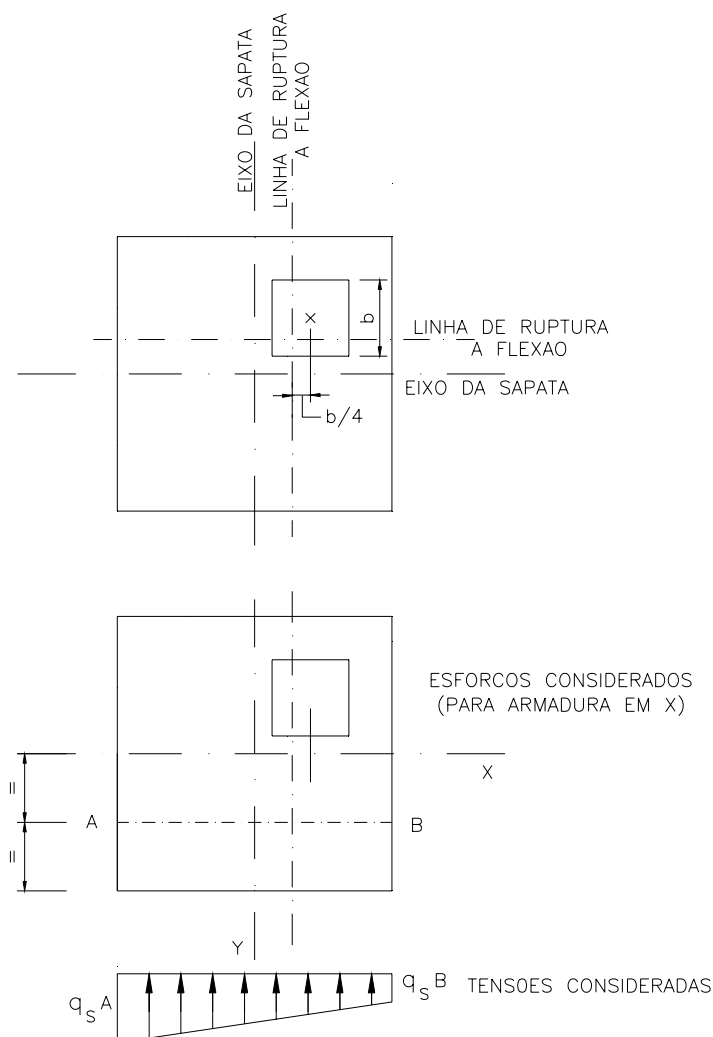
FIGURA 7.18 – Seções de Referência para o Cálculo de Momentos nas Bases
