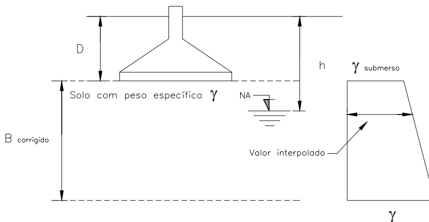
FIGURA 6.8 – Consideração do N.A. sob as Fundações
