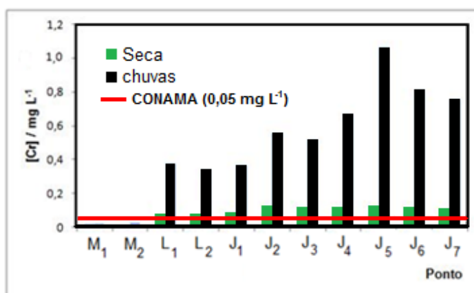
Figura 20: Resultados dos valores de concentração de cromo total, para amostras de água subterrânea coletadas nas minas do Córrego da Paixão. M: Montante; L: Local; J: Jusante. CONAMA: valor de referência.
