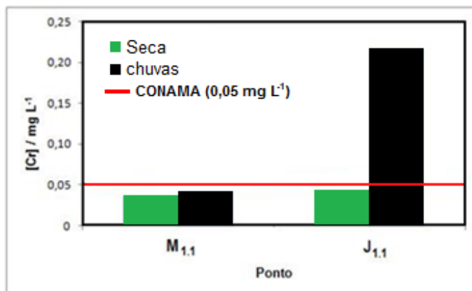
Figura 21: Resultados dos valores de concentração de cromo total, para amostras de água subterrânea coletadas nas minas do Ribeirão da Dobrada. M: Montante; J: Jusante. CONAMA: valor de referência.
