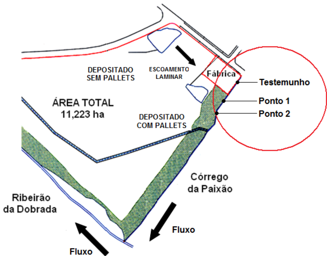
Figura 8 – Esquema da área de estudo ilustrando os pontos de coleta das três amostras de solo na margem direita do Córrego da Paixão.
