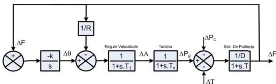
Figura 7.26 – Diagrama de blocos para o caso 6
