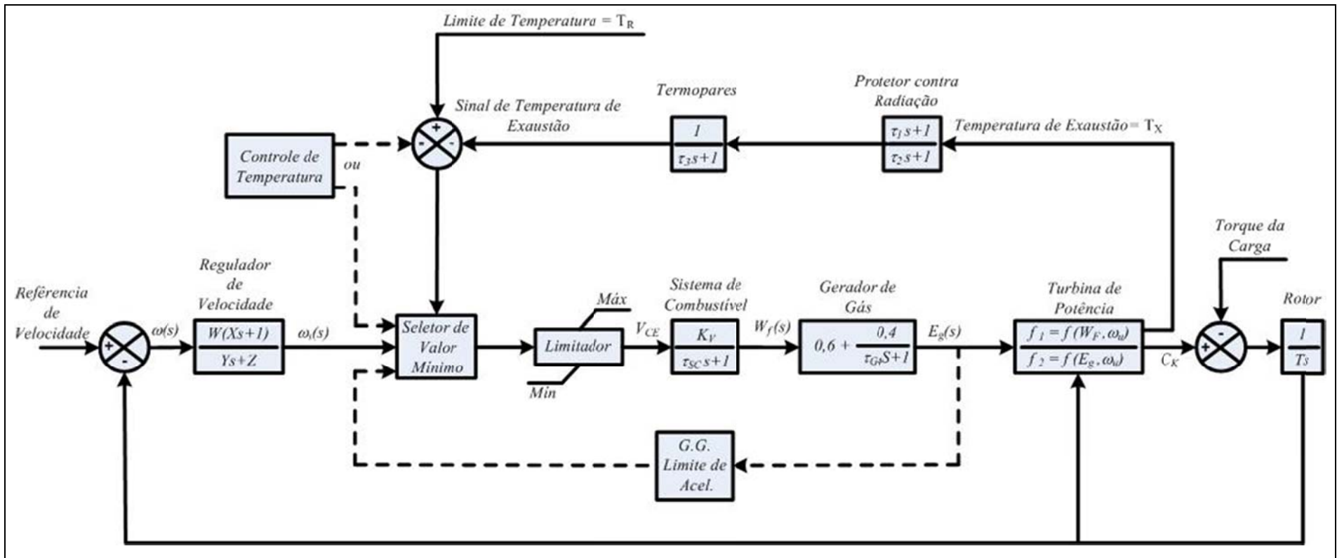
Figura 4.11 – Diagrama de blocos para uma turbina aeroderivativa avançada com dois spools
