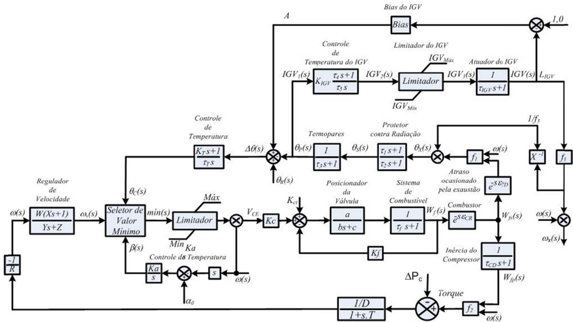
Figura 4.17 – Diagrama de blocos de uma área de controle com turbinas a gás Heavy-Duty
