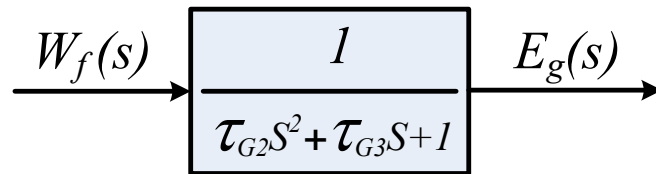
Figura 3.32 – Diagrama de bloco do gerador de gás turbinas Aeroderivativas tradicionais com dois Spools
