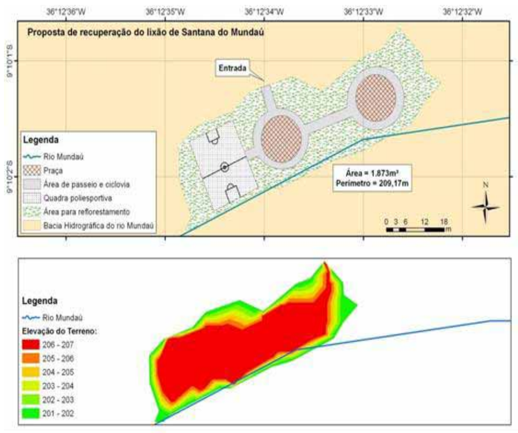
Figura 95 – Modelo Numérico do terreno - MNT do lixão de Santana do Mundaú.
