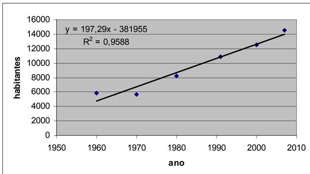
Figura 67 - Curva de crescimento populacional de São José da Laje
