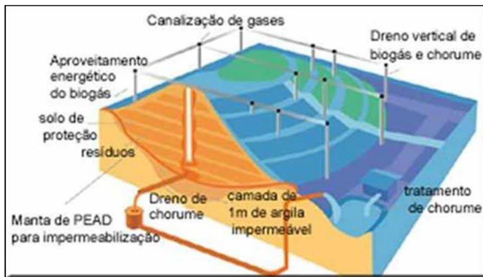
Figura 3- Esquema de canalização de gases e chorume Fonte: Adaptado de Felipetto, 2007.
