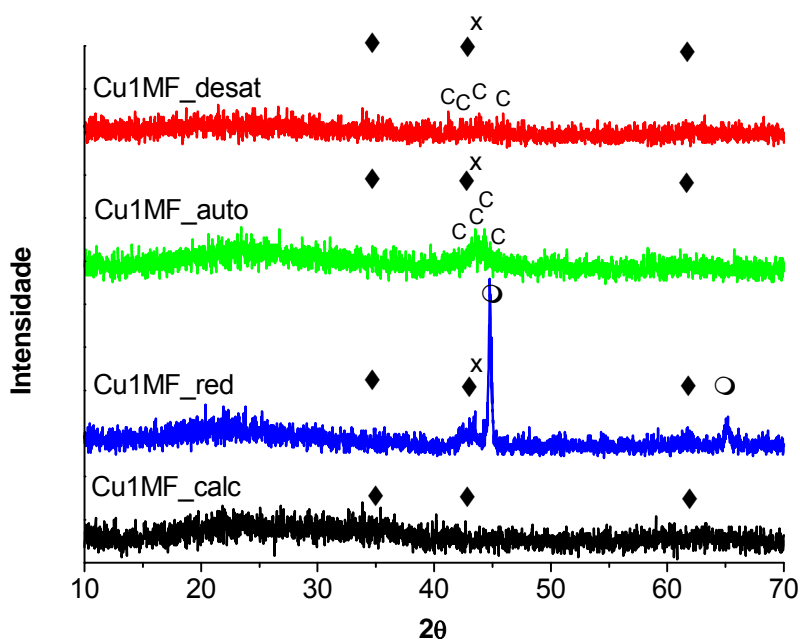
Figura 4.26: Difratogramas de raios-X (XRD) da amostra Cu1MF calcinada, ativada e desativada. As fases cristalinas identificadas são: \blacklozenge , \text{MgFe}_2\text{O}_4 e \text{MgO} ; * , \text{Fe}_2\text{O}_3 ; \circ , \text{Fe}^0 ; \times , \text{Cu}^0 ; C, \text{Fe}_x\text{C} .
