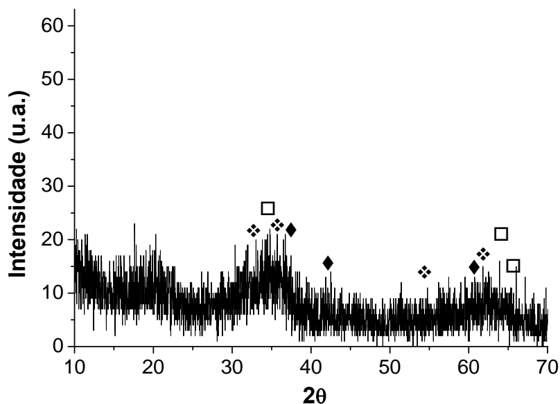
Figura C.2: Difratogramas de raios-X (XRD) de amostra \text{Fe}_{80}\text{Al}_{20} calcinada. As fases cristalinas identificadas são: ◆, \text{FeO} ; □, \text{FeAlO}_3 ; ⋄, \text{Fe}_2\text{O}_3 (AZAMBUJA e PEREZ-LOPEZ, 2007).
