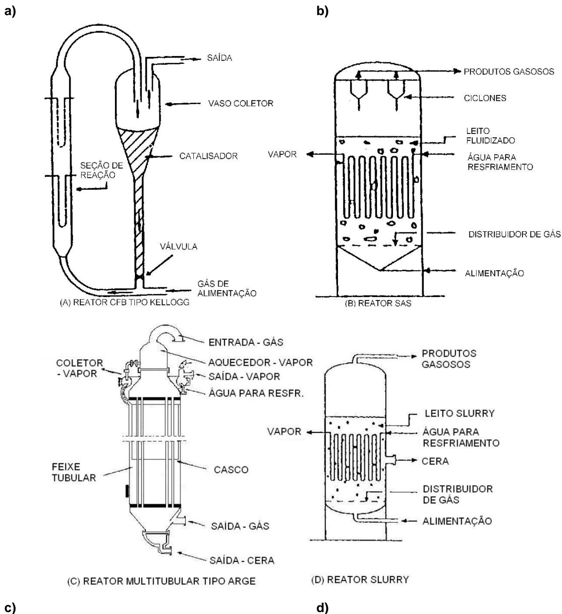
Figura 2.2: Reatores utilizados para FTS: (a) reator CFB tipo Kellogg; (b) reator de leito fluidizado borbulhante SAS; (c) reator multitubular tipo Arge e (d) reator slurry (DRY, 2002; ESPINOZA et al. , 1999).
