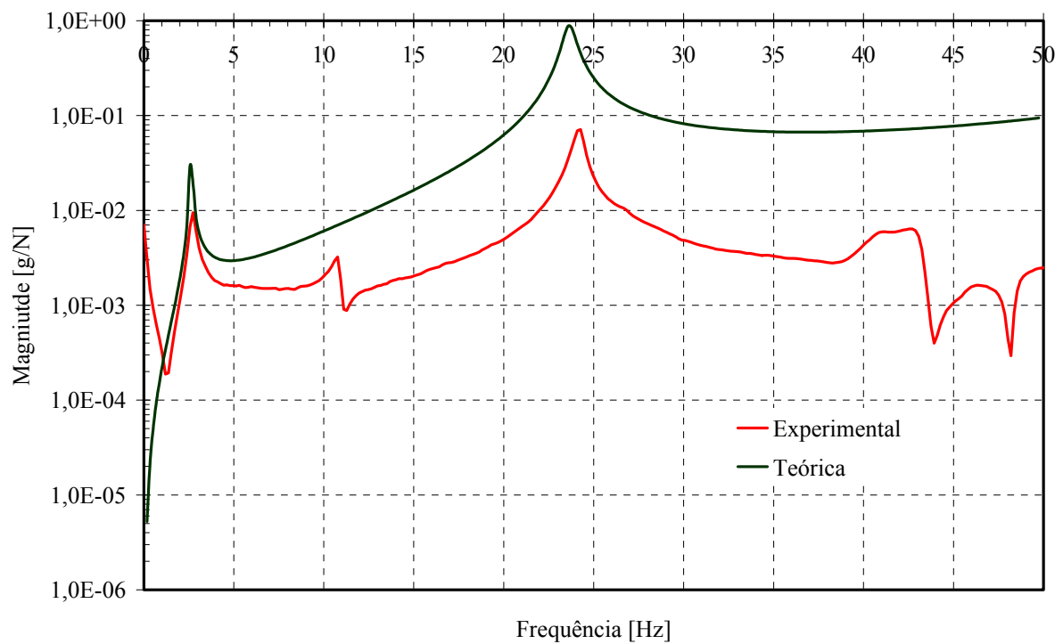
Figura 14.4: FRF de transferência H_{13}
