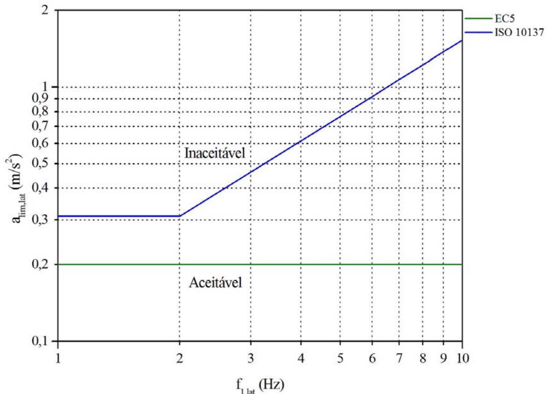
Figura 5.12: Comparativo entre critérios normativos para aceitação de vibração na direção transversal horizontal
