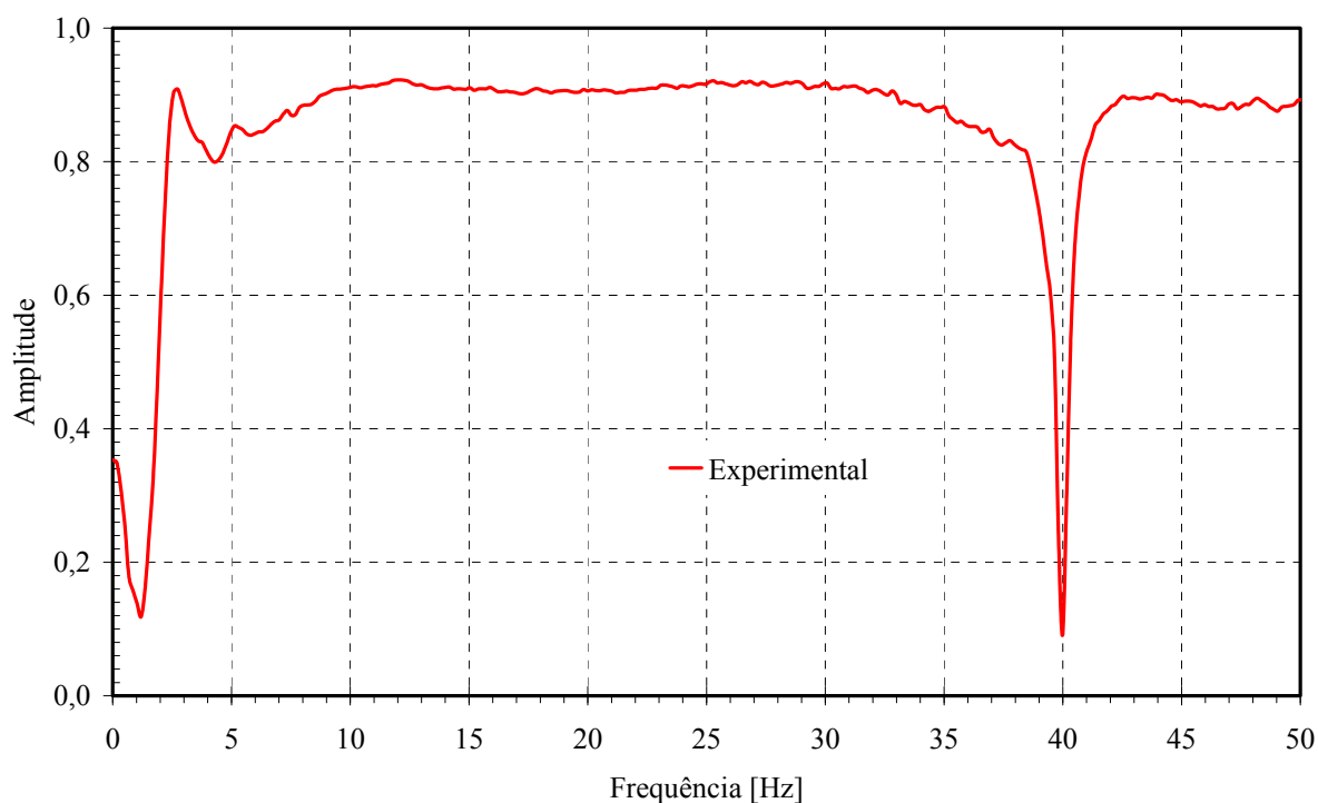
Figura 14.24: Coerência da FRF de transferência H_{25}
