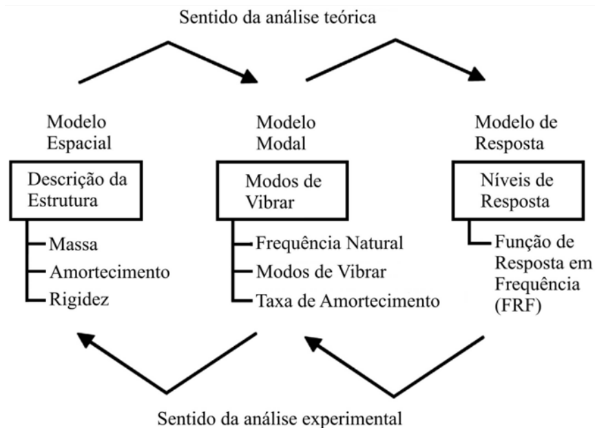
Figura 3.3: Inter-relações entre os modelos da análise modal
