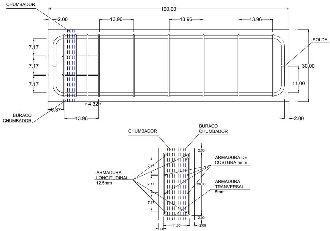
Figura 3.6 – Distribuição da armadura na viga para os modelos 1, 2 e 3.
