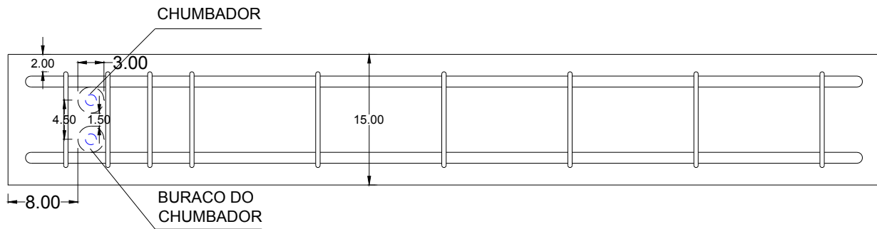
Figura 3.9 – Posicionamento dos chumbadores.
