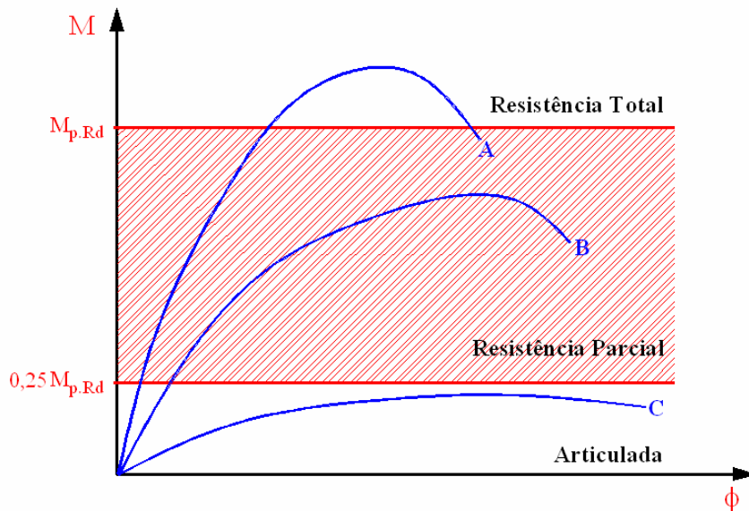
Figura 2.5 - Classificação das ligações pela resistência.
