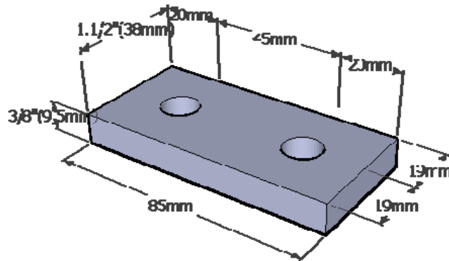
Figura A.7 - Ancorador
