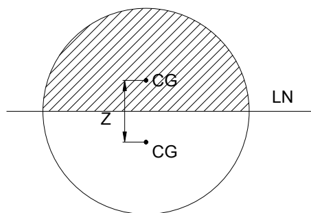
Figura B.2 - Seção do chumbador.
