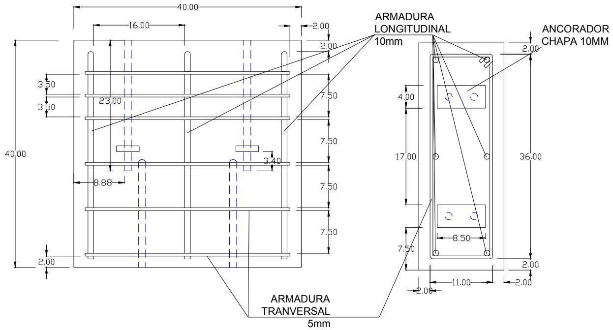
Figura 3.4 – Detalhamento da armadura do pilar para os modelos 1, 2 e 3.
