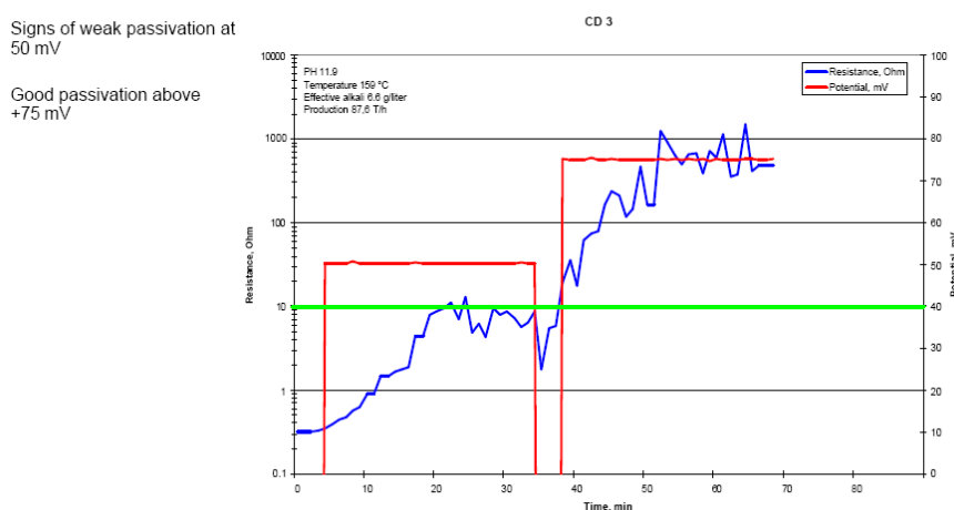
Figura 5.13: resultados CER do digestor 2, abril 2007 (Savcor, 2007).
