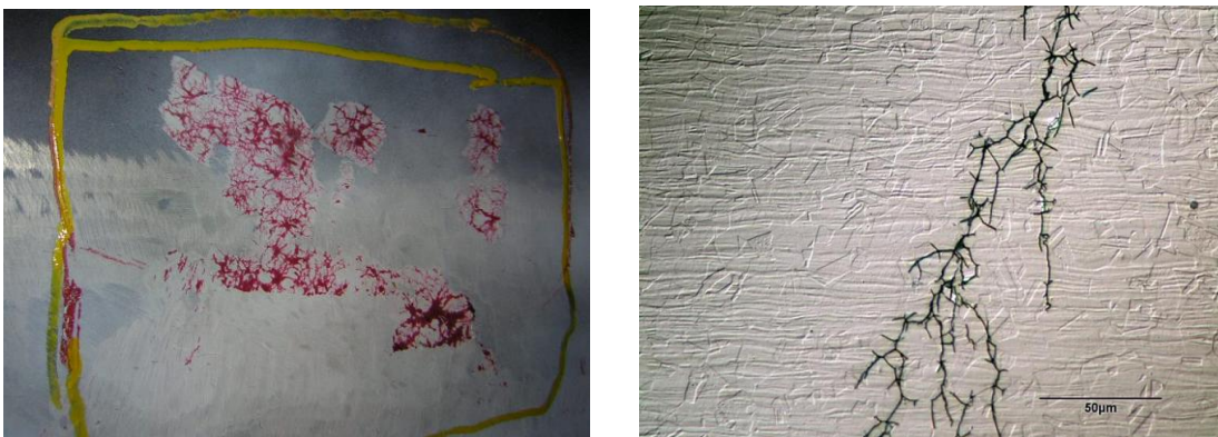
Figura 3.10: aspecto macrográfico (a) e micrográfico (b) da corrosão sob tensão fraturante (SCC) (CENIBRA, 2004; Wensley, 2006).
