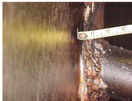
Figura 5.3: área com corrosão uniforme. Notar a perda de material junto à solda (CENIBRA, 2002).
