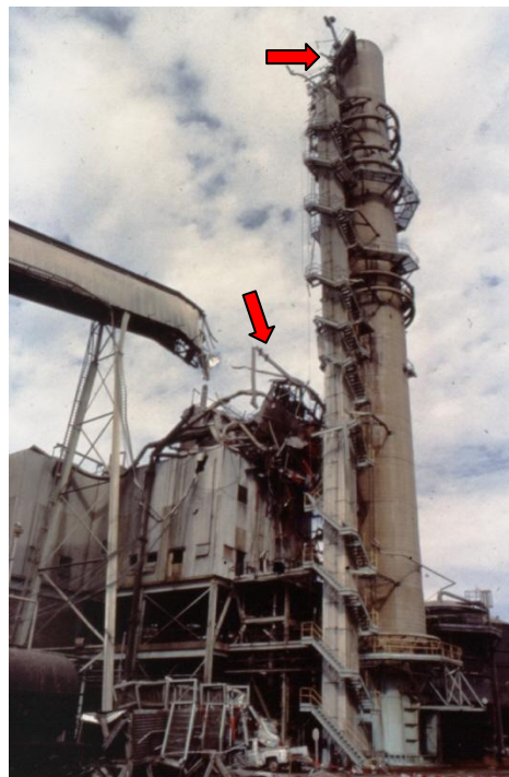
Figura 1.1: falha catastrófica de digestor contínuo em Pine Hill, Alabama, 1980, devido à corrosão sob tensão fraturante, SCC (Wensley, 2008).
