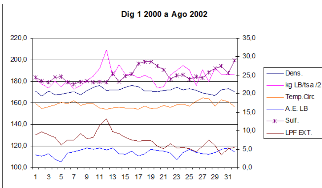
Figura 5.9: dados de processo do digestor 1, 2000 a 2002 (CENIBRA, 2003).
