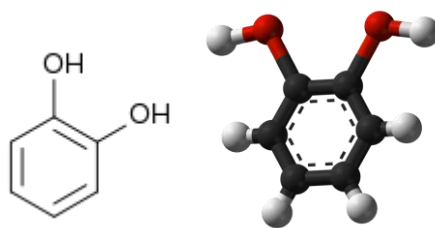
Figura 3.16: estrutura do catecol (Hazlewood, 2006)
