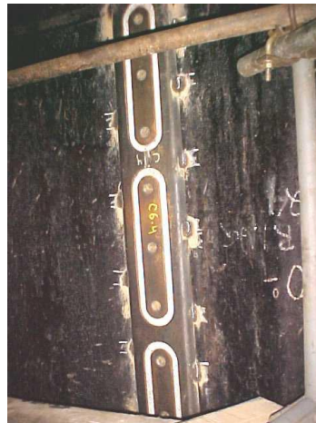
Figura 3.21: detalhe de um catodo fixado por solda intermitente à superfície interna do digestor (CENIBRA, 2006).
