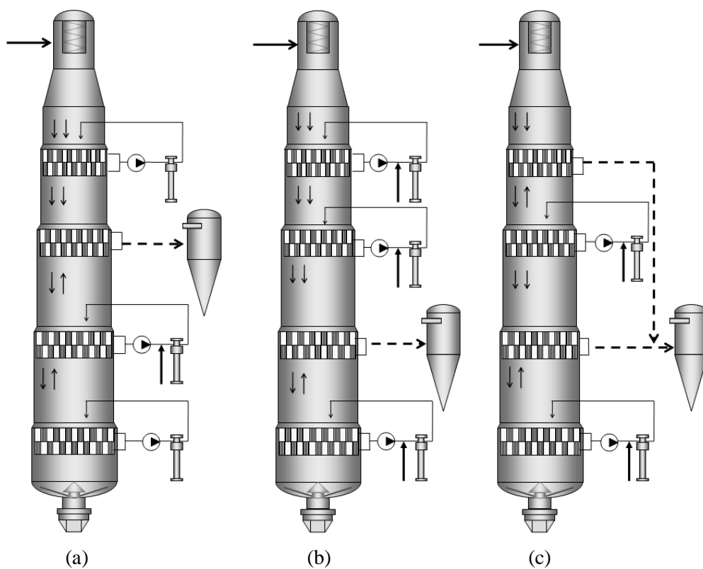
Figura 3.2: esquemas de alguns tipos de cozimento modificado: (a) Cozimento Contínuo Modificado (MCC), (b) Cozimento Contínuo Modificado Estendido (EMCC) / Cozimento Isotérmico (ITC™) e (c) LoSolids™ (adaptado de Klarin-Henricson, 2004).
