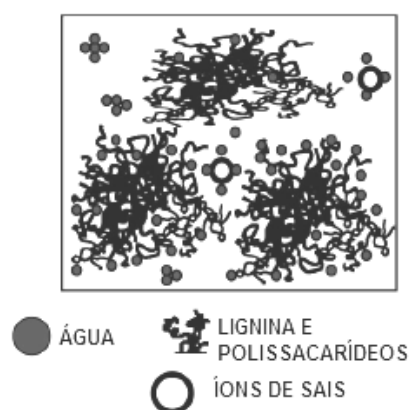
Figura 3.14: estrutura do licor preto (Cardoso et al. , 2008)
