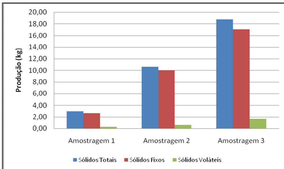
Figura 47 – Produção de sólidos totais, fixos e voláteis, ao longo das três amostragens realizadas na fossa de sedimentos.
