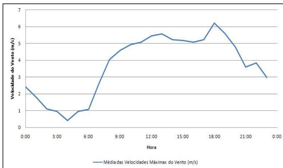
Figura 54 – Velocidades máximas horárias do vento entre os dias 30/11/2007 e 06/12/2007.
