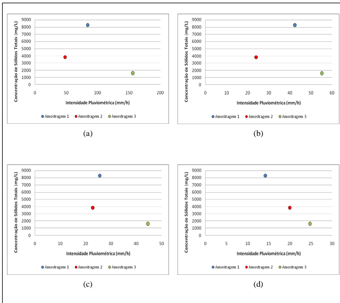
Figura 52 – Relação entre a intensidade pluviométrica máxima entre os eventos antecedentes à amostragem e a concentração média de sólidos em suspensão da amostragem: (a) Discretização de 1 minuto; (b) Discretização de 15 minutos; (c) Discretização de 30 minutos; e (d) Discretização de 60 minutos.
