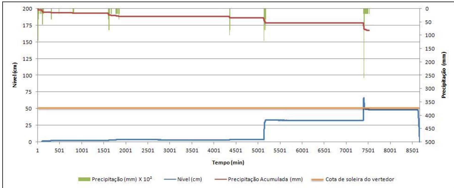
Figura 40 – Registros pluviográficos e linigráficos resultantes dos eventos pluviométricos erosivos antecedentes a Amostragem 3 na microbacia.
