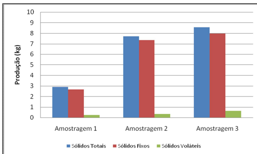
Figura 44 – Produção de sólidos totais, fixos e voláteis, relativa às amostras de fundo, ao longo das três amostragens realizadas na fossa de sedimentos.
