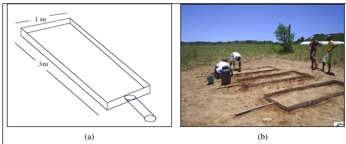
Figura 23 – (a) Esquemática da parcela de erosão instalada na bacia experimental (SANTOS, 2006); e (b) Instalação das parcelas experimentais de erosão.
