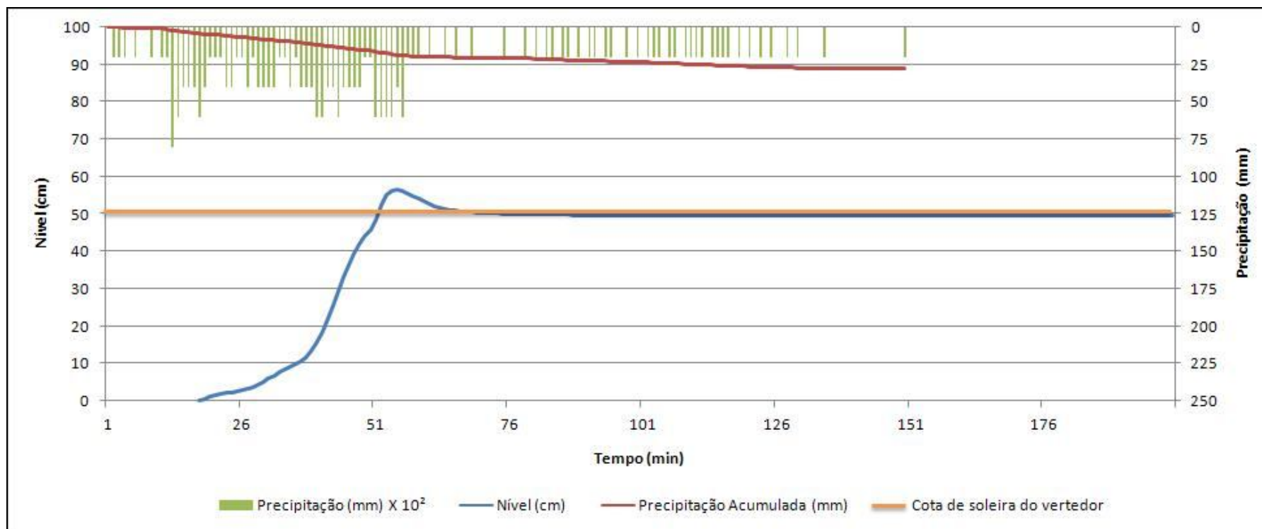
Figura 39 – Registros pluviográficos e linigráficos resultantes do evento pluviométrico erosivo 13 na microbacia.
