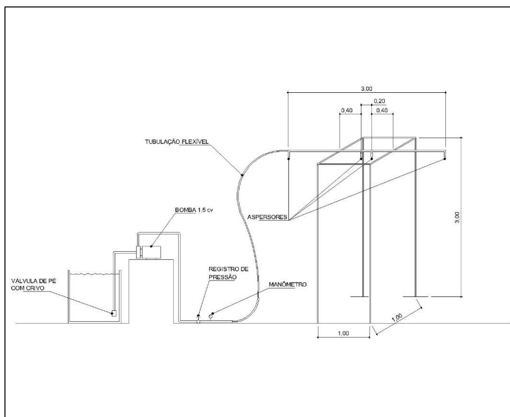
Figura 25 – Esquematização do simulador de chuvas operado nas parcelas experimentais de erosão.
