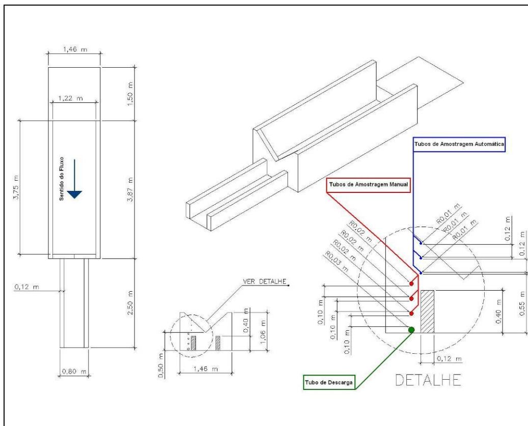
Figura 16 – Esquemática da fossa de sedimentos construída na microbacia.
