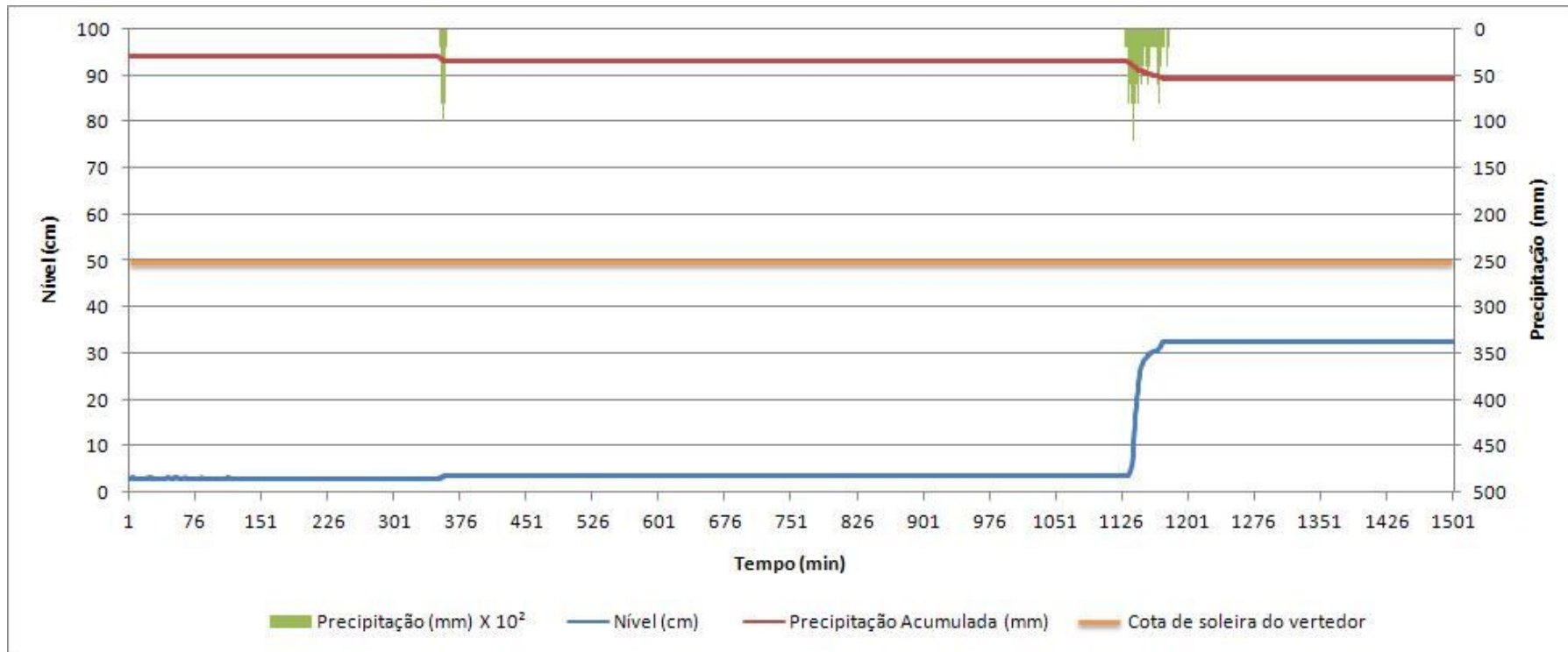
Figura 42 – Registros pluviográficos e linigráficos resultantes do evento pluviométrico erosivo 16 na microbacia.
