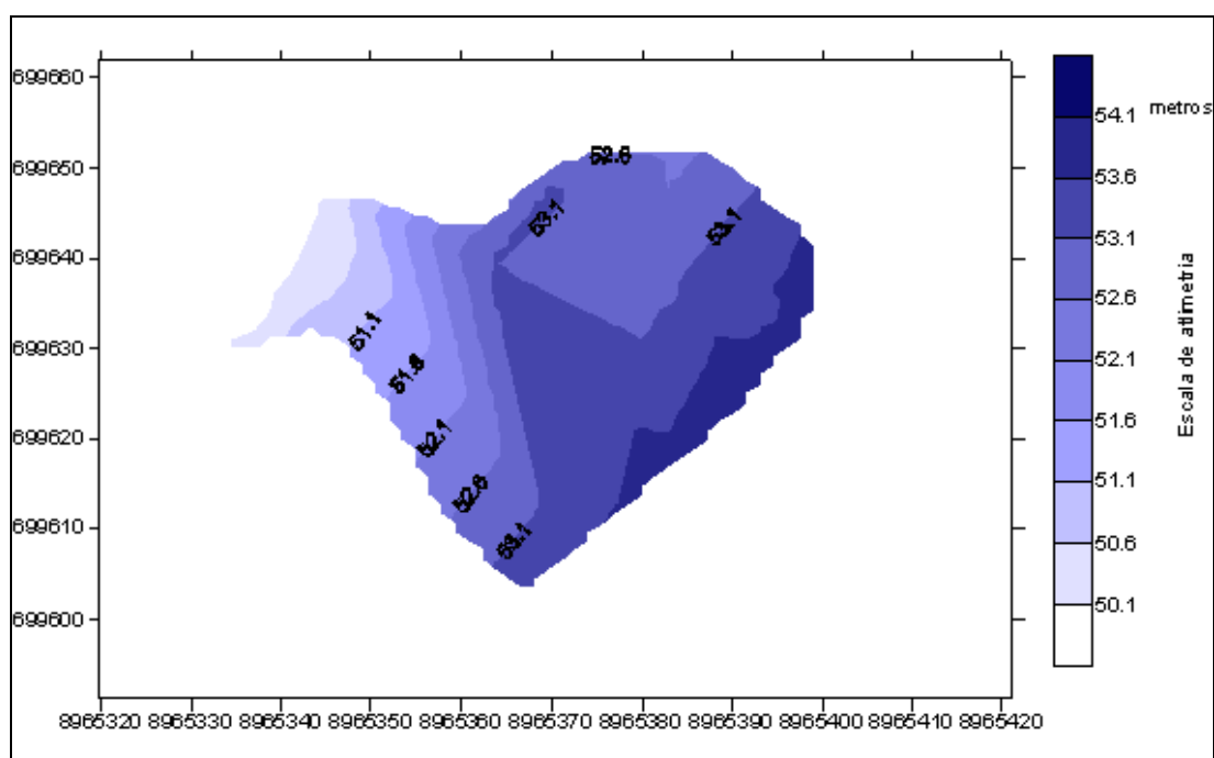
Figura 14 – Isolinhas de nível da microbacia.
