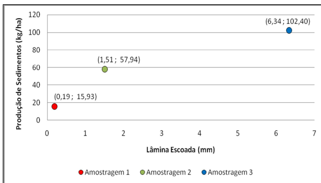
Figura 48 – Relação entre a produção de sedimentos e a lâmina total escoada antecedente à cada amostragem realizada na fossa de sedimentos da microbacia.
