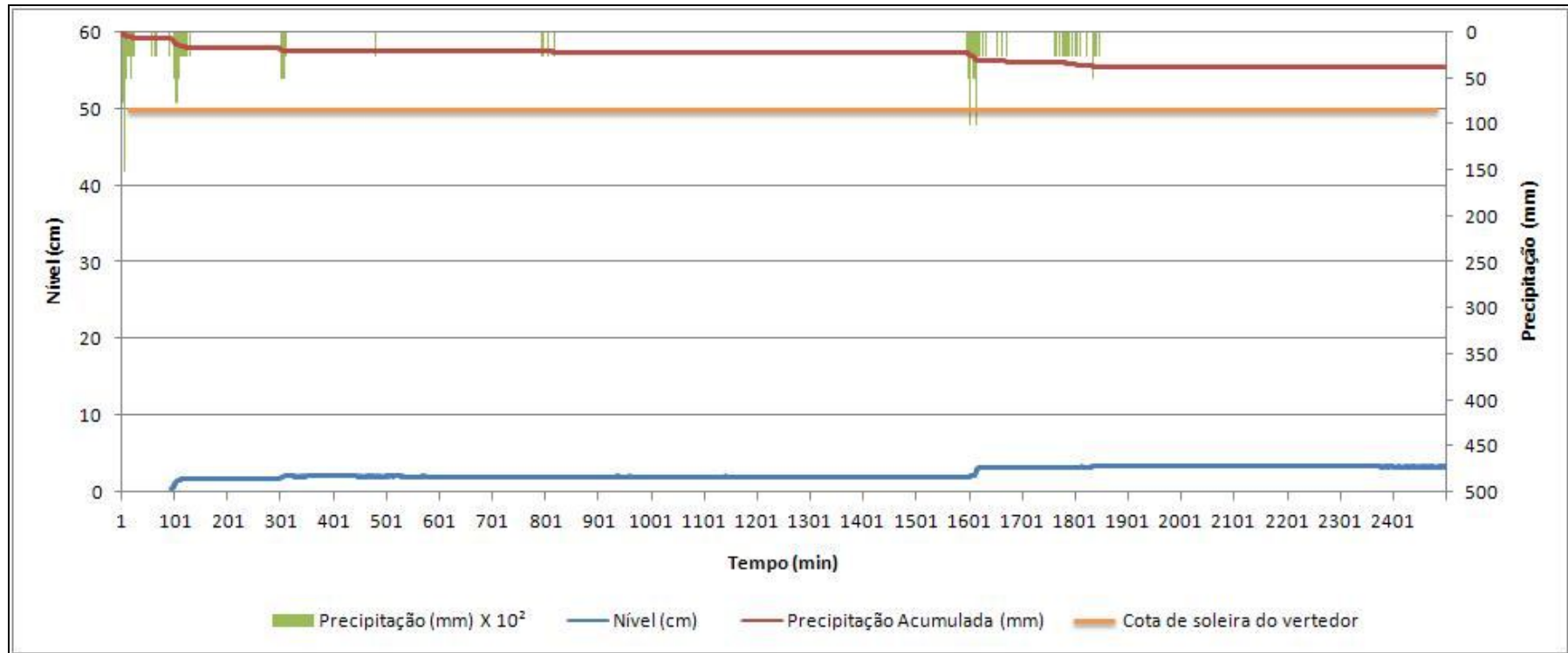
Figura 41 – Registros pluviográficos e linigráficos resultantes dos eventos pluviométricos erosivos 14 e 15 na microbacia.
