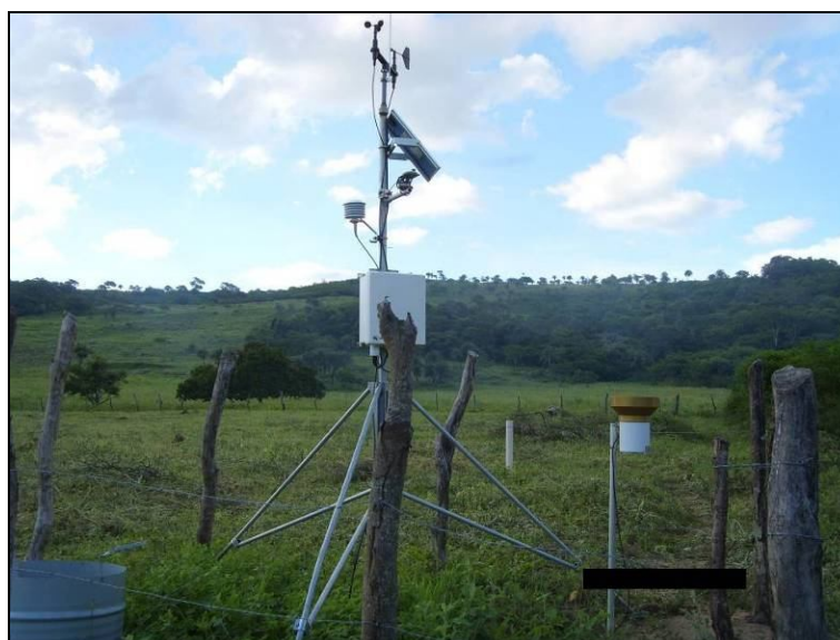
Figura 11 – Estação meteorológica compacta (CAMPBELL SCIENTIFIC) instalada na bacia experimental.
