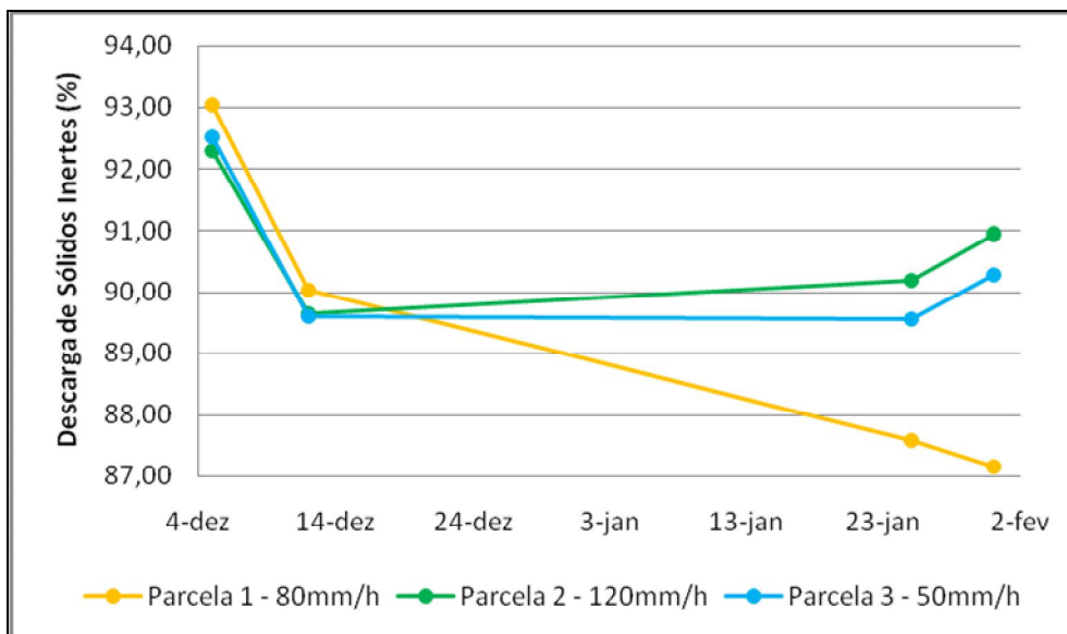
Figura 56 – Fração de sólidos fixos, nas parcelas experimentais de erosão, ao longo das simulações de chuva.
