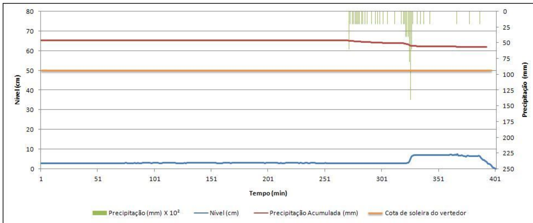
Figura 37 – Registros pluviográficos e linigráficos resultantes do evento pluviométrico erosivo 10 na microbacia.
