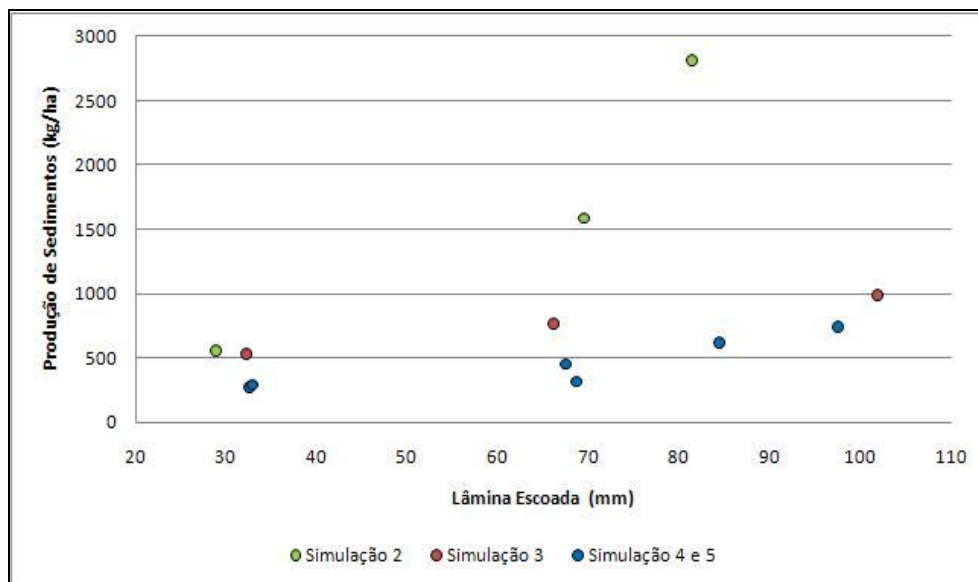
Figura 58 – Relação entre a produção de sedimentos e a lâmina total escoada referente às simulações de chuva nas parcelas experimentais de erosão.
