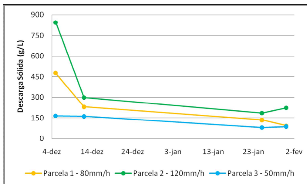
Figura 55 – Descarga média de sólidos totais, nas parcelas experimentais de erosão, ao longo das simulações de chuva.
