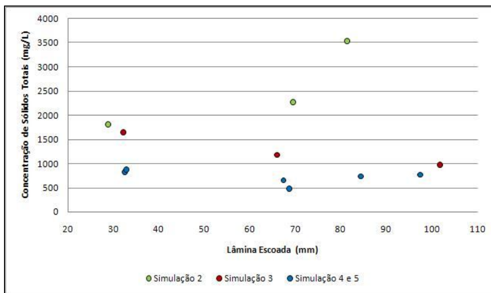
Figura 59 – Relação entre a concentração de sólidos totais e a lâmina total escoada referente às simulações de chuva nas parcelas experimentais de erosão.
