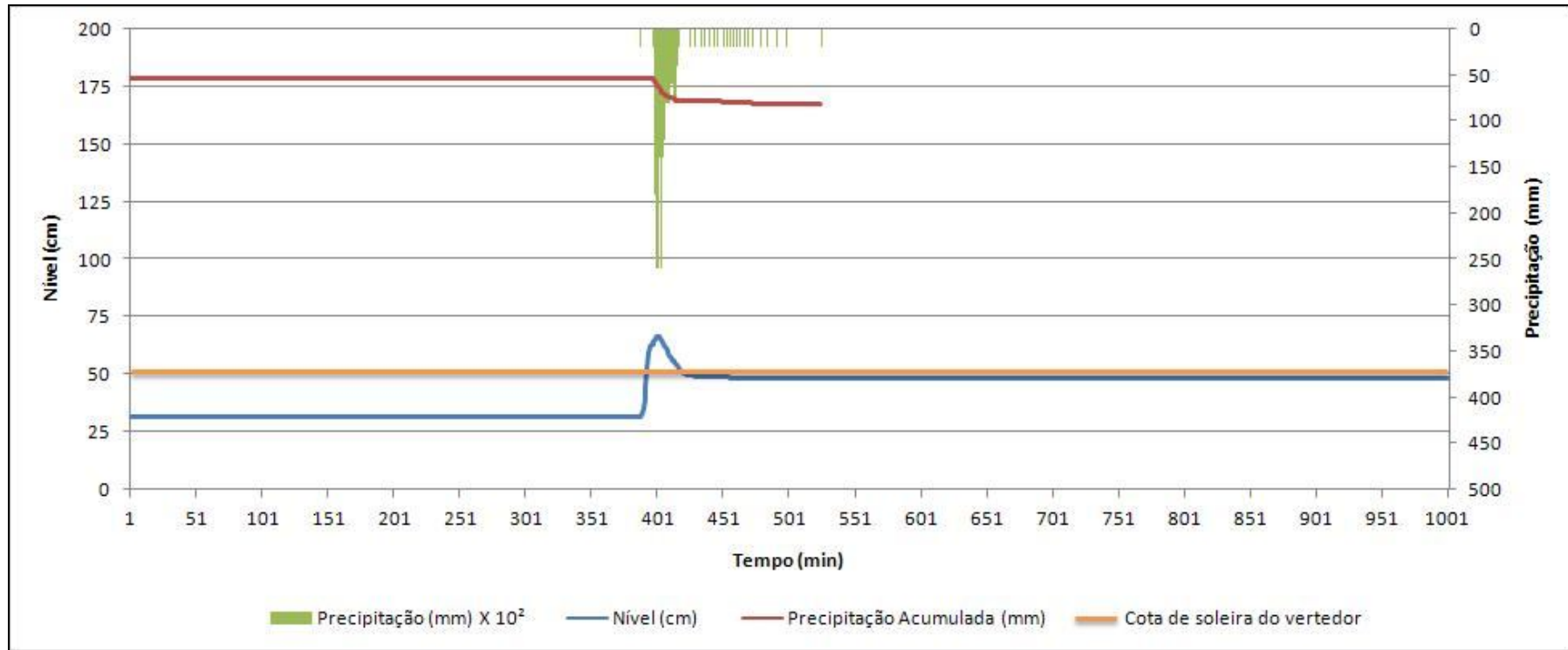
Figura 43 – Registros pluviográficos e linigráficos resultantes do evento pluviométrico erosivo 17 na microbacia.
