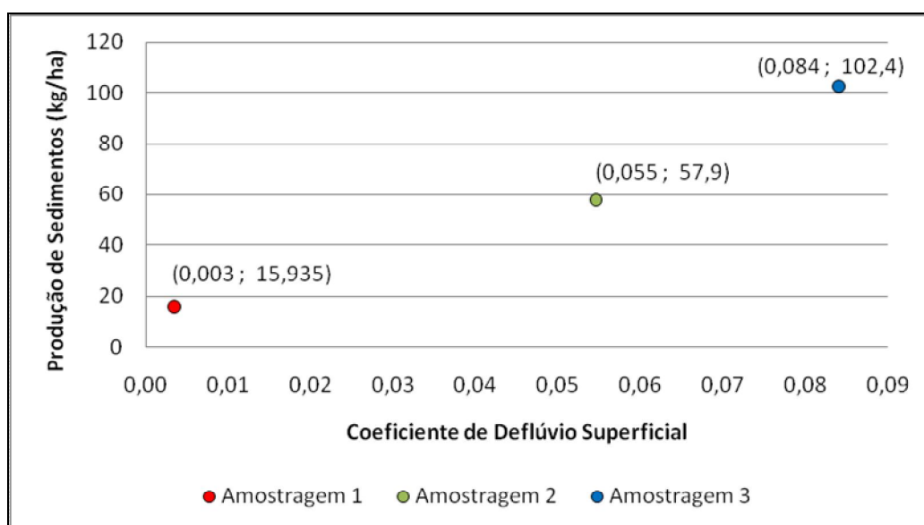
Figura 49 – Relação entre a produção de sedimentos e o coeficiente de deflúvio superficial antecedente à cada amostragem realizada na fossa de sedimentos da microbacia.
