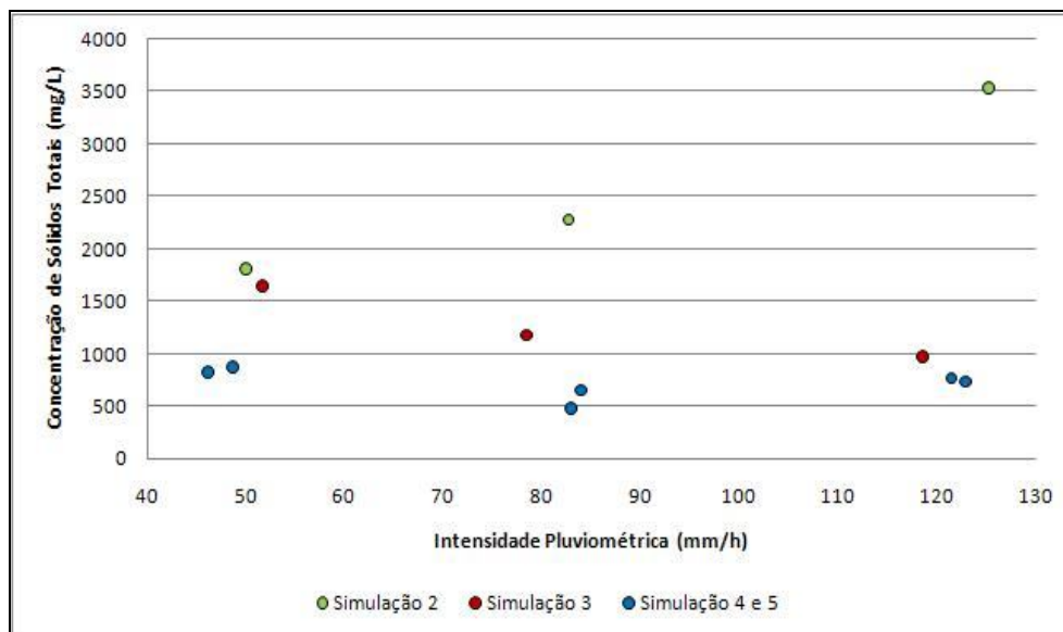
Figura 61 – Relação entre a concentração de sólidos totais e a intensidade pluviométrica de 60 minutos, referente às simulações de chuva nas parcelas experimentais de erosão.
