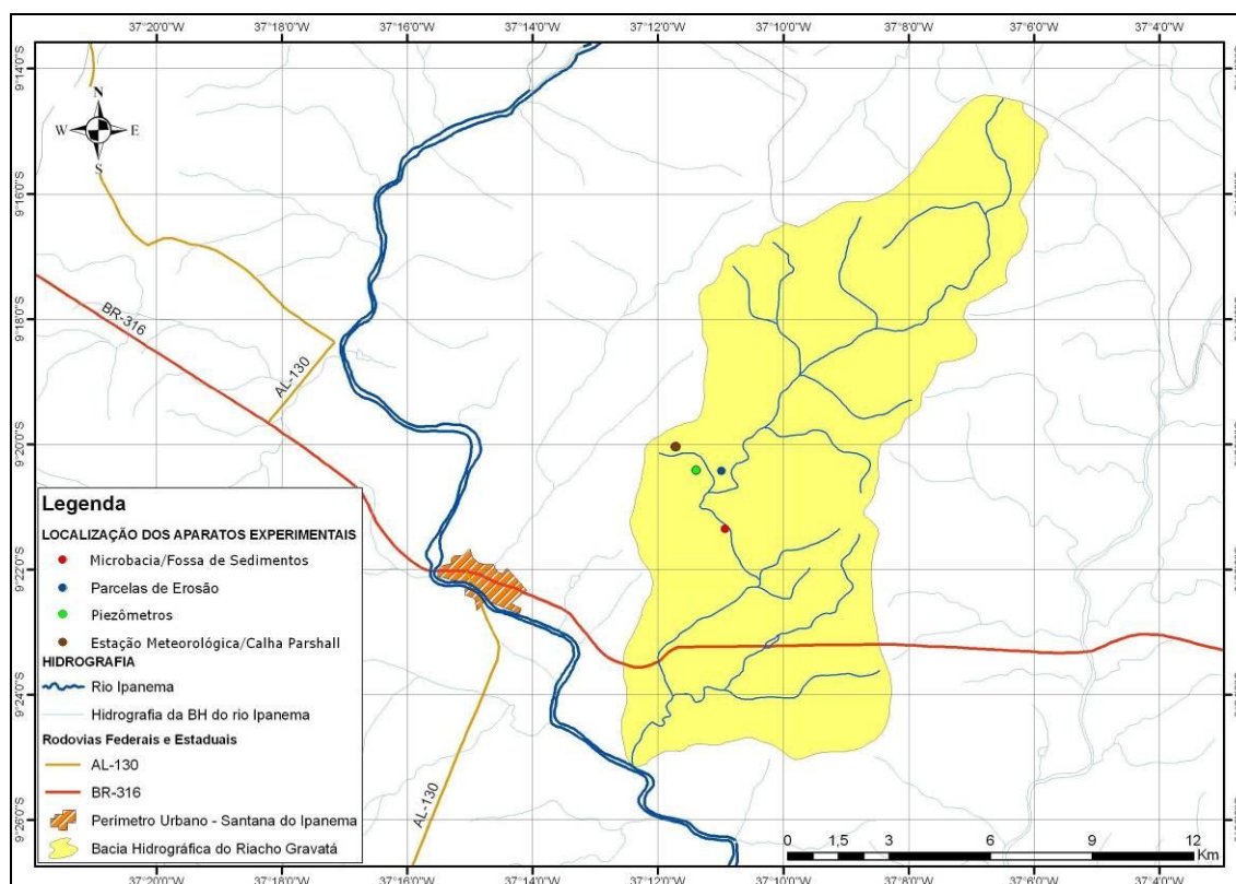
Figura 10 – Aparato experimental na Bacia hidrográfica do riacho Gravatá.
