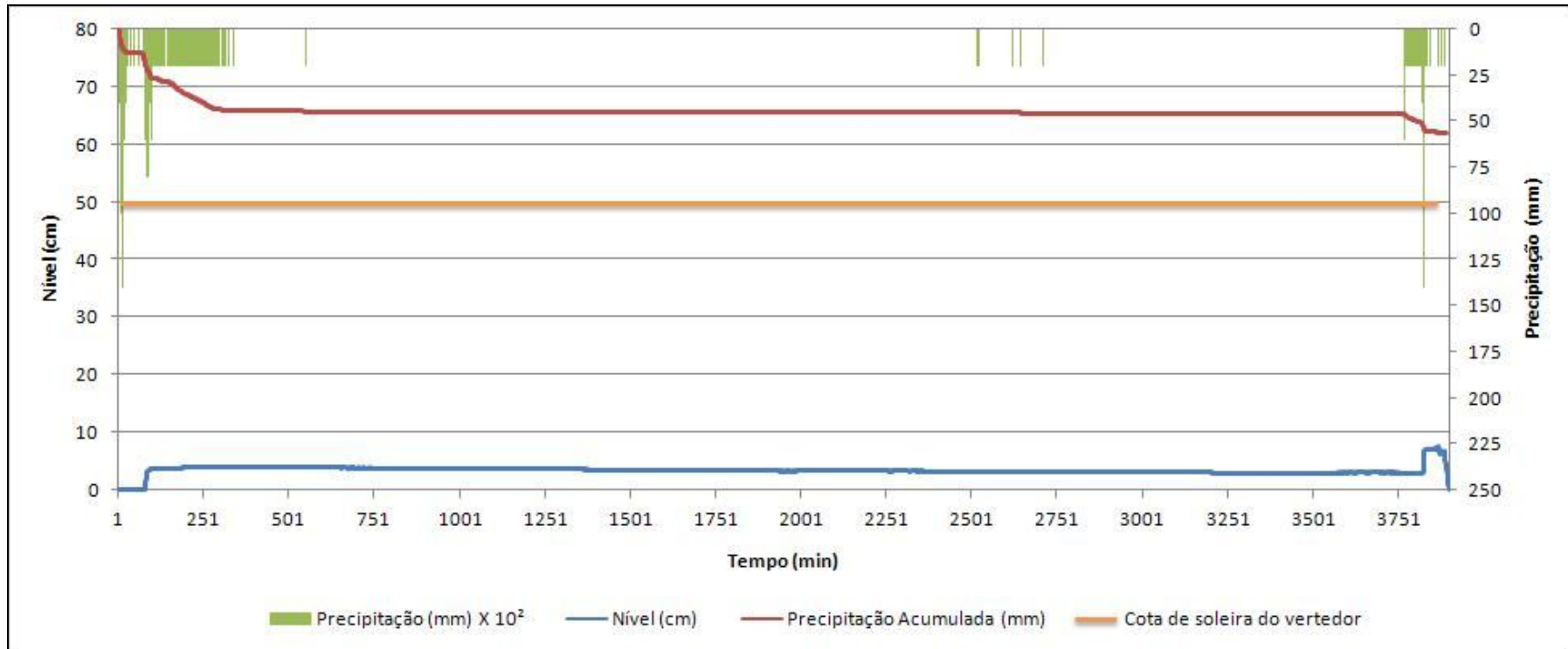
Figura 34 – Registros pluviográficos e linigráficos resultantes dos eventos pluviométricos erosivos antecedentes a Amostragem 1 na microbacia.
