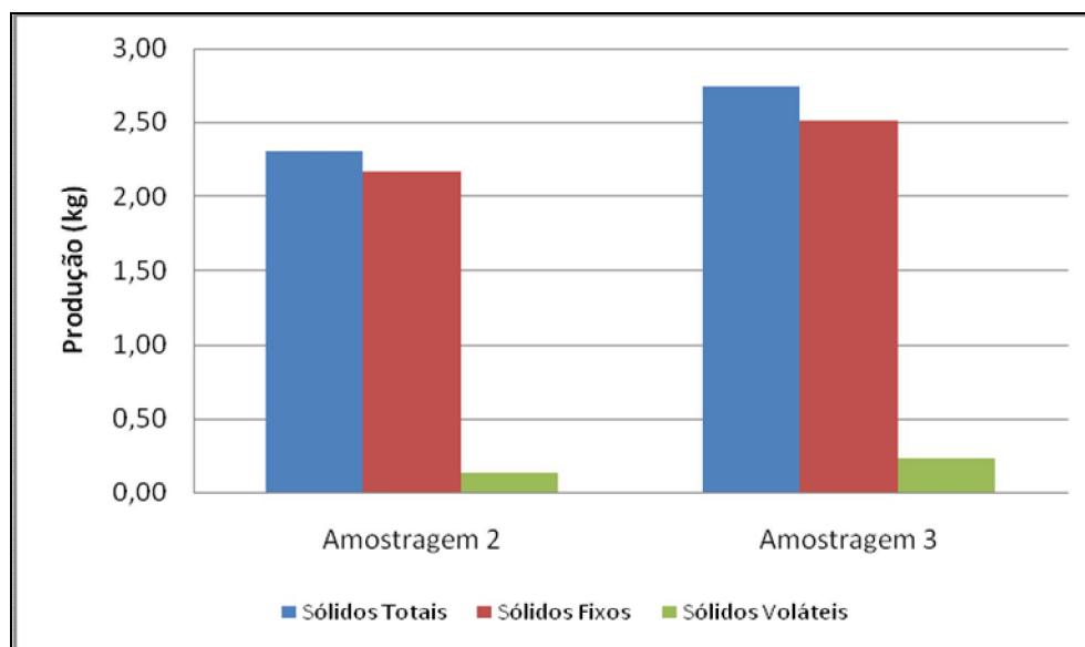
Figura 45 – Produção de sólidos totais, fixos e voláteis, relativa às amostras coletadas nos tubos de amostragem manual, ao longo das duas amostragens realizadas na fossa de sedimentos.
