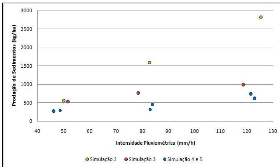
Figura 60 – Relação entre a produção de sedimentos e a intensidade pluviométrica de 60 minutos, referente às simulações de chuva nas parcelas experimentais de erosão.
