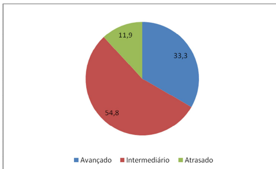
Figura 30 – Distribuição percentual, por padronização pluviométrica, dos eventos pluviométricos erosivos registrados no pluviógrafo da microbacia.
