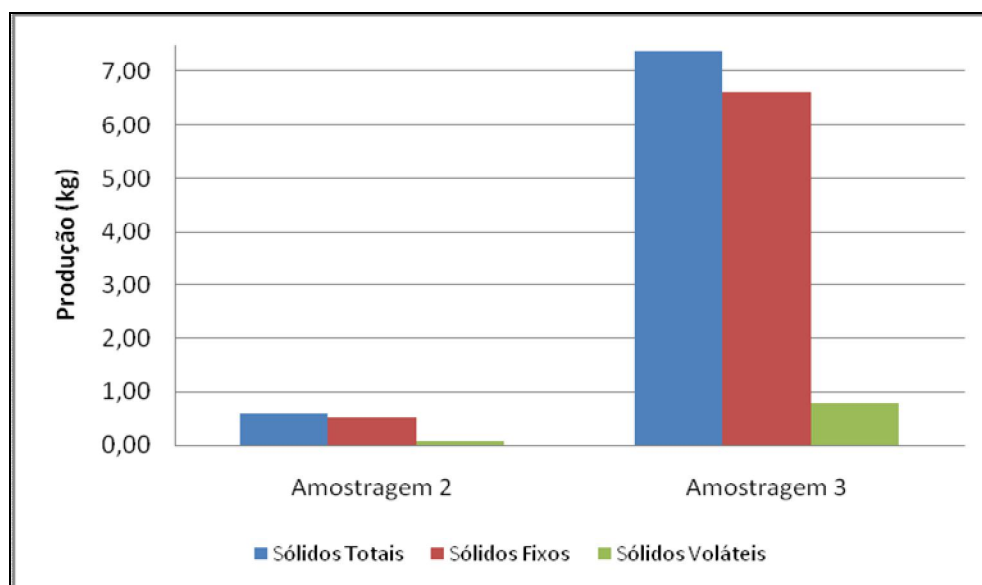
Figura 46 – Produção de sólidos totais, fixos e voláteis, relativa às amostras coletadas nos tubos de amostragem automática, ao longo das duas amostragens realizadas na fossa de sedimentos.
