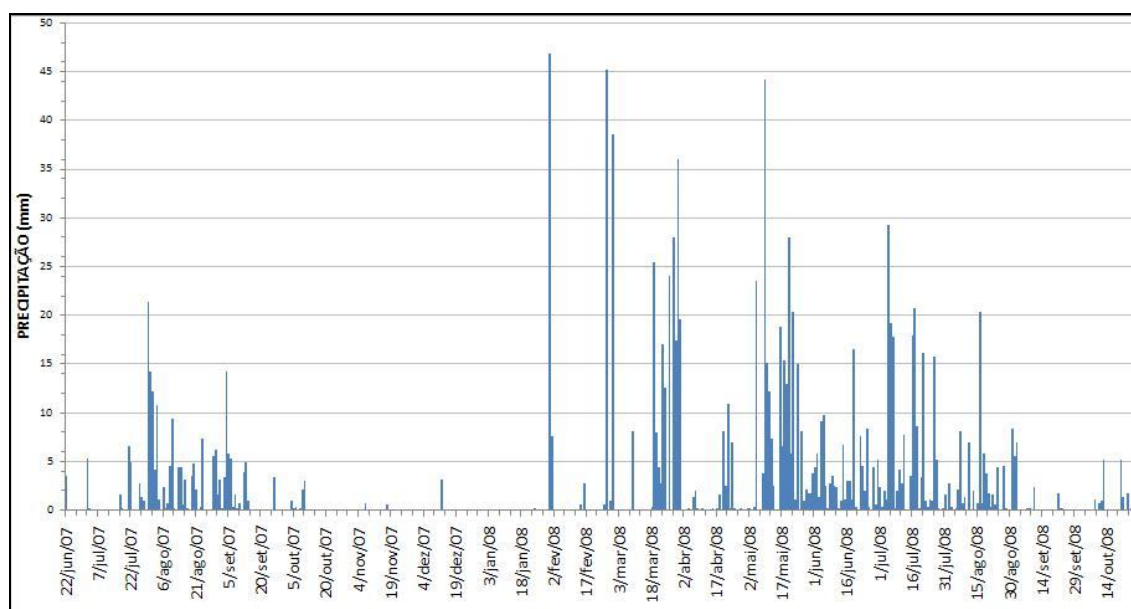
Figura 29 – Precipitação diária registrada no pluviógrafo instalado na microbacia entre os dias 22/06/2007 e 25/10/2008.
