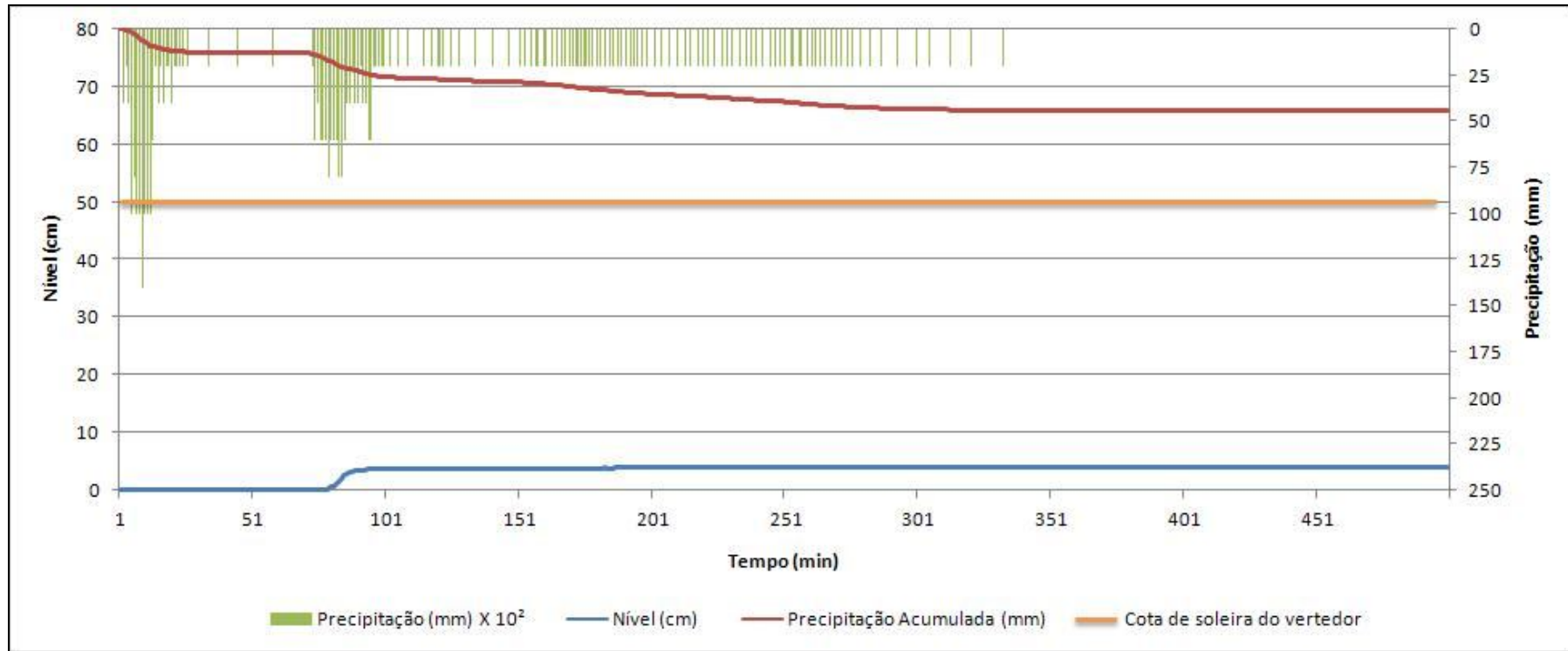
Figura 36 – Registros pluviográficos e linigráficos resultantes do evento pluviométrico erosivo 9 na microbacia.
