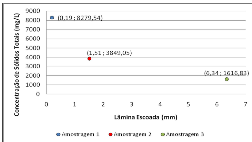
Figura 50 – Relação entre a concentração de sólidos totais e a lâmina total escoada antecedente à cada amostragem realizada na fossa de sedimentos da microbacia.
