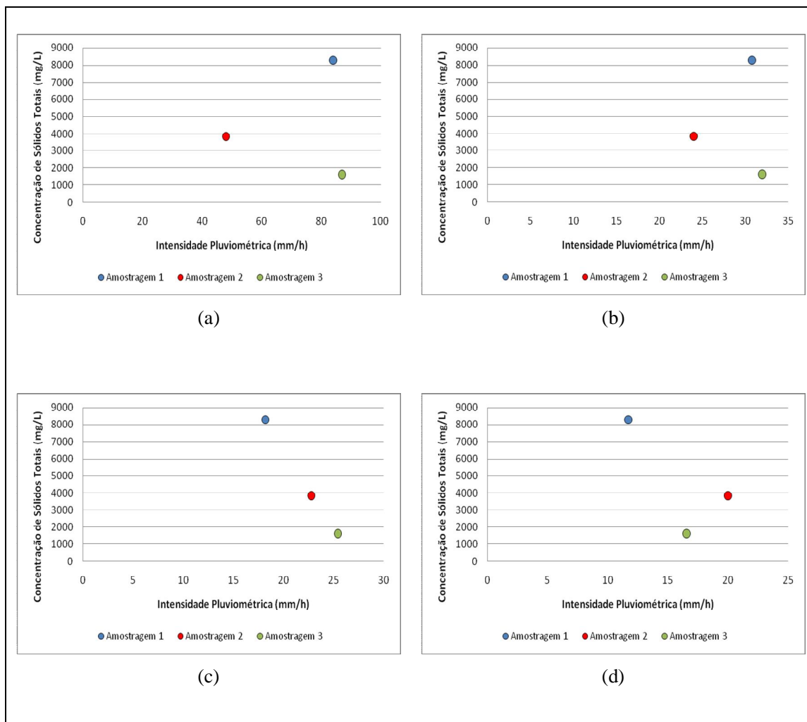
Figura 51 – Relação entre a média das intensidades pluviométricas máximas dos eventos antecedentes à amostragem e a concentração média de sólidos em suspensão da amostragem: (a) Discretização de 1 minuto; (b) Discretização de 15 minutos; (c) Discretização de 30 minutos; e (d) Discretização de 60 minutos.
