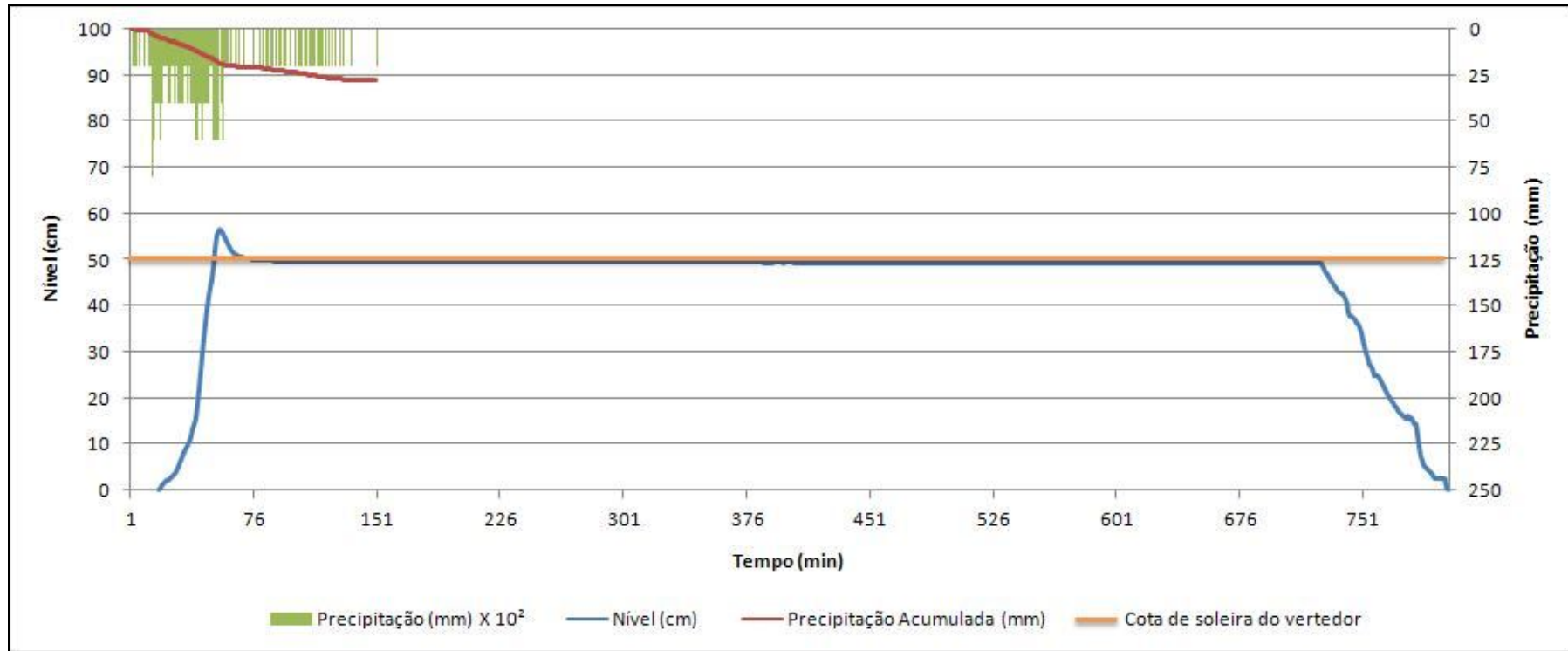
Figura 38 – Registros pluviográficos e linigráficos resultantes do evento pluviométrico erosivo antecedente a Amostragem 2 na microbacia.
