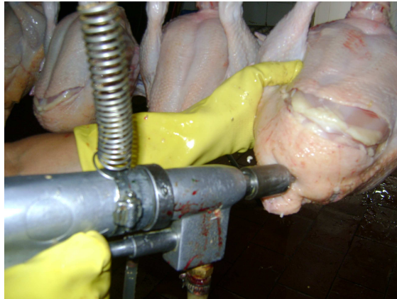
Figura 6. Pistola de oclusão da cloaca.
