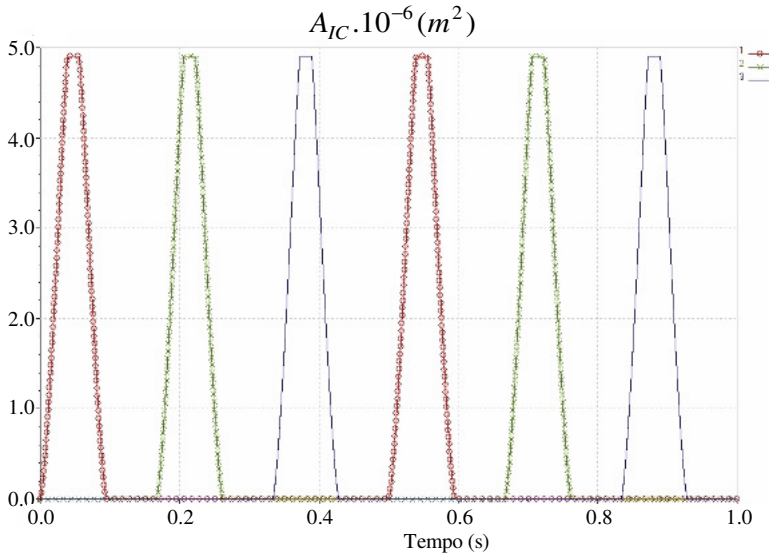
Figura A 4.13 – Área de passagem no tempo para N_{ORIFICIOS} = 2 , N_{DUTOS} = 3 e f_R = 1Hz .
