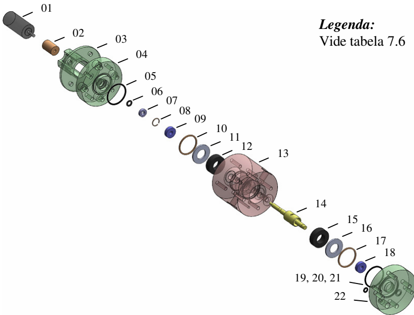
Figura 7.26 – Características e formas geométricas do Protótipo 2 de VRI proposto em vista explodida.
