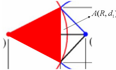
Figura A 4.2 – Área A(R, d_1) em detalhe.
