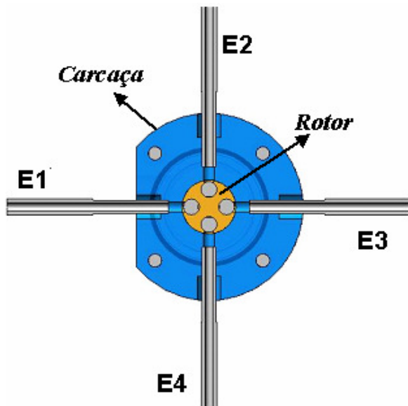
Figura 3.6 – Alinhamento dos orifícios radiais da VRI.
