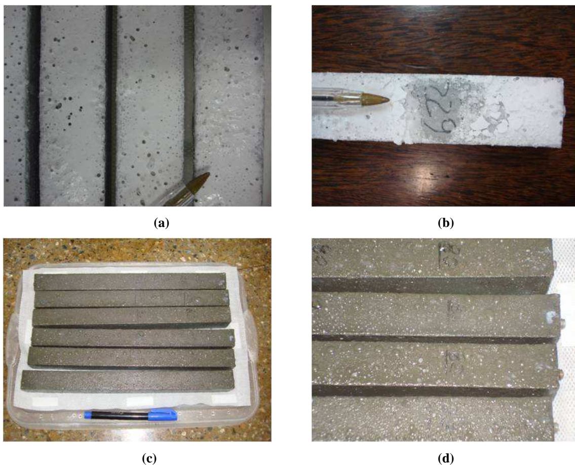
Figura 41: Aspectos gerais das barras. (a) Após imersão na solução com silano metiltrimetoxissilano e água, a 10%; (b) remoção do produto em excesso na superfície; (c) Após imersão na solução com silano octiltriethoxissilano, água e etanol, a 10%; (d) Detalhe da imagem e.
