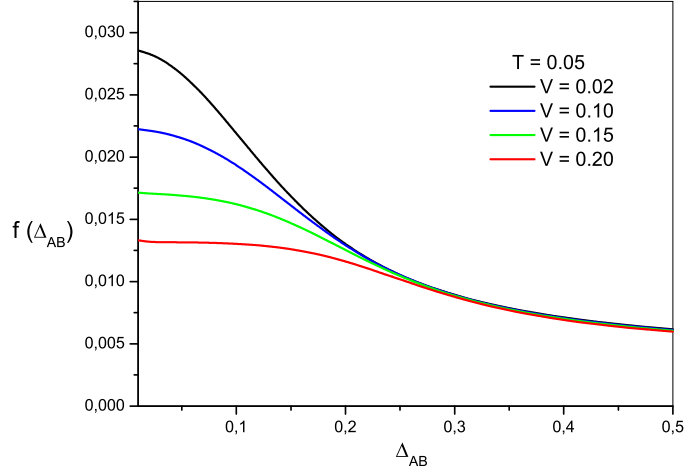
Figura 3.8: Gráfico f(\Delta_{ab}, V) \times \Delta_{ab} , para vários valores de V , com T fixo, todos normalizados por \mu_a .
