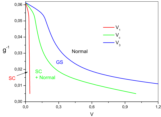
Figura 3.3: Diagrama de fase g^{-1} \times V , normalizado por \mu_a . A sequência de curvas mostra as diferentes regiões do diagrama de fase e os limites de metaestabilidade, onde as fases GS e SC+Normal estão descritas no texto.
