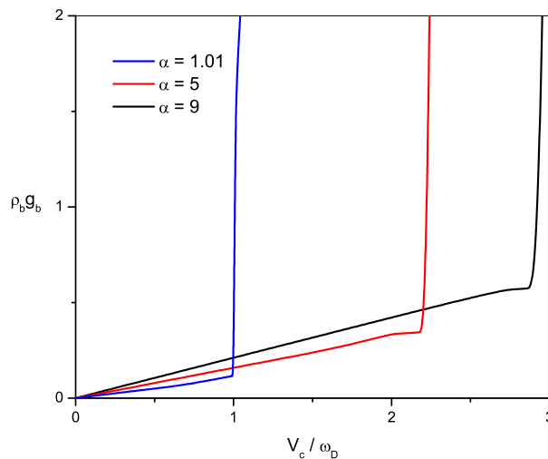
Figura 3.11: Comportamento de V_c obtido numericamente para o caso intra-banda
