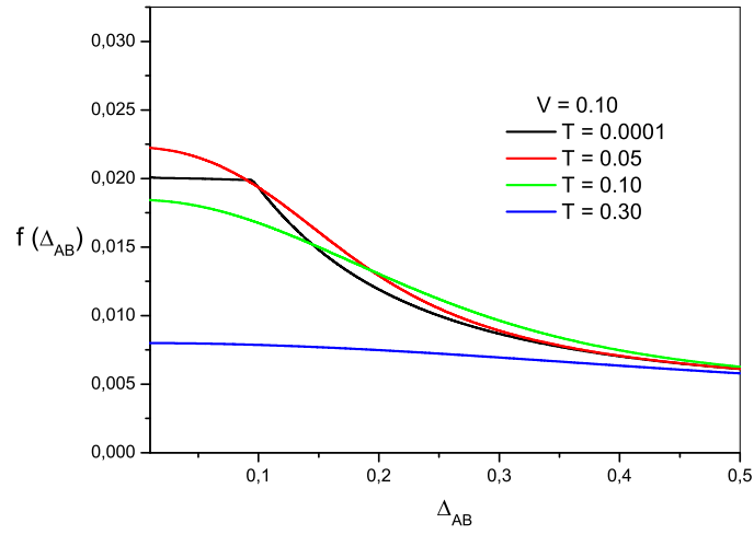
Figura 3.6: Gráfico f(\Delta_{ab}, V) \times \Delta_{ab} , para vários valores de T , com V fixo, onde T = k_B T / \mu_a , V = V / \mu_a e \Delta_{ab} = \Delta_{ab} / \mu_a .
