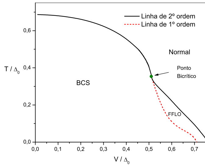
Figura 4.3: Diagrama \frac{T}{\Delta_0} \times \frac{V}{\Delta_0} para um sistema assimétrico na presença de hibridização caracterizando o ponto bicrítico pelo par ordenado (0.510, 0.354) .
