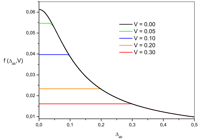
Figura 3.5: Gráfico da função de gap f(\Delta_{ab}, V) \times \Delta_{ab} para diferentes valores de V , ambos \Delta_{ab} e V estão normalizados por \mu_a .
