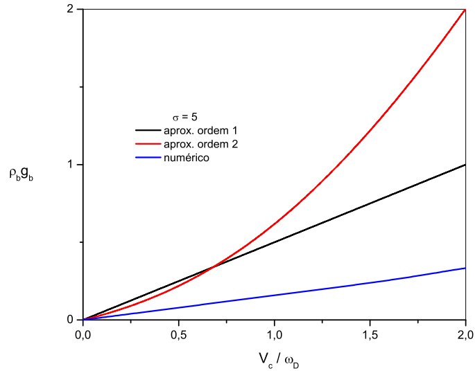
Figura 3.12: Comportamento de V_c para o caso intra-banda comparando todas as aproximações com o caso numérico.
