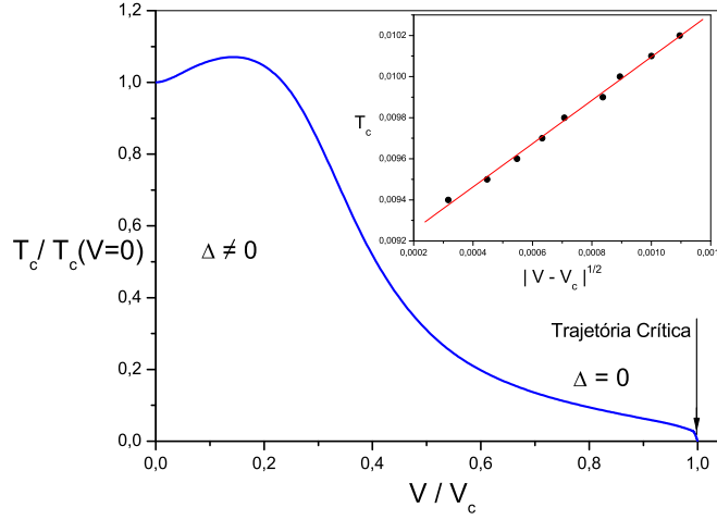
Figura 3.13: Diagrama de fase T_c \times V normalizado das temperaturas críticas supercondutoras como uma função da hibridização. A transição ao longo da linha crítica é contínua e V_c é um ponto crítico quântico supercondutor (PCQS). Em destaque, é mostrado o comportamento de T_c próximo ao PCQS, cujo expoente crítico \frac{1}{2} nos mostra o resultado esperado de um tratamento tipo campo médio.
