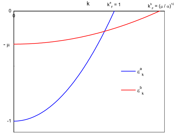
Figura 3.1: Dispersão parabólica das bandas do sistema.
