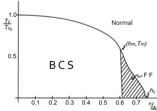
Figura 2.4: Diagrama de fase T_c \times h obtido por Takada e Izuyama [16], onde as transições do estado supercondutor para o normal são sempre de segunda ordem enquanto a transição da fase BCS para a FFLO é de primeira ordem.
