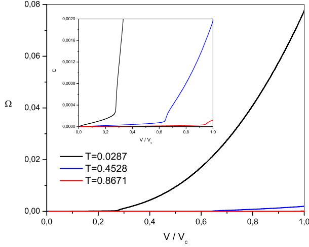
Figura 3.9: Gráfico da razão \Omega = \frac{\sum \langle b_{-k} a_k \rangle}{\sum \langle b_{-k} b_k \rangle} \times \frac{V}{V_c} para vários valores de temperatura normalizadas. Em destaque mostra o comportamento para valores em torno de zero da razão \Omega .
