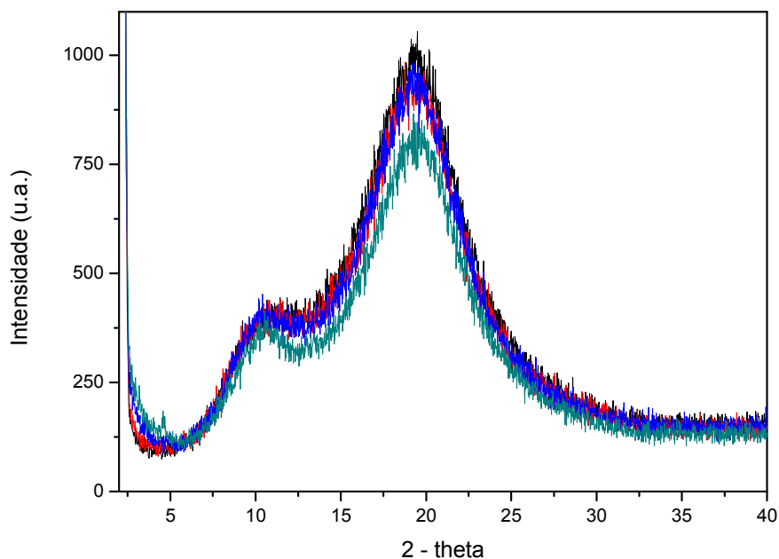
Figura 5.10 – Difratomogramas de raios-X do HIPS (linha preta) e dos nanocompósitos deHIPS: 3a (linha vermelha), 3b (linha azul) e 3c (linha verde).
