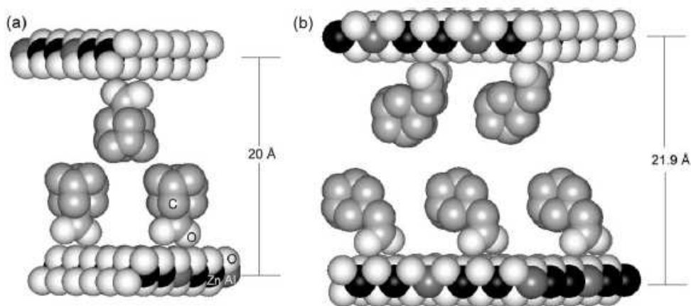
Figura 3.7 – Modelo computacional para os prováveis arranjos de (a) 1-ácido adamantancarboxílico e (b) 1-ácido adamantanoacético entre as lamelas da hidrotalcita. 70
