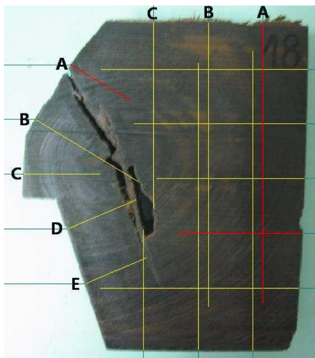
FIGURA B.18 – Resultados obtidos para a fatia 18, referente à posição 18-19 dos transdutores de frequência de 500 kHz.
