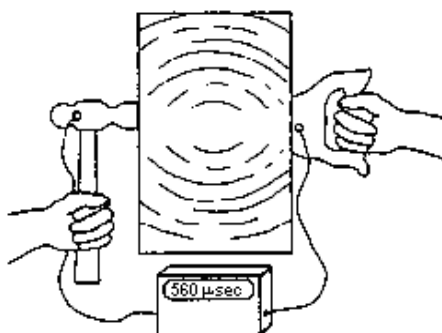
FIGURA 2.4 – Representação esquemática do equipamento medidor de ondas de tensão.
