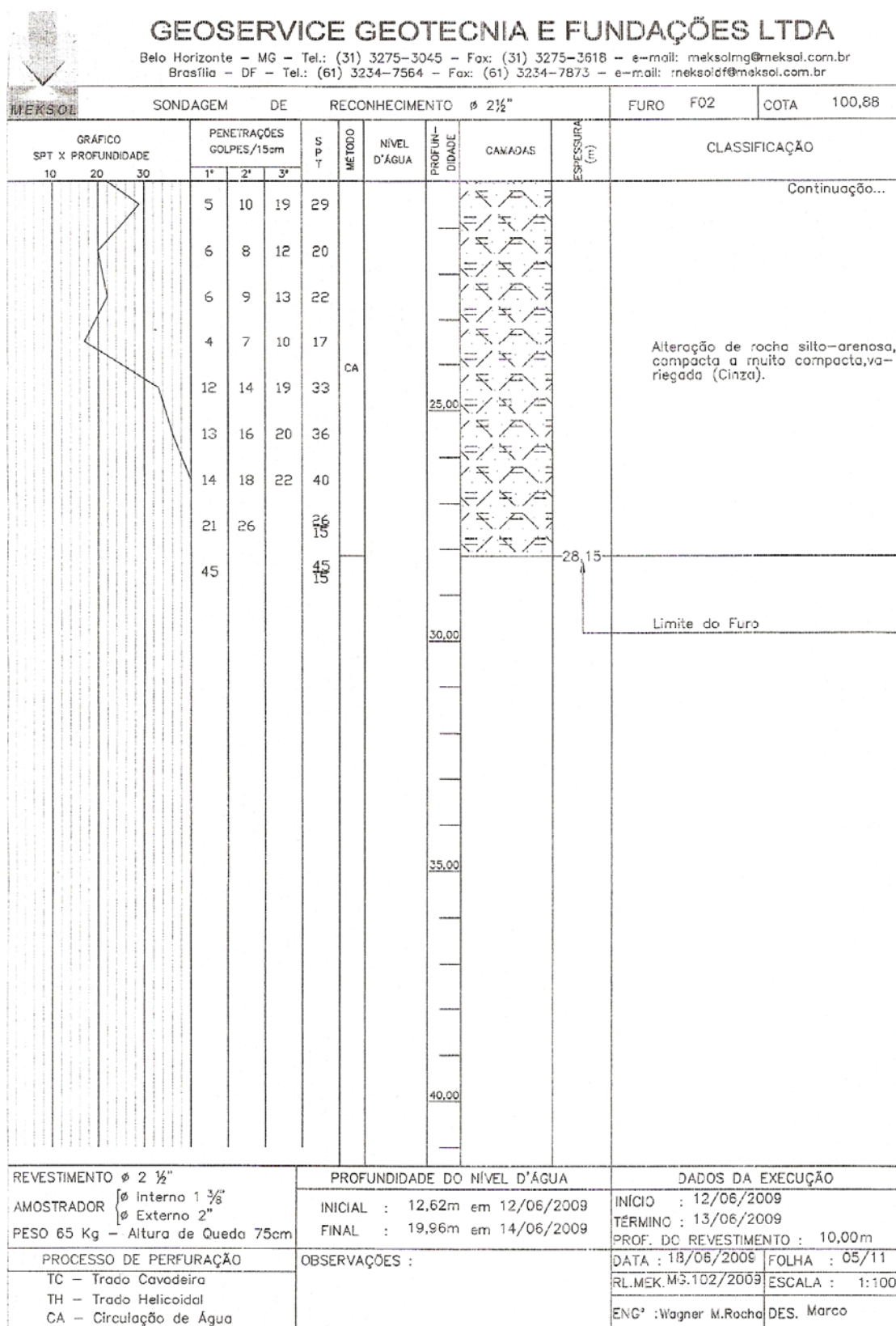
FIGURA A.3 – Relatório de Sondagem 2 (2/2).
