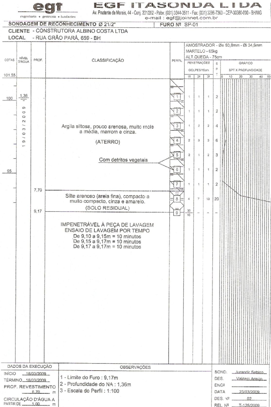
FIGURA A.4 – Relatório de Sondagem 3.
