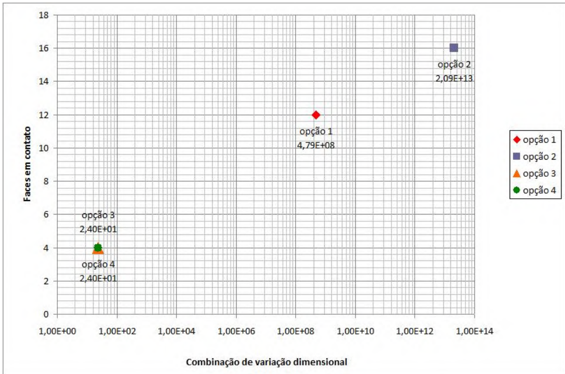
Figura 45: Curva de correlação – faces em contato x combinação de variação dimensional.
