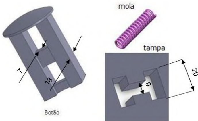
Figura 41: Configuração de sinalizador existente em outro produto.
