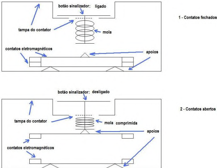
Figura 40: Princípios de solução do sinalizador.
