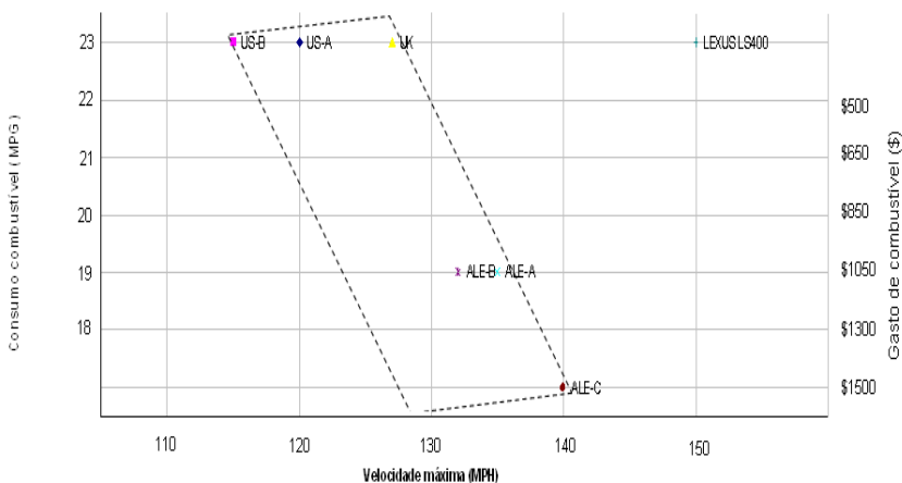
Figura 24: Curva correlação - ajuste de meta de velocidade e consumo.
