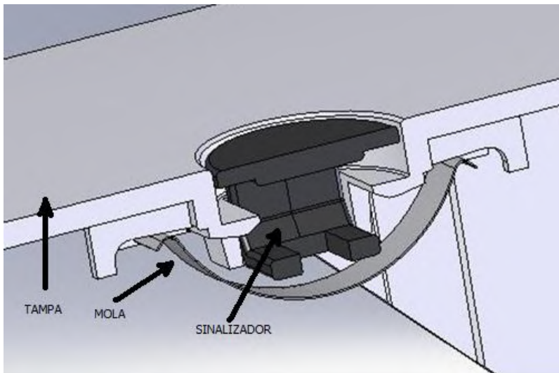
Figura 47: Montagem do sinalizador.
