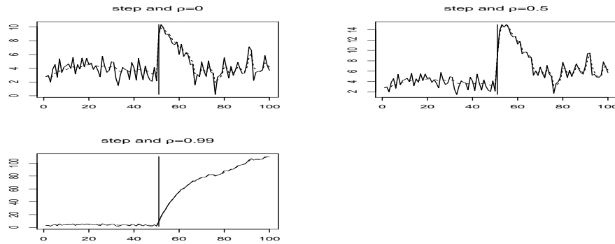
Figura 4.3: Exemplos da função degrau para o Modelo 2, com n = 100 e \rho = 0.00, 0.50 e 0.99 . A linha vertical indica o instante da intervenção, T = 50 , a linha contínua indica a série, y_t , e a linha tracejada indica a resposta média \alpha_t .
