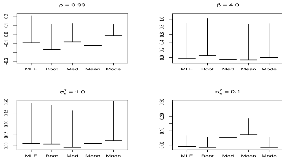
Figura 4.4: Máxima verossimilhança, bootstrap e estimação Bayesiana para o Modelo 1 com função pulso e \rho = 0.99 . As linhas horizontal e vertical (o comprimento da linha) indicam o vício e a raiz quadrada do EQM, respectivamente.
