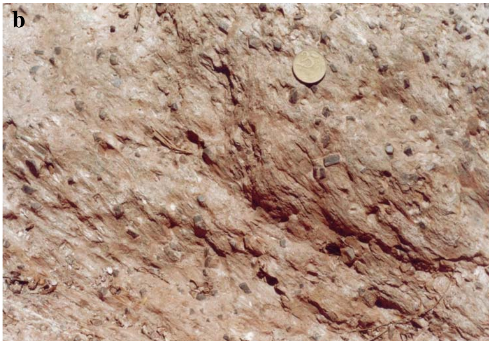
Figura 4.16- a) Veios de quartzo, cianita, granada, clinozoisita em cianita-granada-estaurolita micaxisto a oeste da área de estudo próximo a Braquianticlinal do Lontra. b) Detalhe do estaurolita-granada micaxisto onde destacam-se porfiroblastos de granada e estaurolita.
