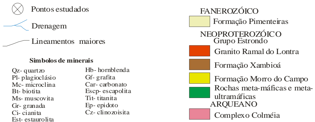
Figura 6.1- mapa geológico simplificado da região de Xambioá-Araguanã, com distribuição das principais associações minerais que definem o metamorfismo na área. Modificado de CPRM(2000).
