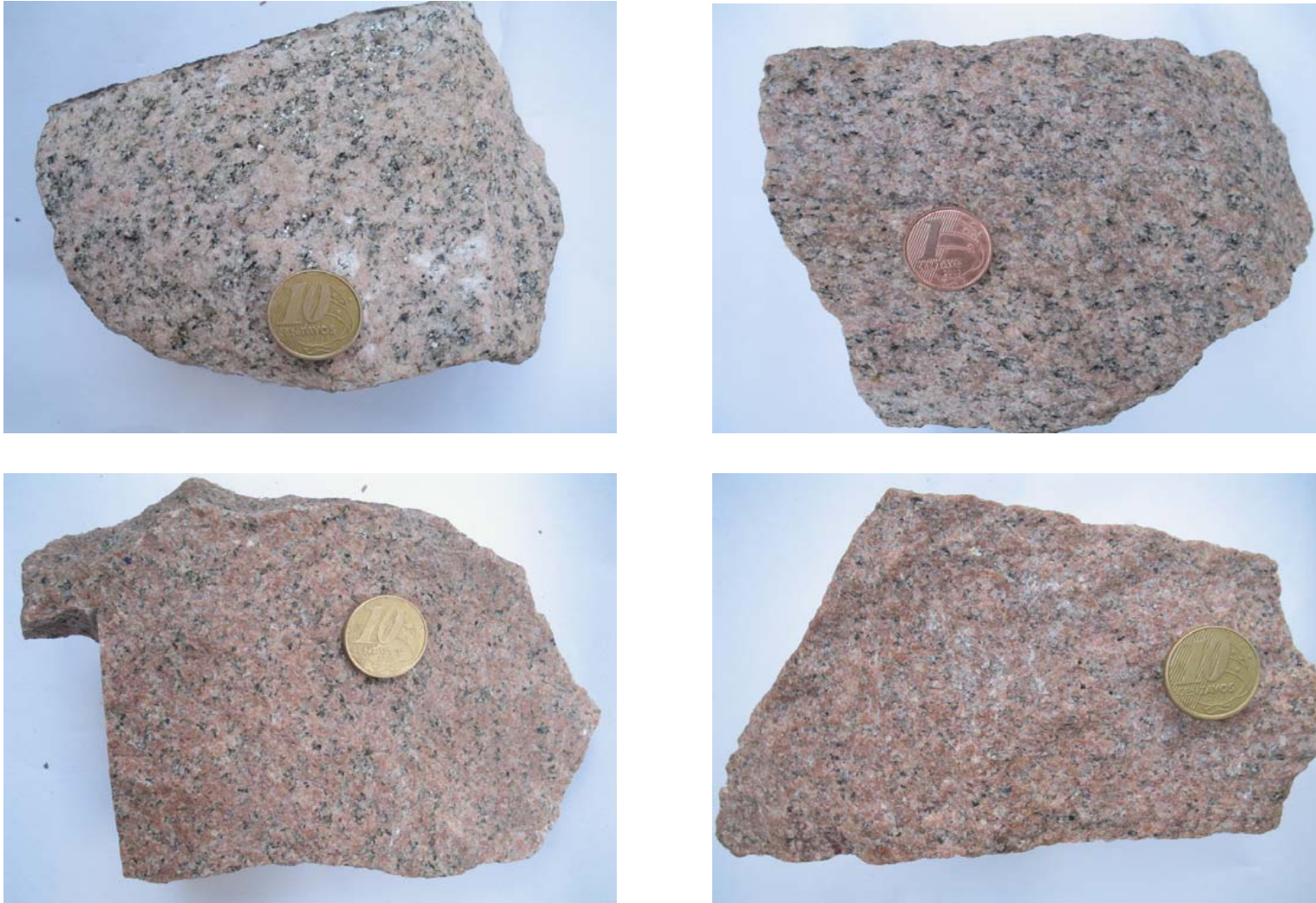
Figura 5.2- Aspectos macroscópicos do Granito Ramal do Lontra.
