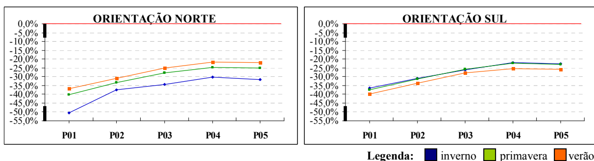
Gráfico 3-04 – Gráficos da diferença percentual entre a “Janela em Sacada” com beiral e a “Janela em Sacada” por período do ano nas orientações Norte, Leste, Sul e Oeste.
