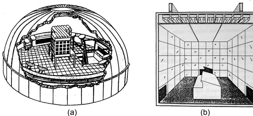
Figura 1-28 – Simuladores de Céu: a vista de uma “Cúpula de Céu” ou “Sky Dome” (a) e a vista de um Simulador “Céu de Espelho” ou “Mirror Sky” (b). Fonte: Baker e Steemers (2002) (a, b).
