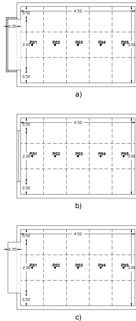
Figura 2-09 – Modelos para simulações: “Janela em Sacada” versus janela simples e “Janela em Sacada” versus janela simples com beiral: Planta Modelo de “Janela em Sacada”, com malha de estudo de 5x1 (a); Planta Modelo de janela simples, com malha de estudo 5x1 (b); Planta Modelo de janela simples com beiral, com malha de estudo 5x1 (c).
