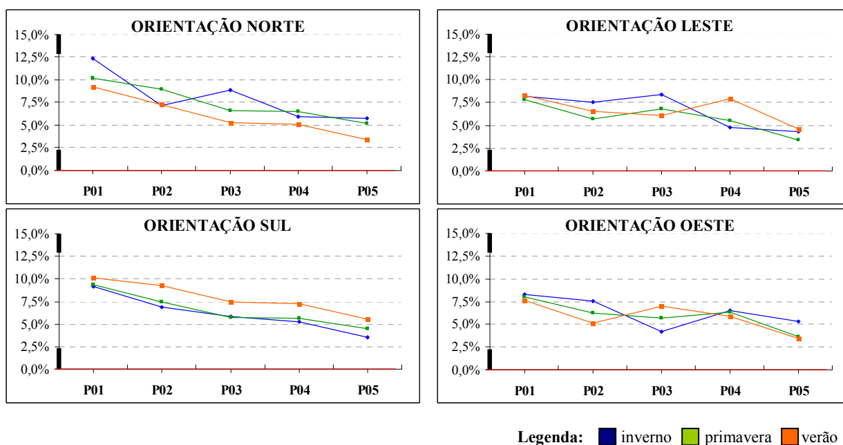
Gráfico 3-02 – Gráficos da diferença percentual entre a “Janela em Sacada” e a janela simples com beiral por período do ano nas orientações Norte, Leste, Sul e Oeste.
