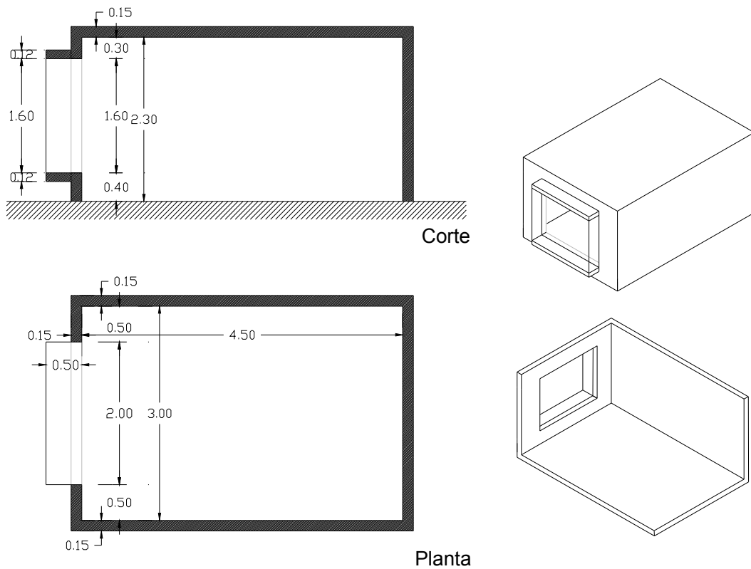
Figura 2-05 – Localização e dimensões da “Janela em Sacada”, mostradas em corte longitudinal, planta e isométrica externa e interna.
