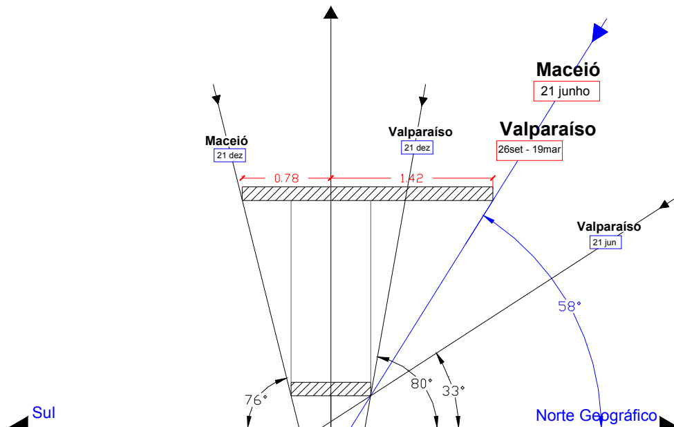
Figura 2-12 – Angulo de proteção solar às 12h nas orientações Norte e Sul, e dimensões do beiral da “Janela em Sacada” para a cidade de Maceió e Valparaíso.
