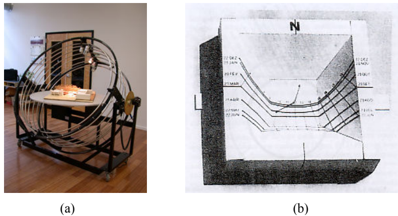
Figura 1-29 – Simuladores do Sol: o “Heliodon” (a) e o Relógio de Sol (b). Fonte: www.philau.edu (a), Baker e Steemers (2002) (b).
