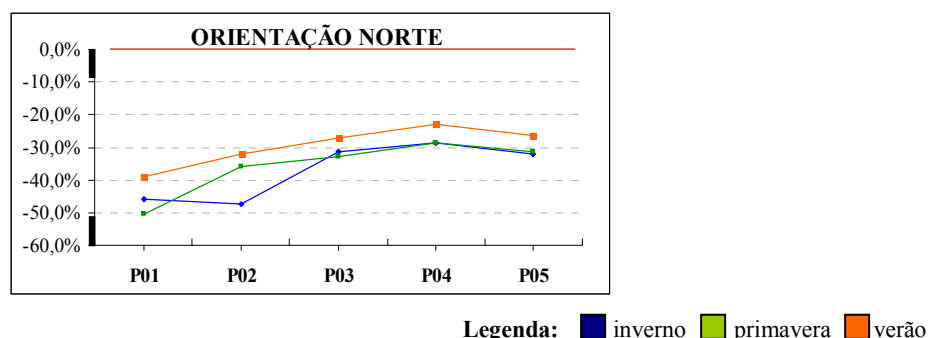
Gráfico 3-08 – Gráficos da diferença percentual entre a “Janela em Sacada” com beiral e a “Janela em Sacada” por período do ano na orientação Norte.
