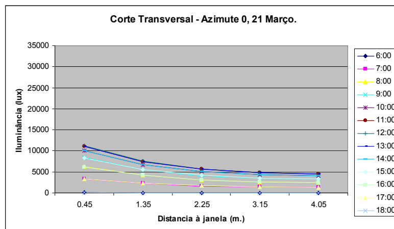
Gráfico 2-03 – Modelo (exemplo) de gráfico de iluminâncias na seção transversal da sala, observando-se a distribuição e o valor das iluminâncias.
