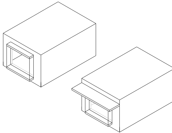
Figura 2-07 – “Janela em Sacada” sem e com o protetor solar, em isométrica.
