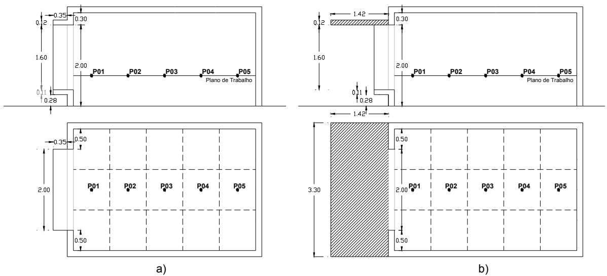
Figura 2-11 – Modelos de “Janela em Sacada” simples e “Janela em Sacada” com beiral para a fase 3 das simulações (corte e planta). “Janela em Sacada” sem beiral (a), “Janela em Sacada” com beiral (b).
