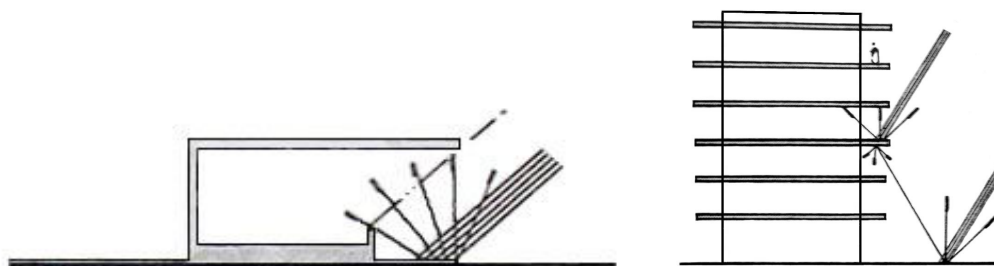
Figura 1-20 – O Beiral como protetor solar e o aproveitamento da luz refletida do exterior (a) e edifícios que controlam a radiação direta e geram radiação refletiva em seus planos inferiores (b).
