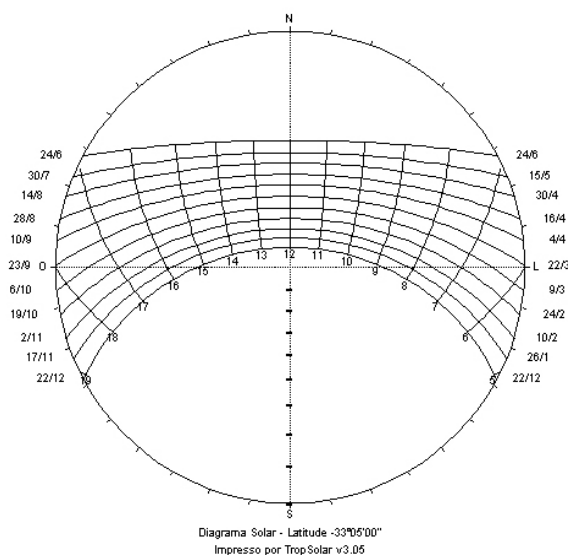
Figura 1-25 – Carta solar de Valparaíso. Fonte: Figura gerada pelo software TropSolar, Cabús (2007).
