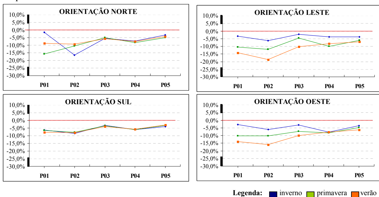
Gráfico 3-05 – Gráficos da diferença percentual entre a “Janela em Sacada” e a janela simples por período do ano nas orientações Norte, Leste, Sul e Oeste.
