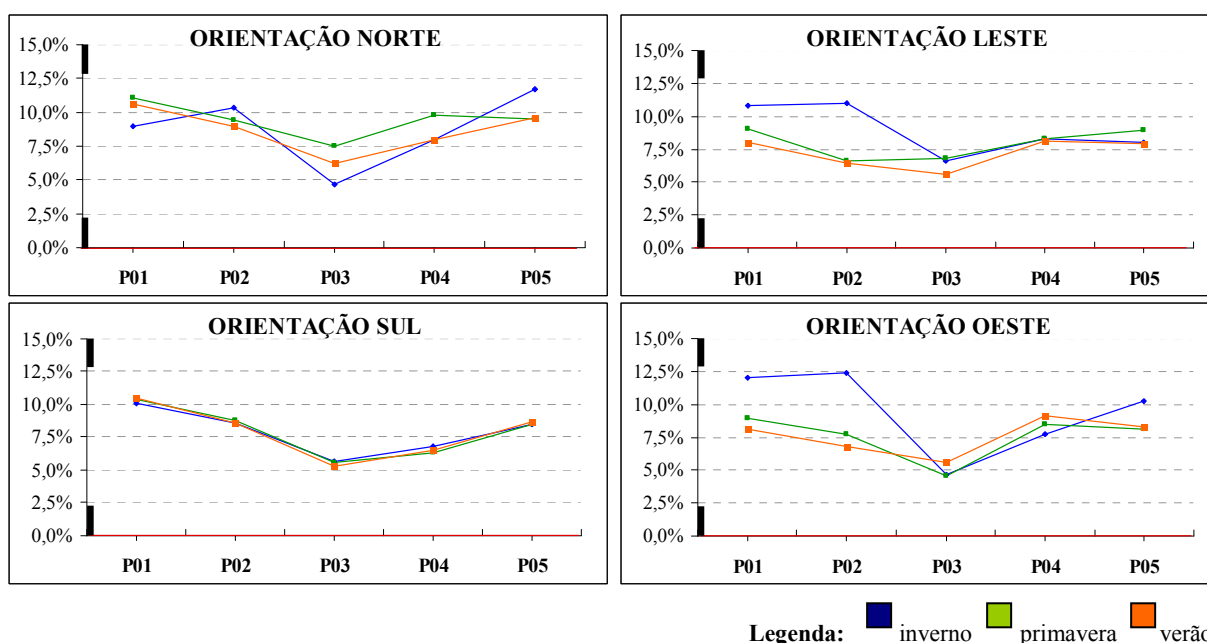
Gráfico 3-06 – Gráficos da diferença percentual entre a “Janela em Sacada” e a janela simples com beiral por período do ano nas orientações Norte, Leste, Sul e Oeste.
