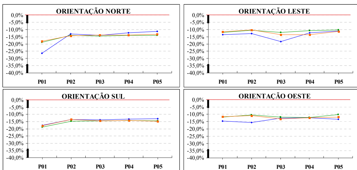
Gráfico 3-03 – Gráficos da diferença percentual entre a “Janela em Sacada” com ambos os planos laterais opacos e a “Janela em Sacada” com ambos os planos laterais transparentes por período do ano nas orientações Norte, Leste, Sul e Oeste.
