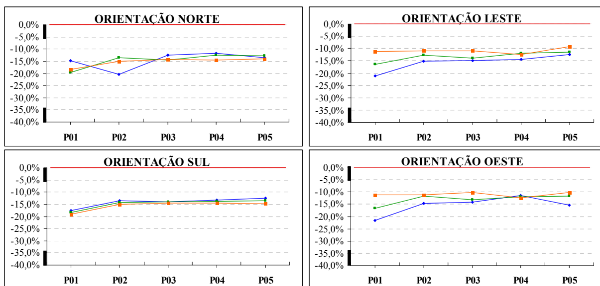
Gráfico 3-07 – Gráficos da diferença percentual entre a “Janela em Sacada” com ambos os planos laterais opacos e a “Janela em Sacada” com ambos os planos laterais transparentes por período do ano nas orientações Norte, Leste, Sul e Oeste.
