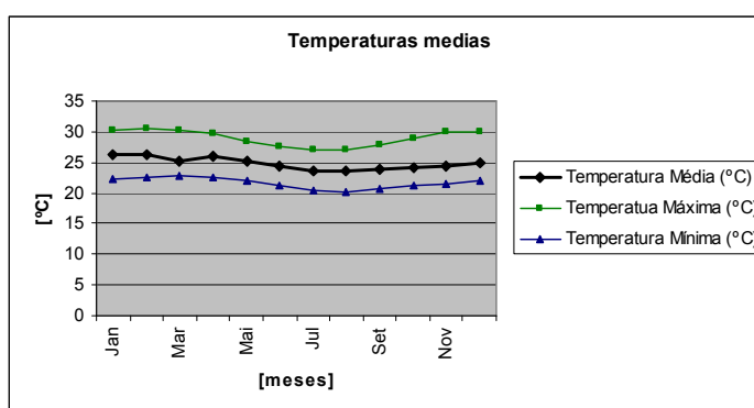
Gráfico 1-01 – Temperatura média mensal, Maceió.
