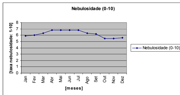
Gráfico 1-05 – Nebulosidade mensal, Maceió. Fonte: Cabús (2002).
