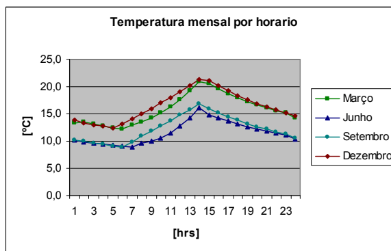
Gráfico 1-08 – Temperaturas horárias, Valparaíso.
