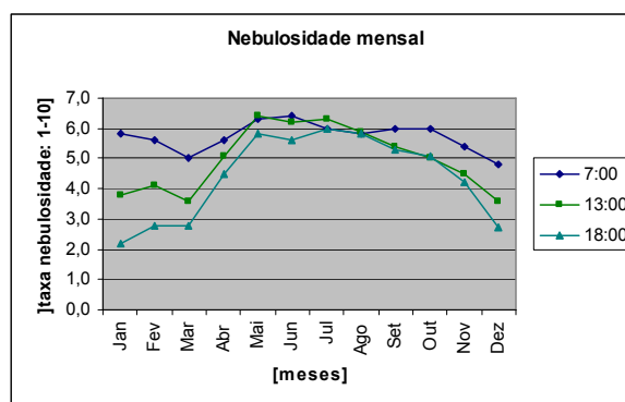
Gráfico 1-12 – Nebulosidade mensal para 3 horários do dia, Valparaíso.
