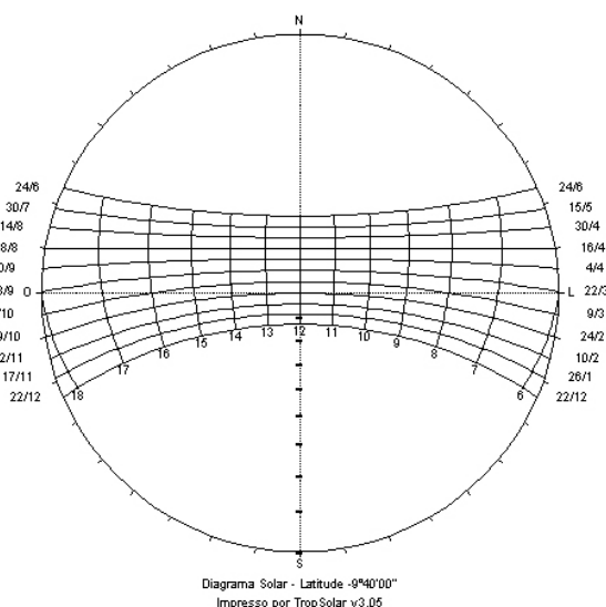
Figura 1-22 – Carta solar de Maceió.
