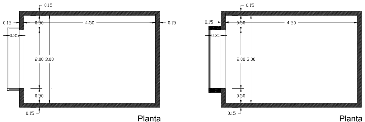
Figura 2-06 – Transparência ou opacidade dos planos laterais da “Janela em Sacada”, em planta.
