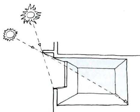
Figura 1-19 – O Beiral como proteção solar no verão, deixando entrar o Sol no inverno. Fonte: Mendizabal (1988).
