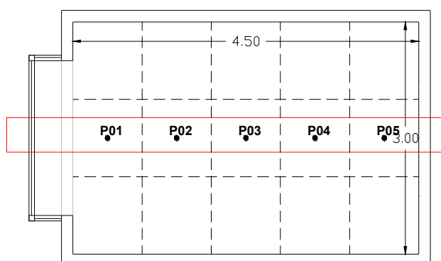
Figura 2-13 – Seção transversal escolhida para o estudo dos modelos.
