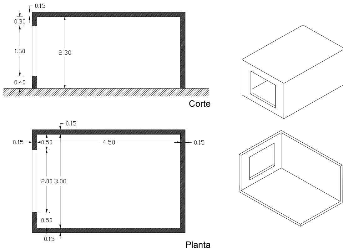
Figura 2-03 – Sala de referência em corte longitudinal, planta e isométrica, externa e interna, mostrando as dimensões e configurações da sala.
