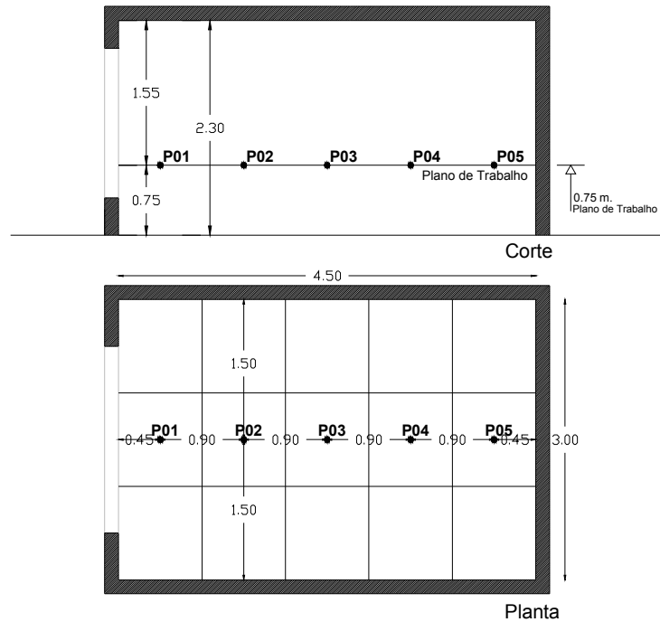
Figura 2-08 – Localização do plano de trabalho e organização da malha de pontos para realização das simulações, no corte e na planta.
