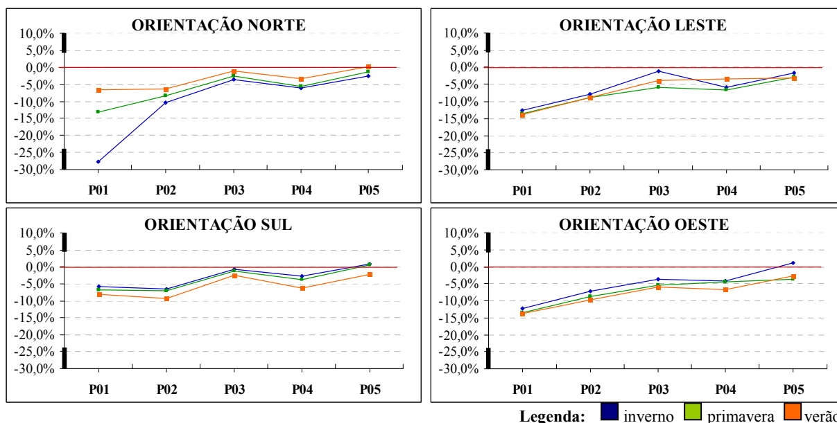
Gráfico 3-01 – Gráficos da diferença percentual entre a “Janela em Sacada” e a janela simples por período do ano nas orientações Norte, Leste, Sul e Oeste.
