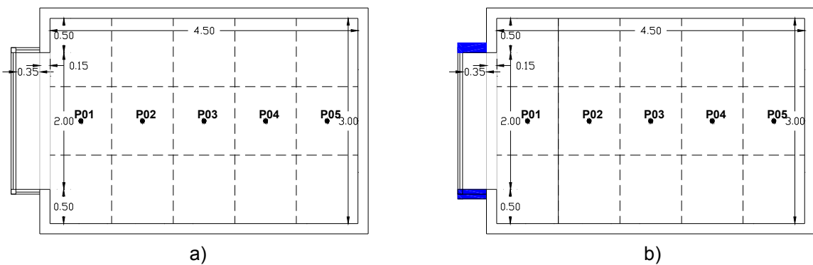
Figura 2-10 – Modelos para simulações: 2 exemplos com diferente materialidade nos planos laterais. "Janela em Sacada" com ambos os planos laterais transparentes (a); "Janela em Sacada" com ambos os planos laterais opacos (b).
