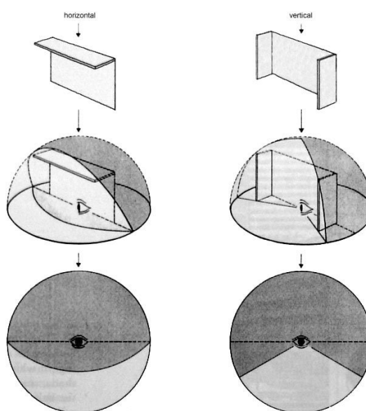
Figura 1-18 – Proteção mediante de dispositivos fixos: horizontal superior e vertical lateral.
