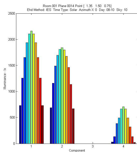
Gráfico 2-04 – Exemplo de gráfico de detalhamento das componentes da luz, segundo a Tabela 3-04, para cada ponto da malha, observando-se a presença e os níveis de luz direta de céu (1), refletida de céu (2), direta de Sol (3) e refletida de Sol (4).
