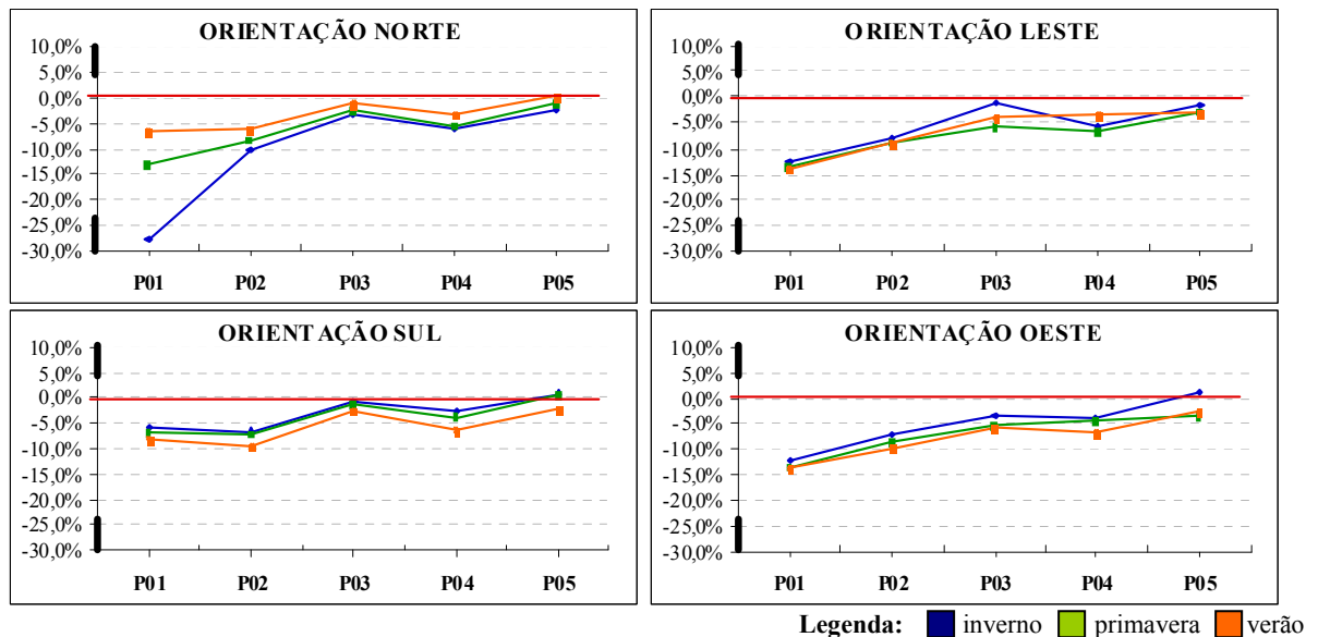
Gráfico 2-02 – Exemplo de gráficos da variação percentual do desempenho luminoso entre janelas, mediante a média das horas do dia por período do ano, nas orientações Norte, Leste, Sul e Oeste.
