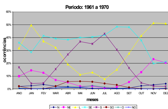
Gráfico 1-03 – Frequência de ventos, Maceió.
