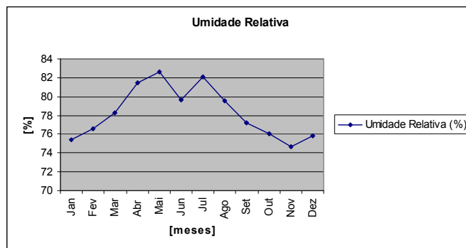
Gráfico 1-02 – Umidade Relativa, Maceió.
