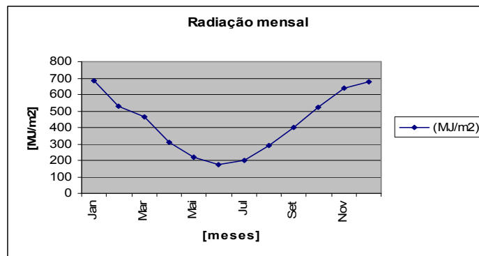
Gráfico 1-13 – Radiação mensal [ \text{MJ}/\text{m}^2 ], Valparaíso.
