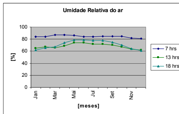
Gráfico 1-09 – Umidade Relativa, Valparaíso.
