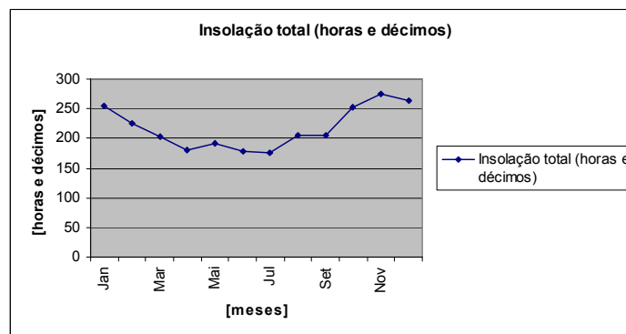
Gráfico 1-06 – Insolação mensal total, Maceió.
