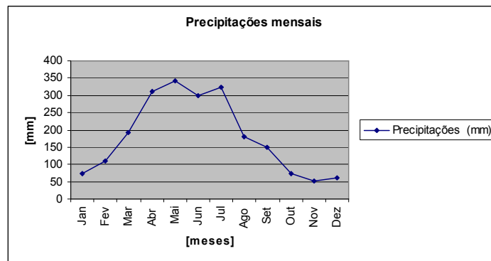
Gráfico 1-04 – Precipitações mensais, Maceió. Fonte: Cabús (2002).
