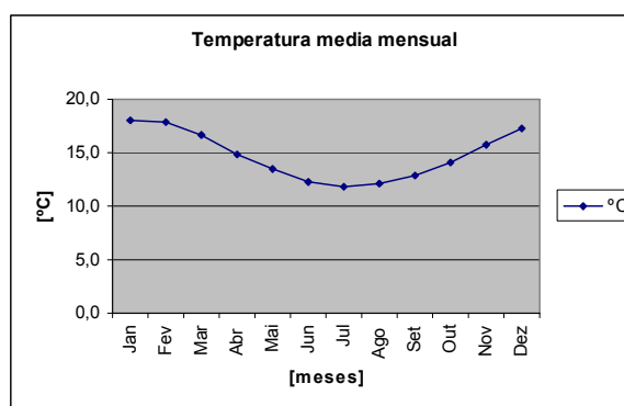
Gráfico 1-07 – Temperaturas médias, Valparaíso.
