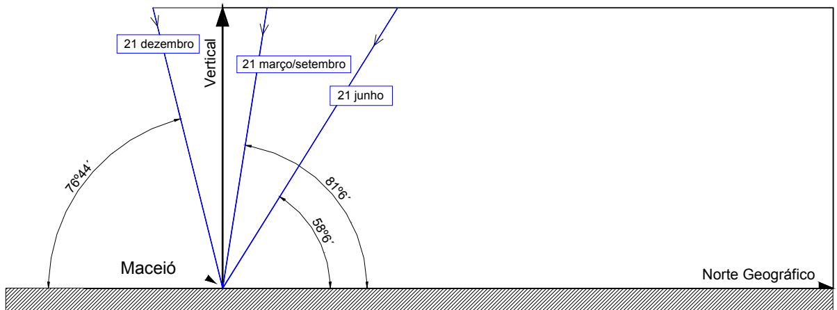
Figura 1-23 – Ângulos de altura solar ao meio-dia em Maceió.
