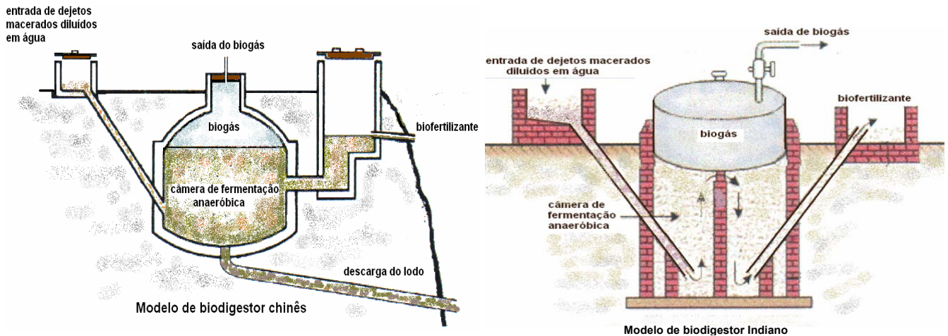
Figura 7-Modelos de biodigestores chineses e indianos. Fonte: WINROCK, 2008
