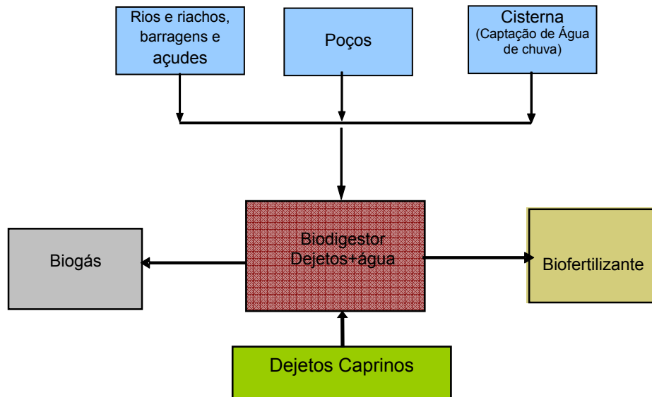
Figura 36-Esquema de ligação das fontes hídricas Fonte: Elaboração da autora, 2009
