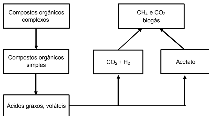
Figura 6-Estágios da biodigestão
