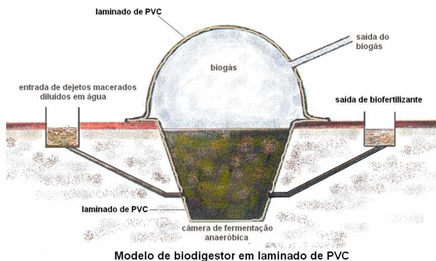
Figura 8-Modelo de biodigestor canadense. Fonte: WINROCK, 2008
