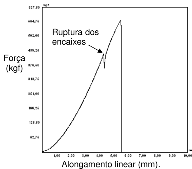
Figura 43: Exemplo de curva típica de força versus alongamento de um corpo de prova típico das juntas coladas encaixadas de Angelim-pedra.
