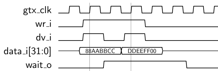
Figura 31: Diagrama de tempo da UDPIPv2 - Pacotes da aplicação para o core UDP/IP.
