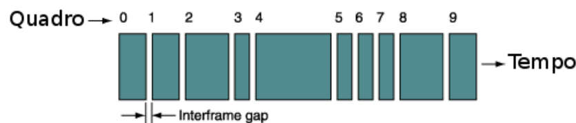
Figura 10: Exemplo de InterFrame Gap .
