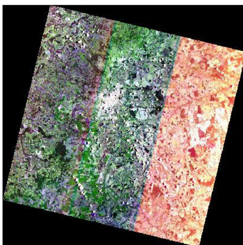
583 584 Figura 25 - Bandeamento. Composição 123, imagem de 04/02/2008, do satélite 585 CBERS-2B.
