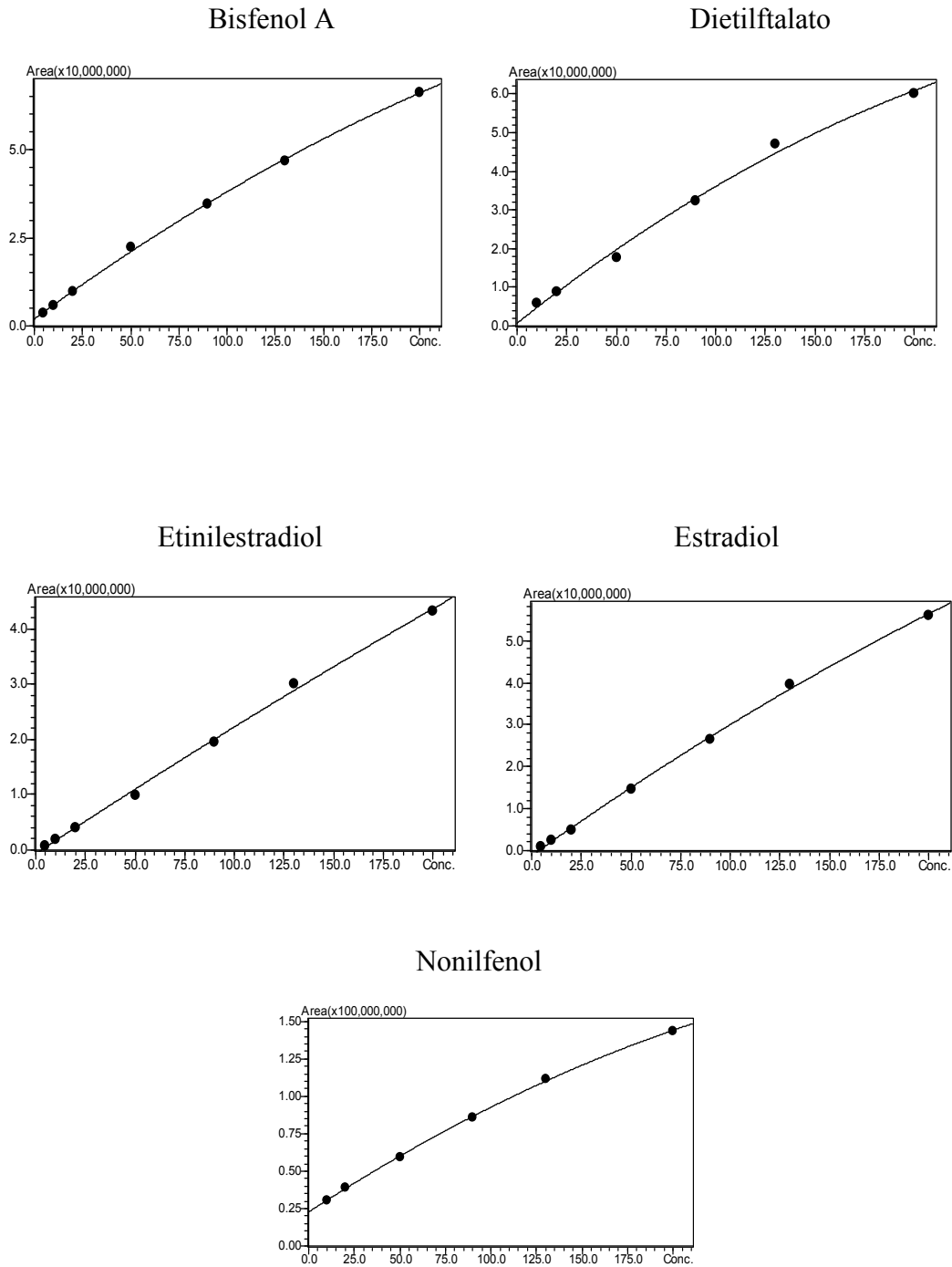
Figura 5. 5: Curvas analíticas dos compostos estudados
