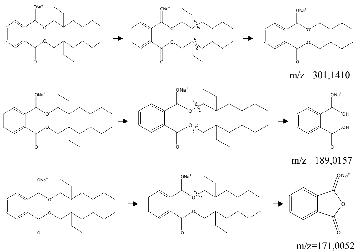
Figura 7. 3: Mecanismo de fragmentação propostos para o bis etil(hexil)ftalato
