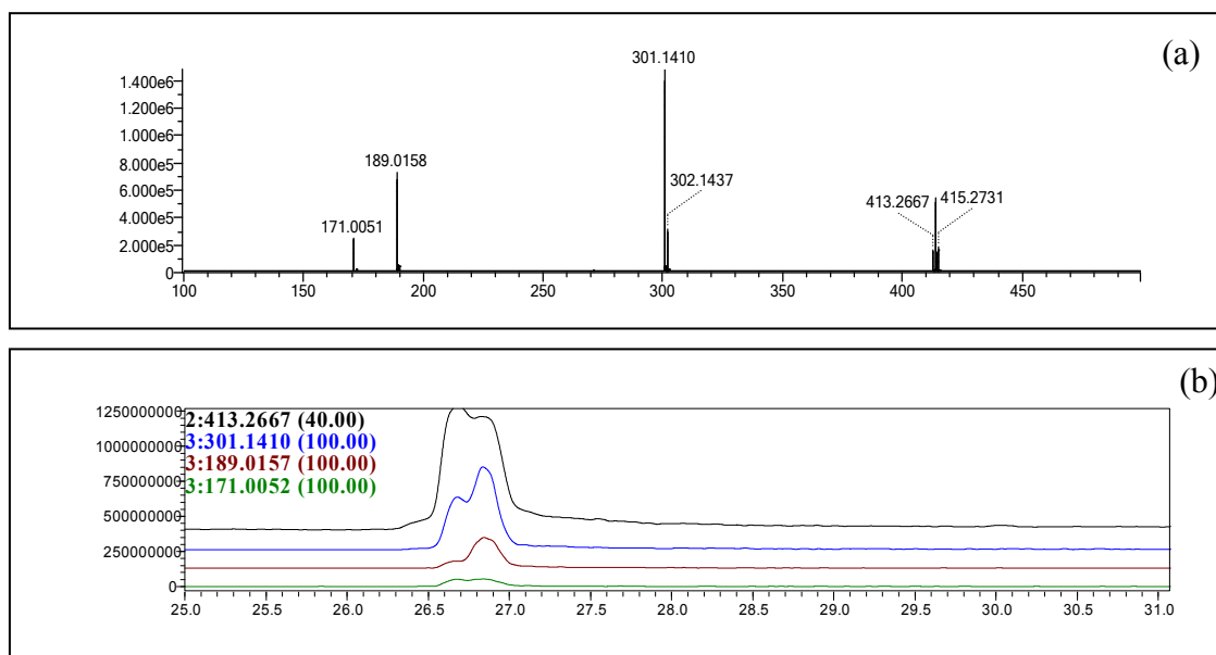
Figura 7. 2: (a) espectro de massas MS^2 obtido para fragmentação do íon m/z=413,2667 ; (b) cromatograma obtido para fragmentação do íon m/z=413,2667
