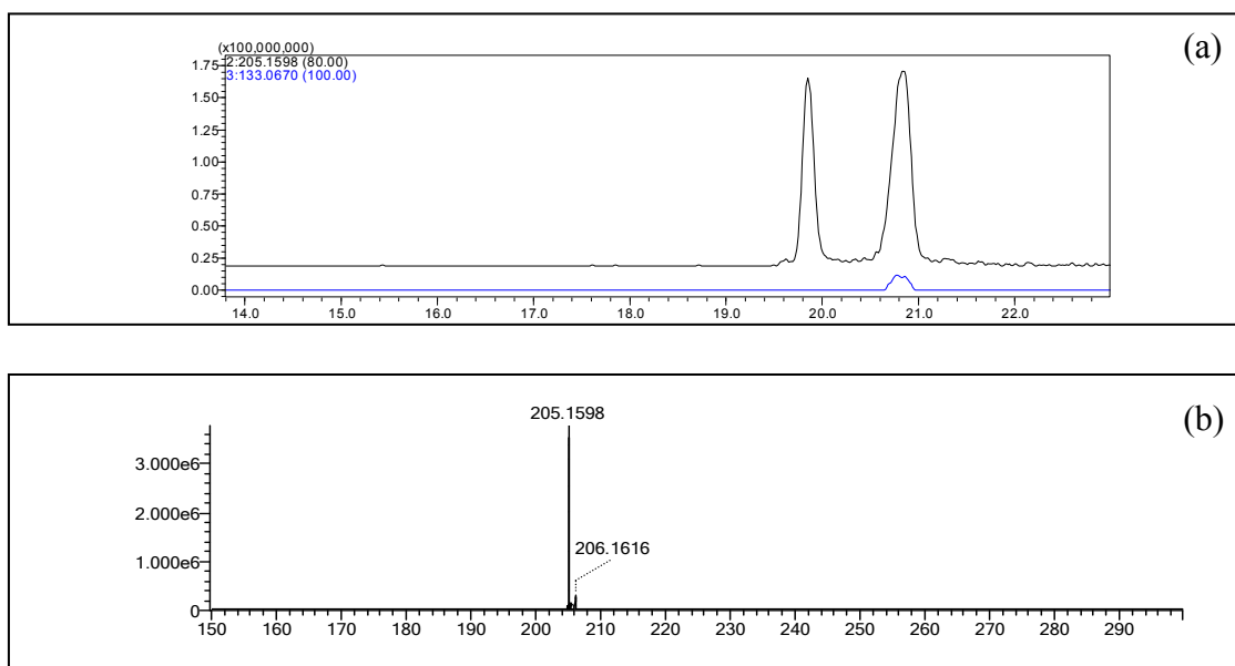
Figura 7. 7: (a) Cromatograma do íon medido m/z=205,1598 ; (b) Espectro de massas obtido do íon m/z=205,1598
