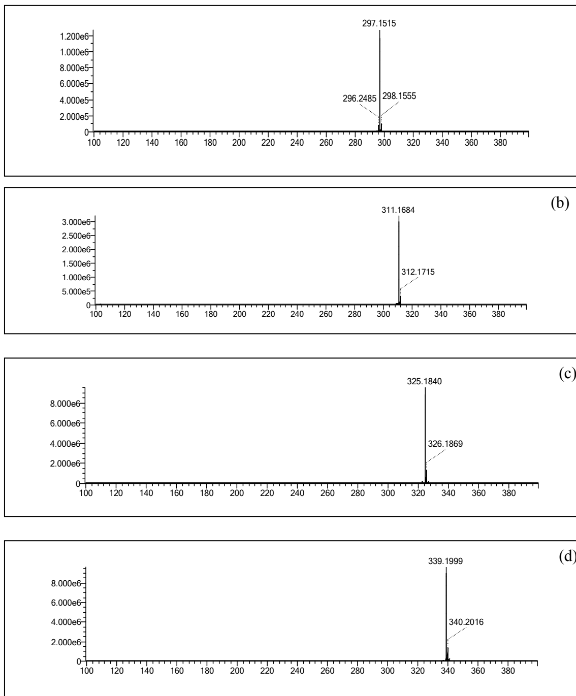
Figura 7. 11: (a), (b), (c) e (d) Espectros de massas obtidos para os íons m/z=297,1515 , m/z=311,1684 , m/z=325,1840 e m/z=339,1999
