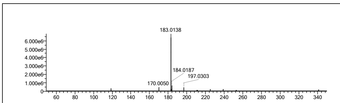
Figura 7. 13: (a), (b), (c) e (d): Espectros de massas MS^2 obtidos na fragmentação dos íons m/z=297,1515 , m/z=311,1684 , m/z=325,1840 e m/z=339,1999
