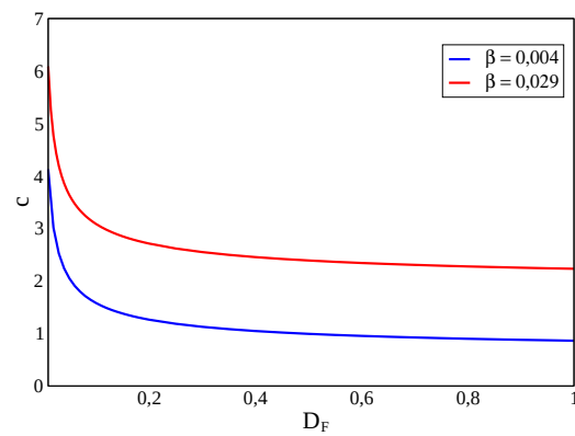
Figura 20: Relação entre a velocidade c de onda viajante e o parâmetro D_F .
