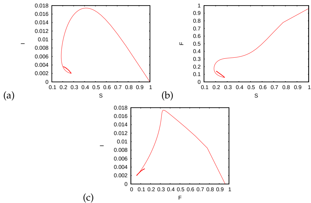
Figura 11: Os diagramas de fase entre (a) caranguejos susceptíveis S e infectados I , (b) caranguejos susceptíveis S e fungos F e (c) caranguejos infectados I e fungos F para \beta = 0,004 , v_F = 0,2 \text{ Km dia}^{-1} , R_C = 1,49 e R_F = 1,60 .
