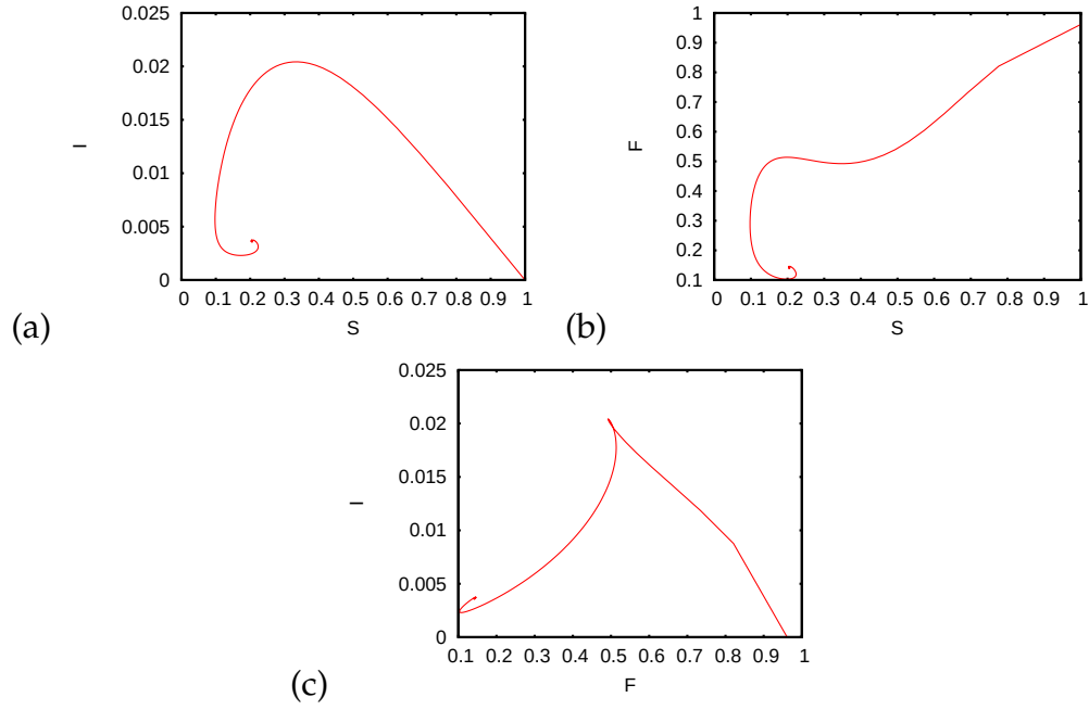
Figura 9: Os diagramas de fase entre (a) caranguejos susceptíveis S e infectados I , (b) caranguejos susceptíveis S e fungos F e (c) caranguejos infectados I e fungos F para \beta = 0,004 , v_F = 0,0 \text{ Km dia}^{-1} , R_C = 1,49 e R_F = 1,60 .
