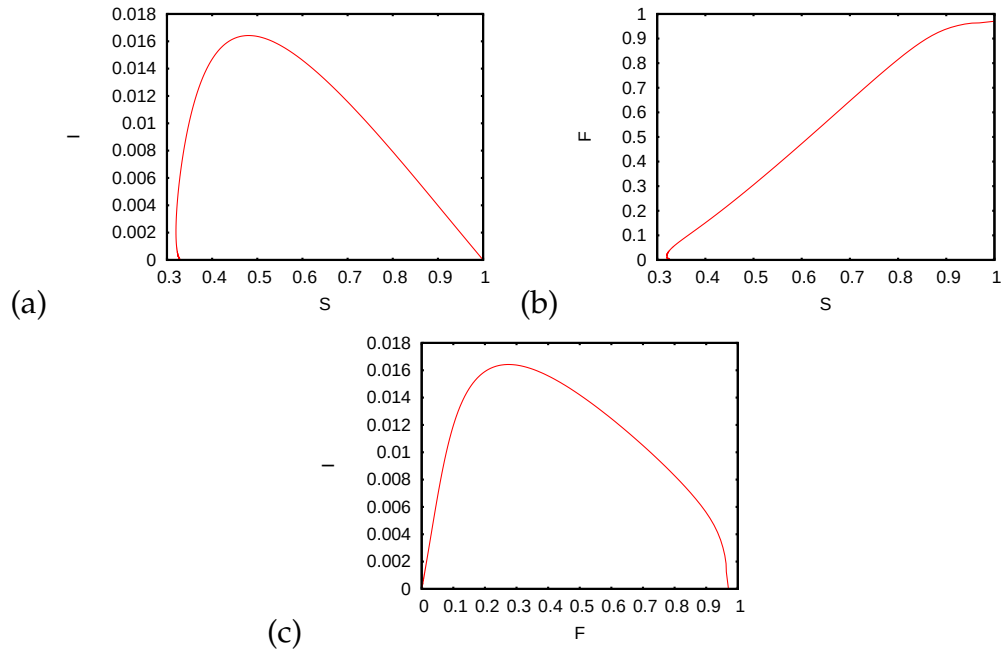
Figura 7: Os diagramas de fase entre (a) caranguejos susceptíveis S e infectados I , (b) caranguejos susceptíveis S e fungos F e (c) caranguejos infectados I e fungos F para \beta = 0,001 , v_F = 0,2 \text{ Km dia}^{-1} , R_C = 1,49 e R_F = 0,40 .
