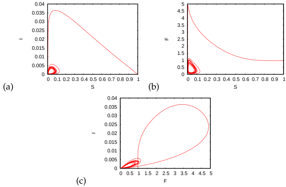
Figura 15: Os diagramas de fase entre (a) caranguejos susceptíveis S e infectados I , (b) caranguejos susceptíveis S e fungos F e (c) caranguejos infectados I e fungos F para \beta = 0,029 , \nu_F = 0,2 \text{ Km dia}^{-1} , R_C = 1,49 e R_F = 11,61 .
