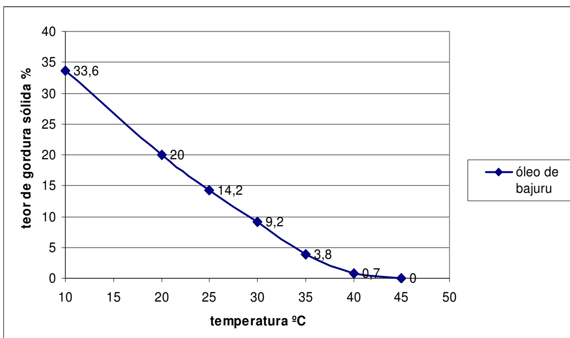
Gráfico 7 – Curva de Sólidos do óleo bruto da semente do bajúru
