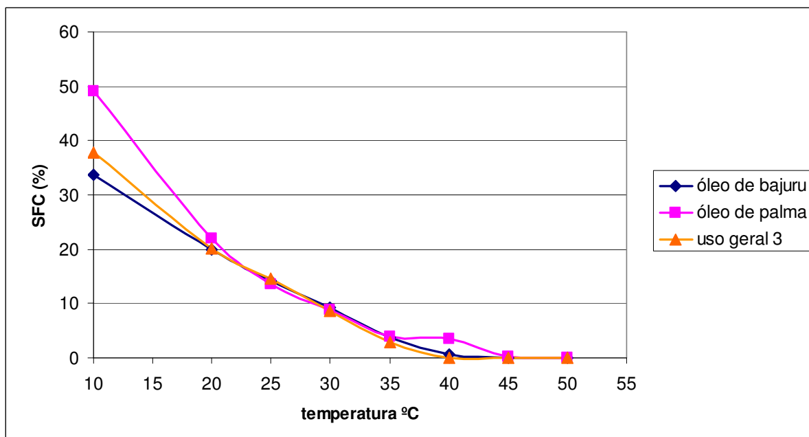
Gráfico 8- Comparação da curva do conteúdo de gordura sólida para diferentes tipos de gorduras.
