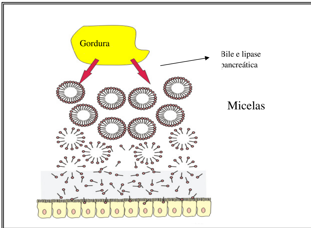
Figura 12- Esquema da formação das micelas pela ação da bile e lípase pancreática ( Fonte: www.en.witibooks.org/digestion_&_Absorption )
