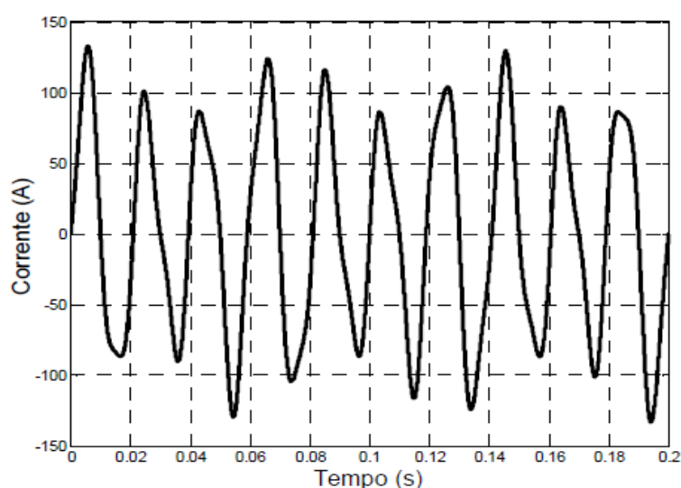
Figura 3.5.3. - Forma de onda com distorções inter-harmônicas.
