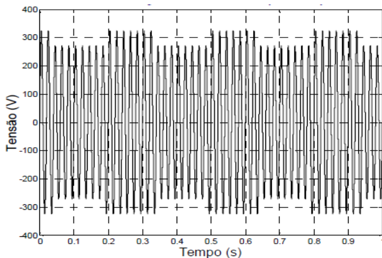
Figura 3.6. - Forma de onda com a presença de flutuação de tensão.
