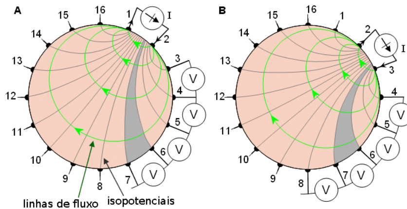
Figura 2.6: O método da vizinhança aplicado a um domínio de seção circular. São apresentados 2 casos de solitação e 4 medidas de diferença de potencial para cada caso. A imagem foi adaptada de [58].
