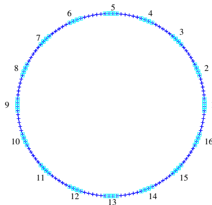
Figura 4.1: Domínio circular e distribuição dos 16 eletrodos no contorno externo.
