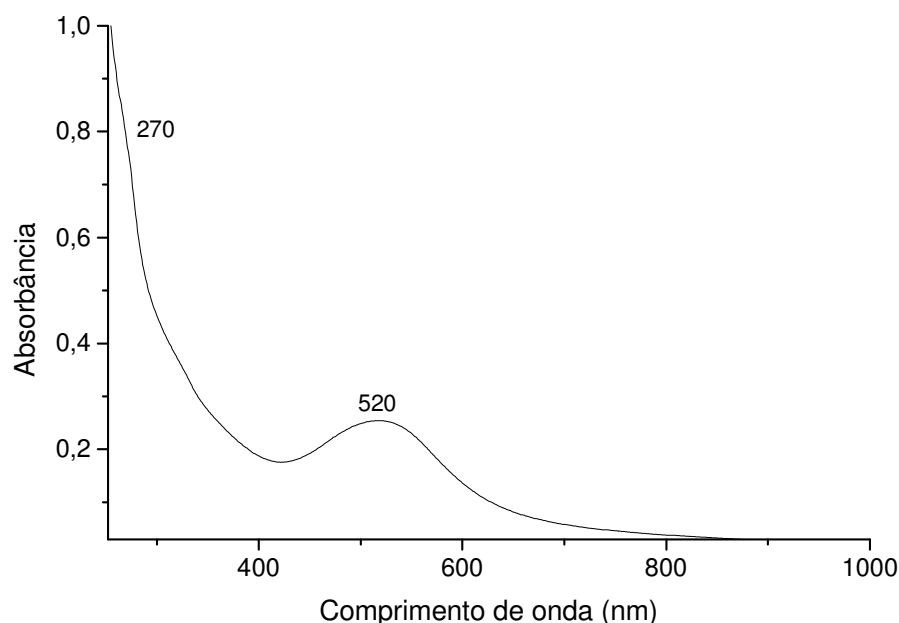
Figura 33 - Espectro eletrônico do complexo cis -[Ru II Cl 2 (dppb)(bqdi)], 7,8 \times 10^{-5} \text{ mol} \cdot \text{L}^{-1} , em solução de CH 2 Cl 2 .
