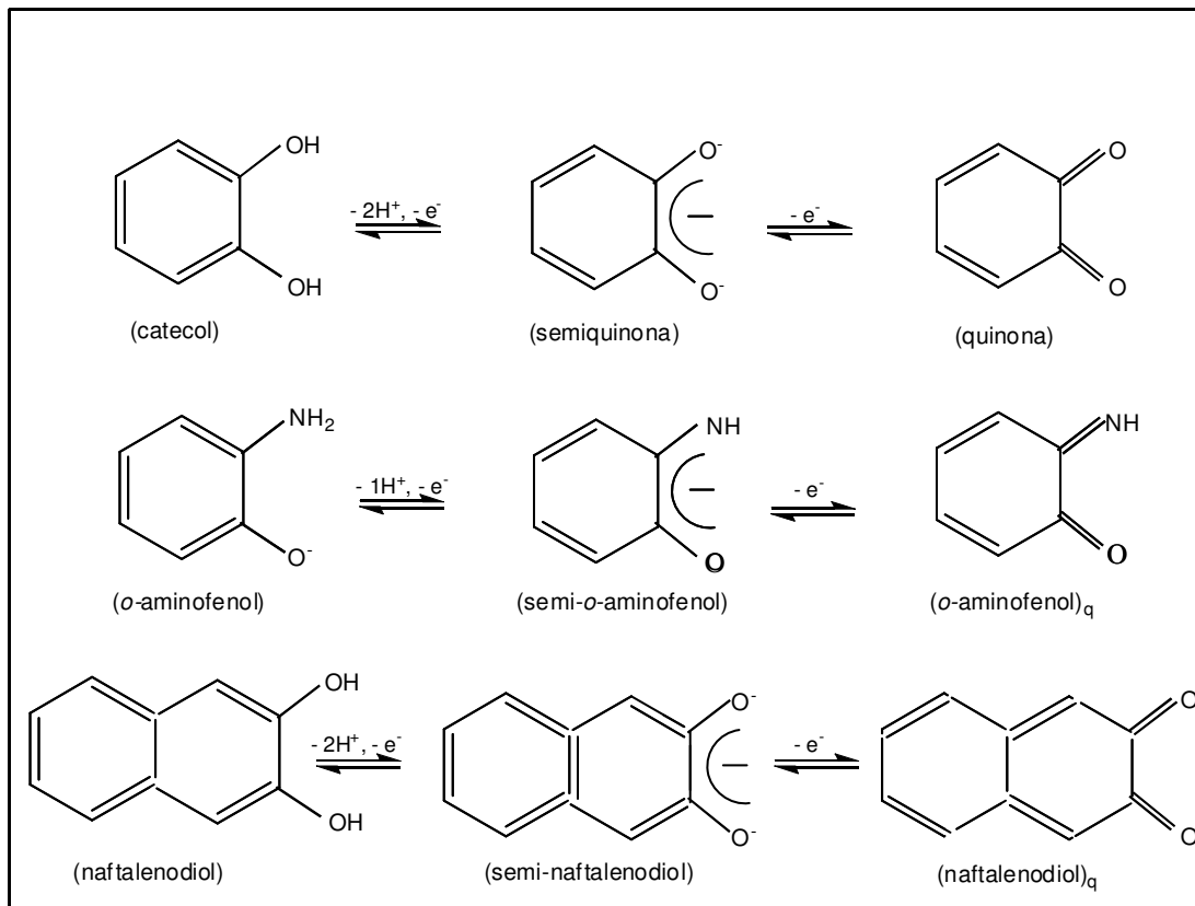
Figura 2 - Isômeros redox dos ligantes catecol, o -aminofenol e naftalenodiol. Adaptada da referência [16].
