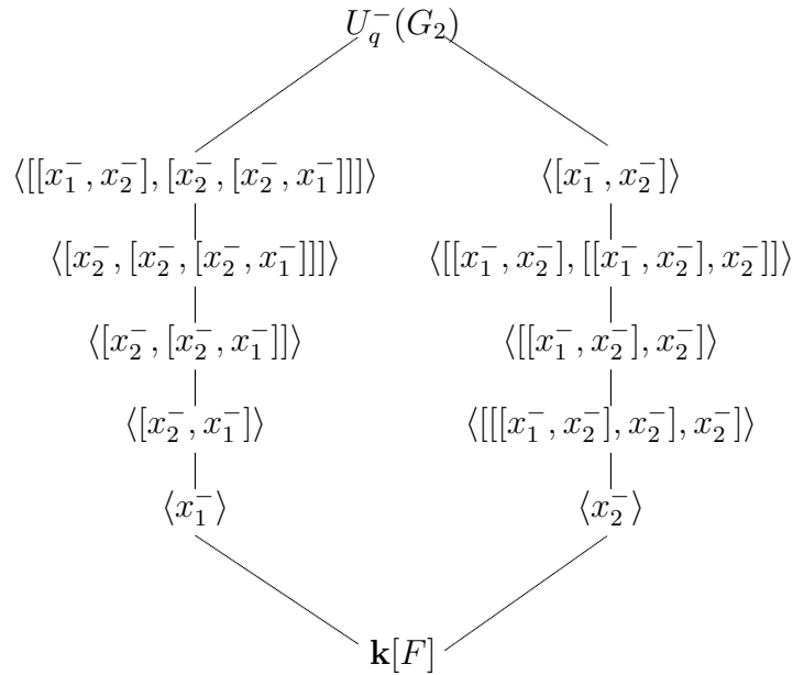
Figura 4.1: Reticulado de Subálgebras Coideais à Direita
