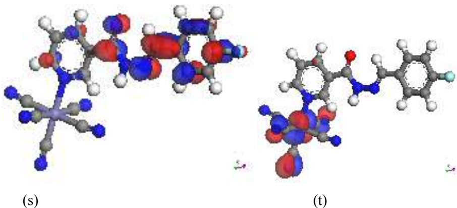
Figura 115. Orbitais de fronteira para os complexos; Orbitais LUMO para estruturas otimizadas do tipo [\text{Fe}(\text{CN})_5\text{L}]^{3-} , onde \text{L} = (a) \text{IO}_3\text{H} ; (c) \text{IO}_3\text{S} ; (e) \text{IO}_3\text{Met} ; (g) \text{IO}_3\text{SMet} ; (i) \text{IA}_4\text{H} ; (k) \text{IA}_4\text{OMet} ; (m) \text{IA}_4\text{F} ; (o) \text{NA}_4\text{H} ; (q) \text{NA}_4\text{OMet} ; (s) \text{NA}_4\text{F} . Orbitais HOMO-2; (b) \text{IO}_3\text{H} ; (d) \text{IO}_3\text{S} ; (f) \text{IO}_3\text{Met} ; (h) \text{IO}_3\text{SMet} ; Orbitais HOMO-1; (j) \text{IA}_4\text{H} ; (l) \text{IA}_4\text{OMet} ; (n) \text{IA}_4\text{F} ; (p) \text{NA}_4\text{H} ; (r) \text{NA}_4\text{OMet} ; (t) \text{NA}_4\text{F} .
