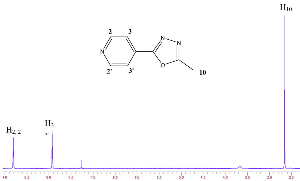
Figura 28. Espectro de RMN 1 H para o composto IO3Met, em CDCl 3 , 500MHz.
