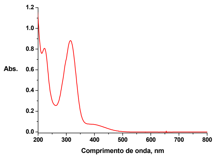
Figura 71. Espectro eletrônico em meio aquoso do íon complexo [\text{Fe}(\text{CN})_5(\text{NA4OMet})]^{3-} pH = 6,8.
