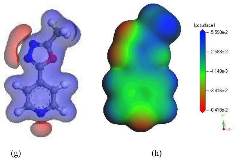
Figura 113. Estrutura otimizada contornada pelo potencial eletrostático para os ligantes oxadiazóis e sua densidade eletrônica molecular total com gradiente de potencial eletrostático. Estruturas otimizadas: (a) IO3S; (c) IO3H; (e) IO3SMet; (g) IO3Met. Gradiente de potencial eletrostático: (b) IO3S; (d) IO3H; (f) IO3SMet; (h) IO3Met.
