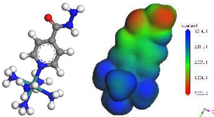
(a) (b) Figura 118. (a) Estrutura otimizada do complexo pentaamin(isoniazida)rutenado (II) (b) Densidade eletrônica molecular total com gradiente de potencial eletrostático do complexo pentaamin(isoniazida)rutenado (II).
