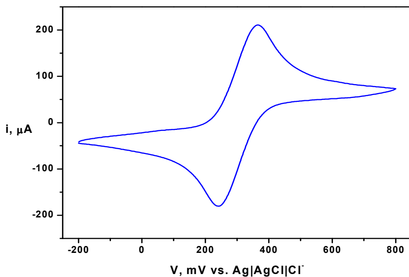
Figura 108. Voltamograma cíclico do eletrodo de carbono vítreo em solução aquosa (NaTFA 0,1 \text{ mol.L}^{-1} , pH = 6,8) contendo o íon complexo [\text{Fe}(\text{CN})_5(\text{IO3Met})]^{3-} , v = 100\text{mV/s} .
