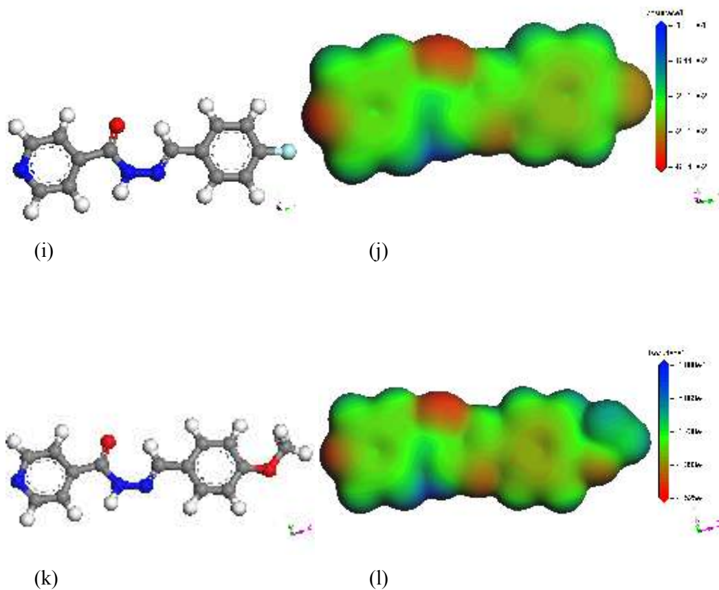
Figura 112. Estrutura otimizada para os ligantes hidrazonas e sua densidade eletrônica molecular total com gradiente de potencial eletrostático. Estruturas otimizadas: (a) NA4H; (c) NA4F; (e) NA4OMet; (g) IA4H; (i) IA4F; (k) IA4OMet. Gradiente de potencial eletrostático: (b) NA4H; (d) NA4F; (f) NA4OMet; (h) IA4H; (j) IA4F; (l) IA4OMet
