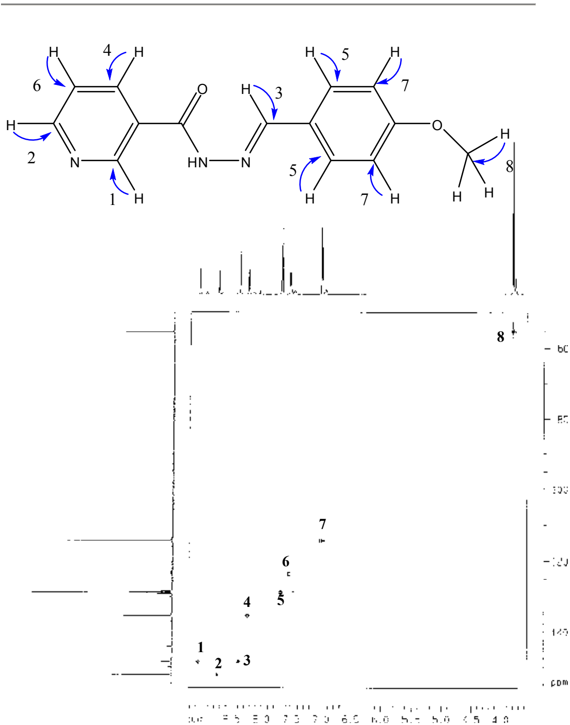
Figura 22. Diagrama de contorno de RMN bidimensional de correlação heteronuclear para o íon complexo NA4OMet, em DMSO, 500MHz.
