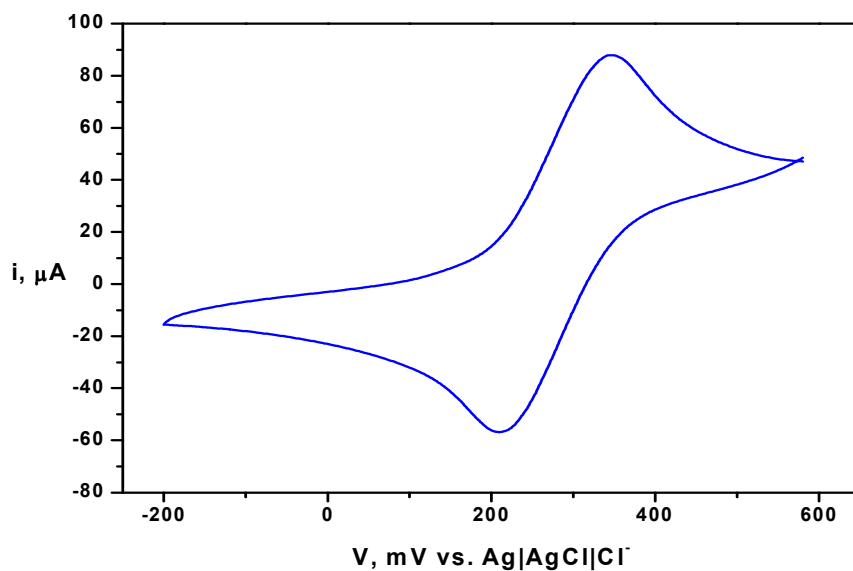
Figura 109. Voltamograma cíclico do eletrodo de carbono vítreo em solução aquosa (NaTFA 0,1 \text{ mol.L}^{-1} , pH = 6,8) contendo o íon complexo [\text{Fe}(\text{CN})_5(\text{IO3S})]^{3-} , v = 100\text{mV/s} .
