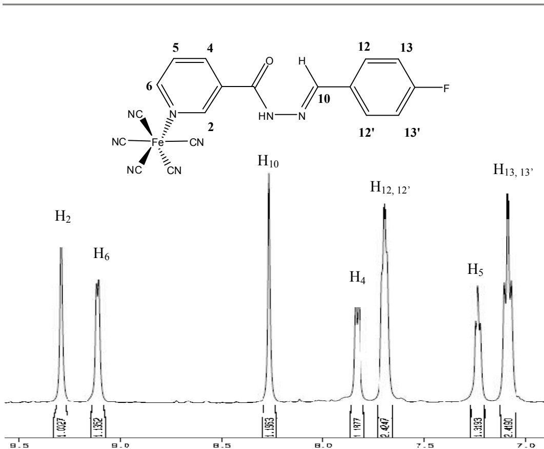
Figura 40. Espectro de RMN ^1\text{H} para o composto [\text{Fe}(\text{CN})_5(\text{NA4F})]^{3-} , em \text{D}_2\text{O} , 500 MHz.
