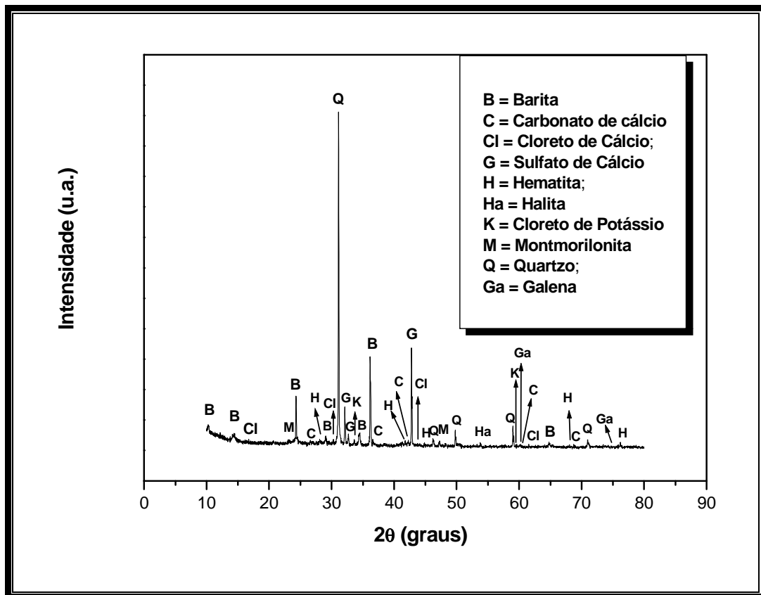
Figura 4.4 – Difratograma de raios-X do resíduo borra de petróleo encapsulada.
