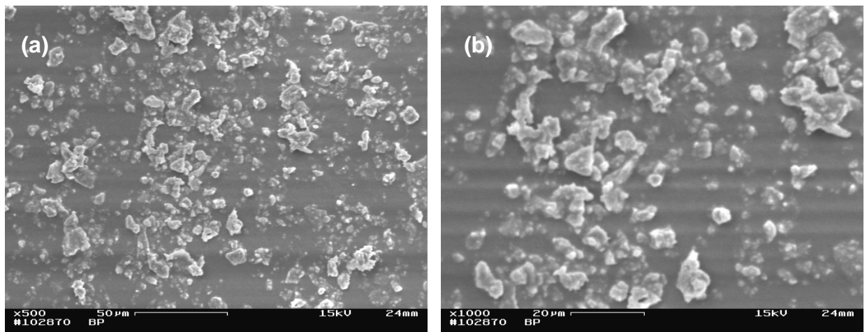
Figura 4.12 – Morfologia das partículas do resíduo borra de petróleo encapsulada. (a) 500x; (b) 1000x.
