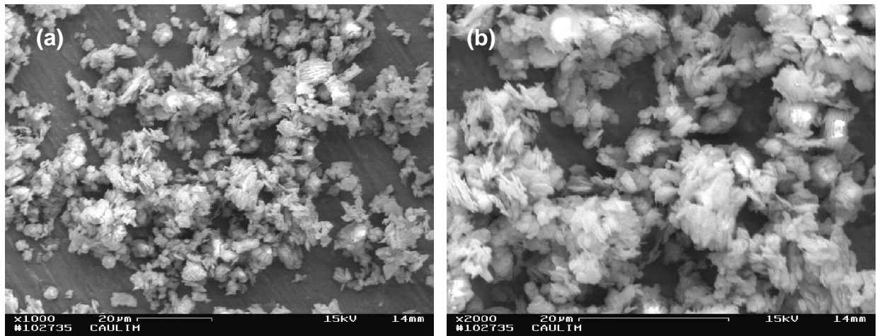
Figura 4.9 – Morfologia das partículas de caulim. (a) 1000x; (b) 2000x.
