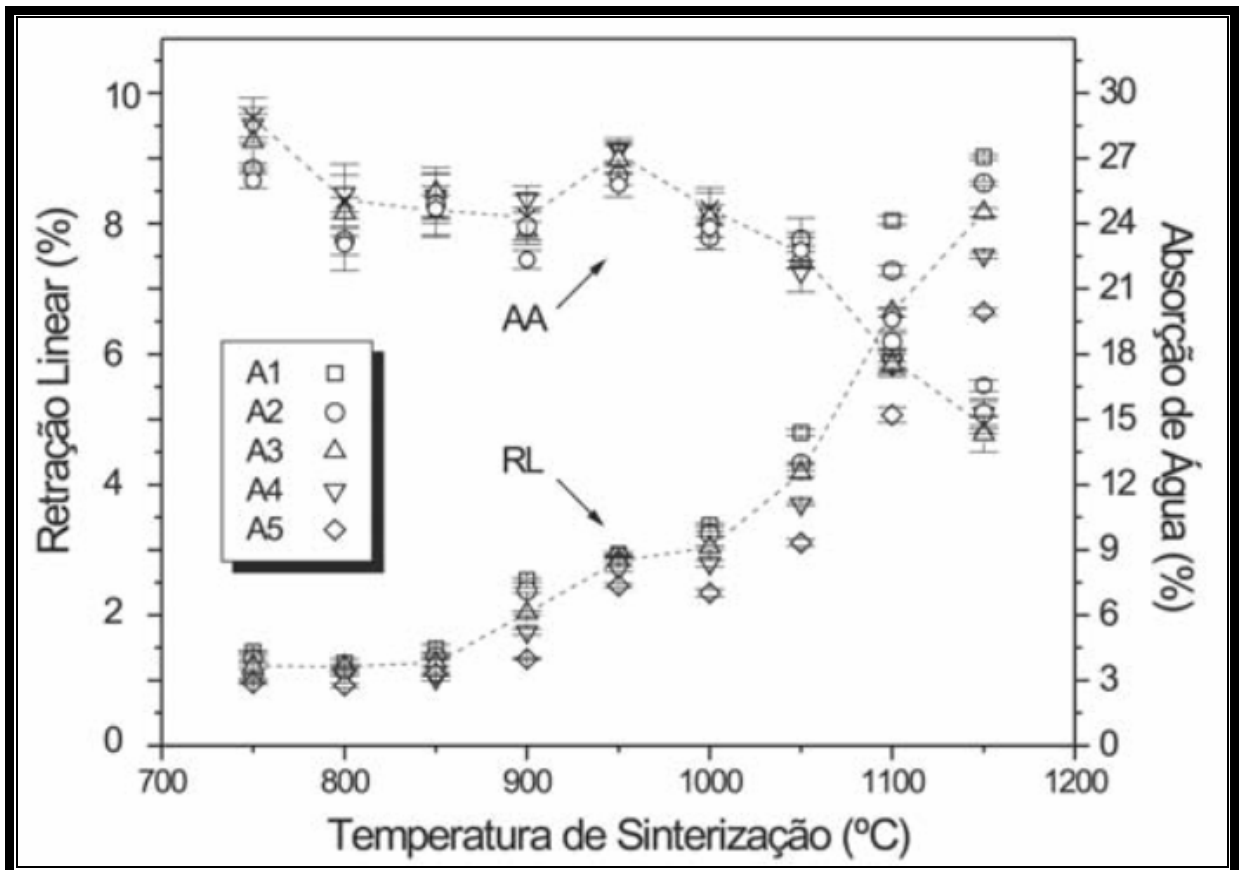
Figura 2.15 – Diagrama de gresificação das massas cerâmicas contendo resíduo (Souza et al. 2003).
