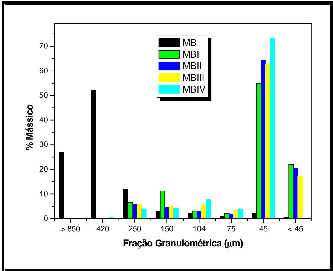
Figura 4.27 – Distribuição de tamanho dos grânulos para as massas cerâmicas granuladas pelo processo via seca.
