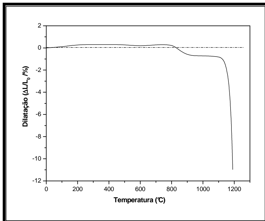
Figura 4.8 – Curva dilatométrica do resíduo borra de petróleo encapsulada.
