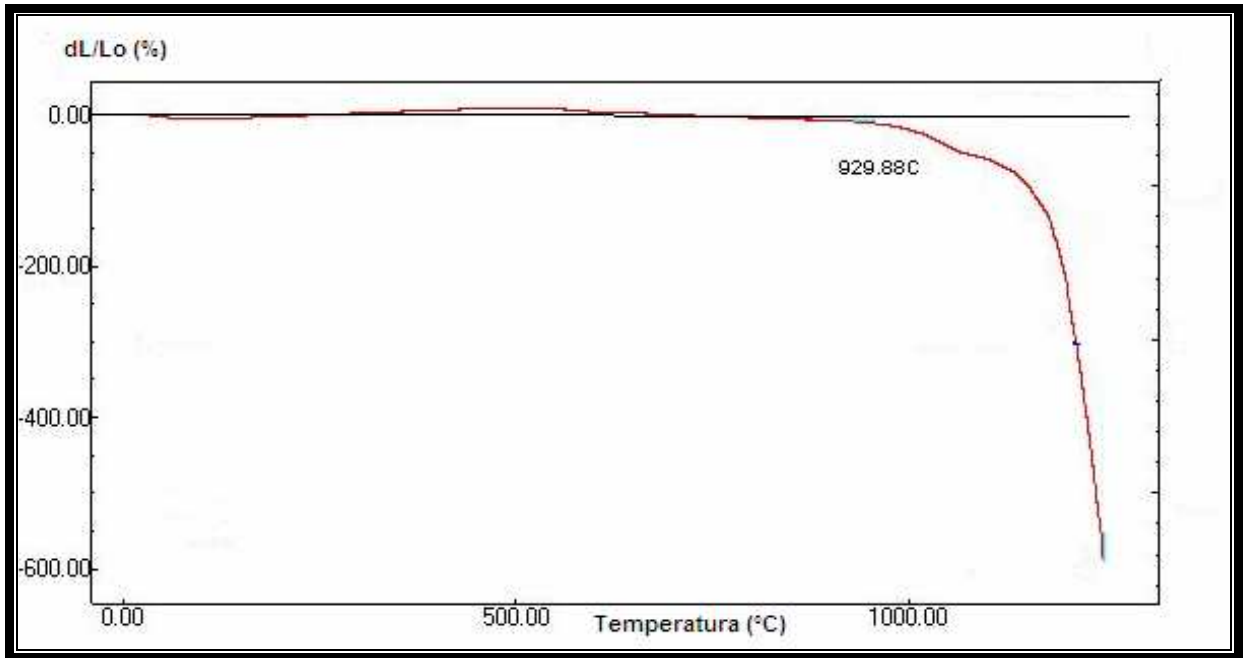
Figura 4.25 – Curva dilatométrica para a massa cerâmica MBIII.
