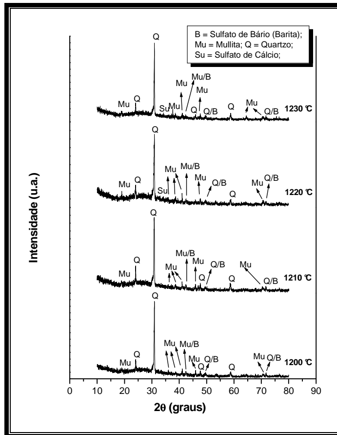
Figura 4.37 – Difratoograma de raios-X para a massa cerâmica MBIV.
