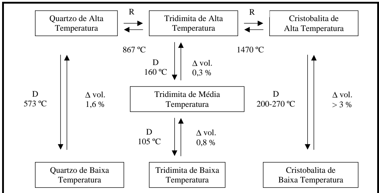
Figura 2.3 - Transformações polimórficas deslocativas (D) e reconstrutivas (R), e mudanças de volume da sílica (Richerson, 1992).
