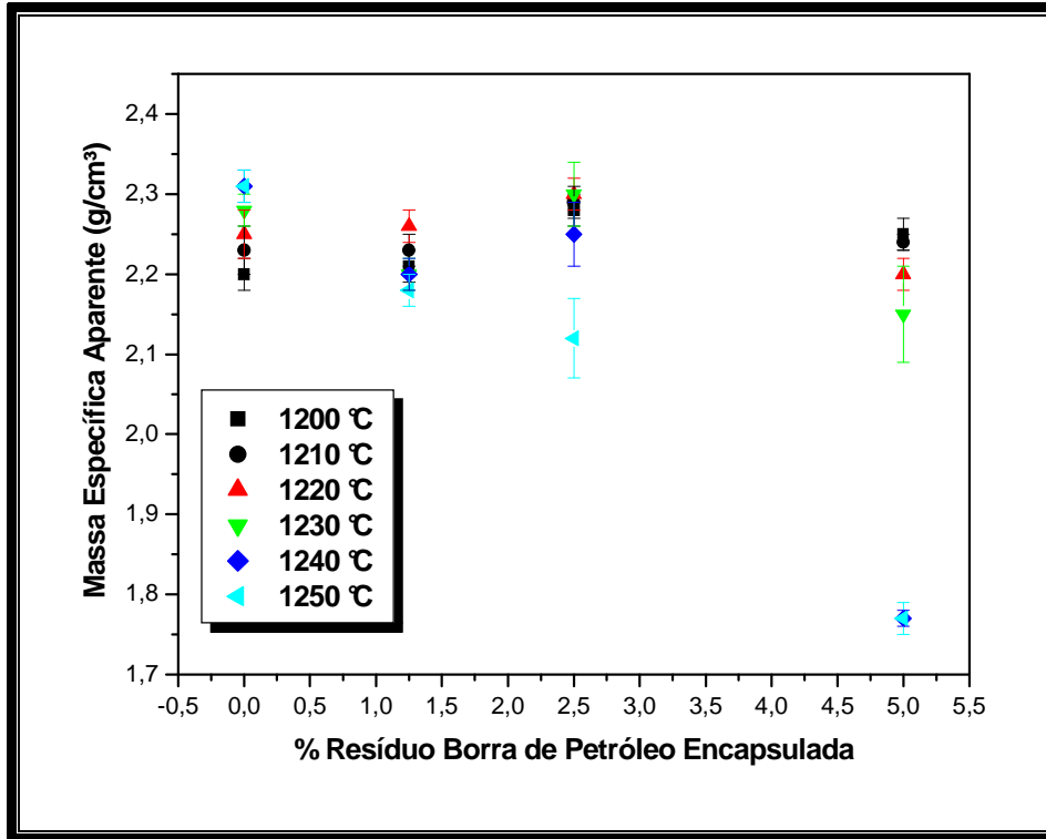
Figura 4.62 – Massa específica aparente em função da adição de resíduo borra de petróleo encapsulada.
