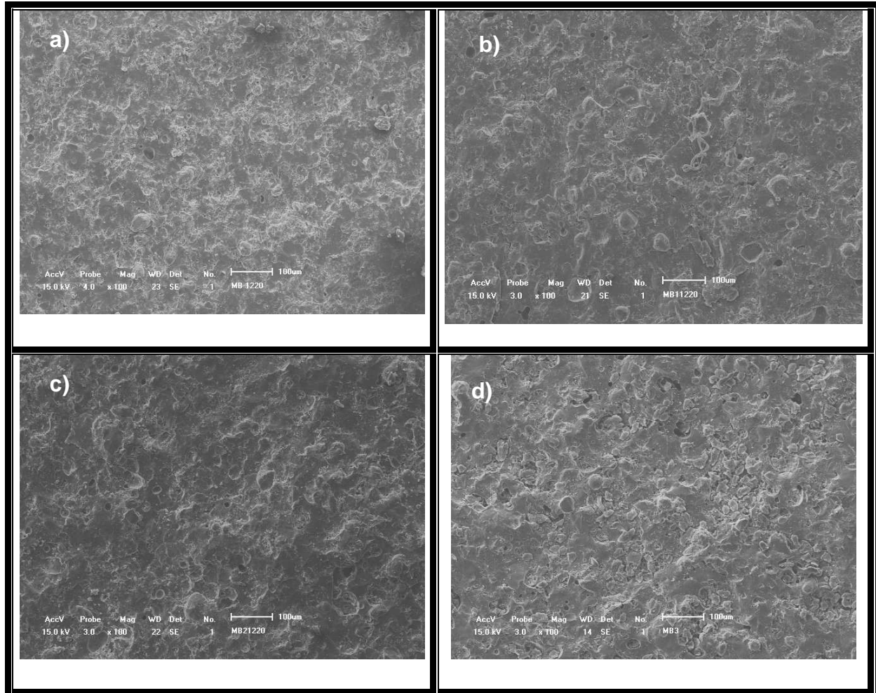
Figura 4.44 – Microestrutura das peças cerâmicas sinterizadas em 1220 °C.
