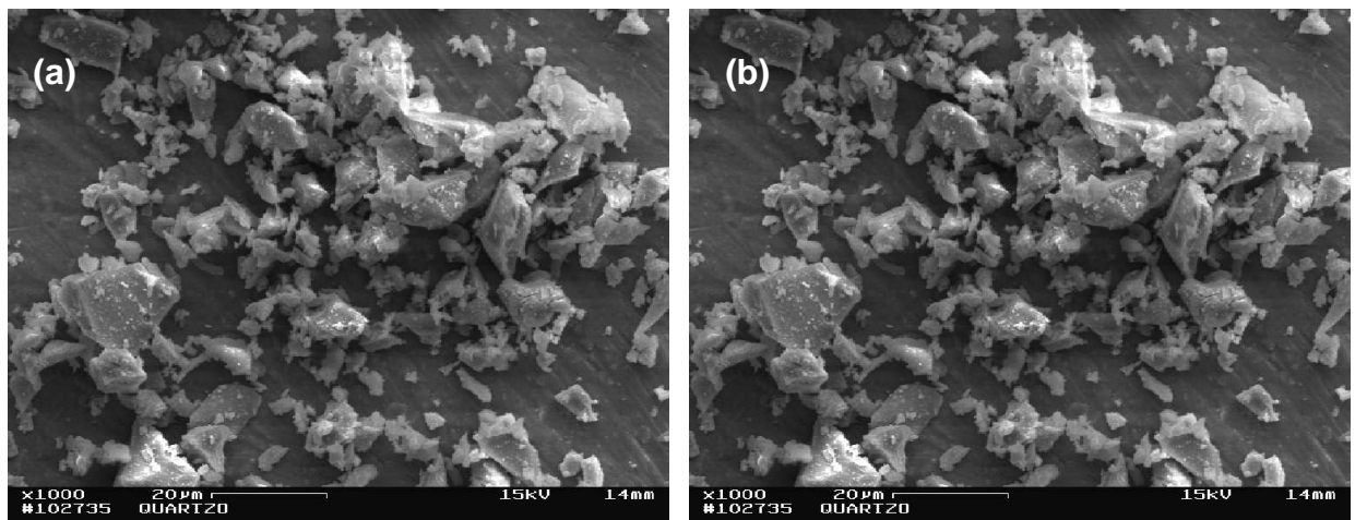
Figura 4.11 – Morfologia das partículas de quartzo (a) 1000x; (b) 2000x.
