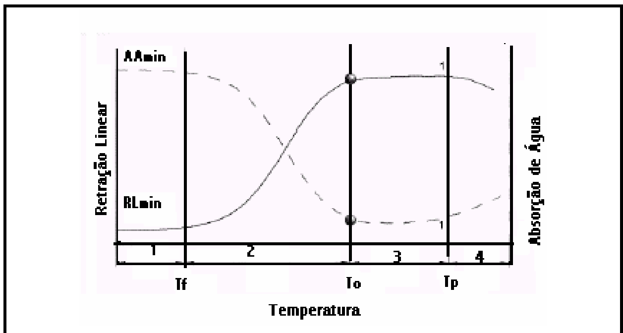
Figura 2.7 – Curva de gresificação para massa ideal de grês porcelanato (Sanchez-Munõz et. al., 2002).
