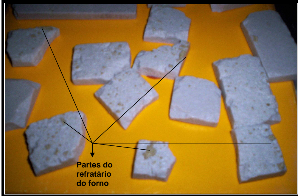
Figura 4.53 – Partes do suporte refratário do forno grudadas nas peças cerâmicas (massa cerâmica MBIV).
