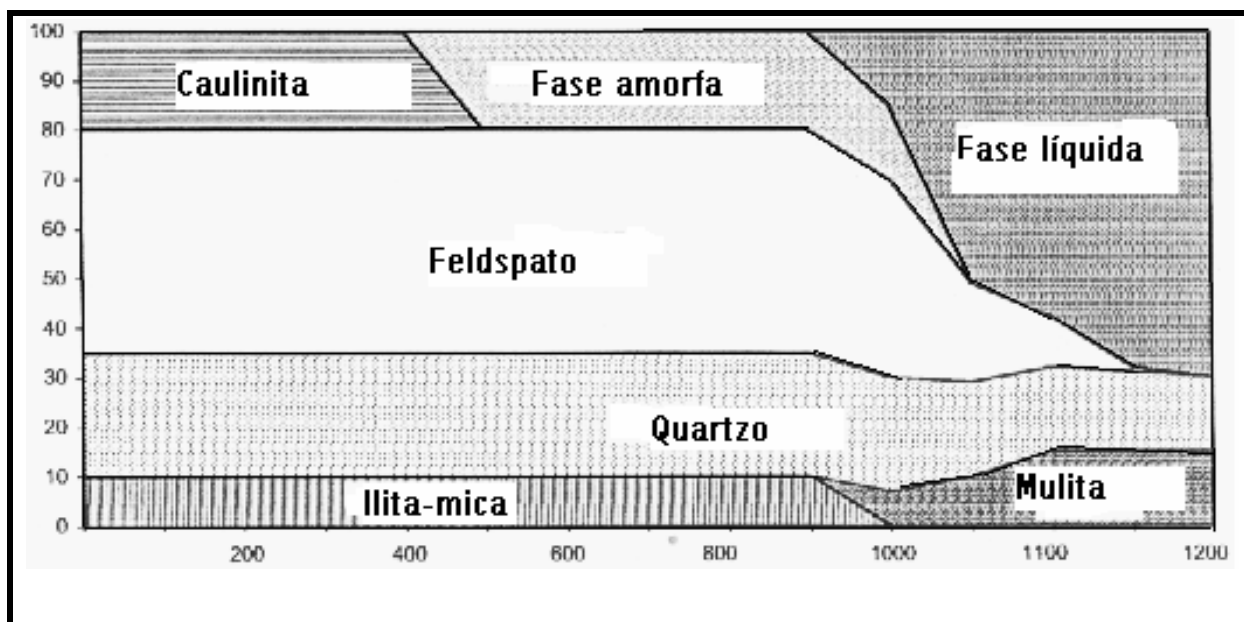
Figura 2.5 – Esquema das transformações de fases que ocorrem durante sinterização do grês porcelanato (Zanelli et. al., 2003).
