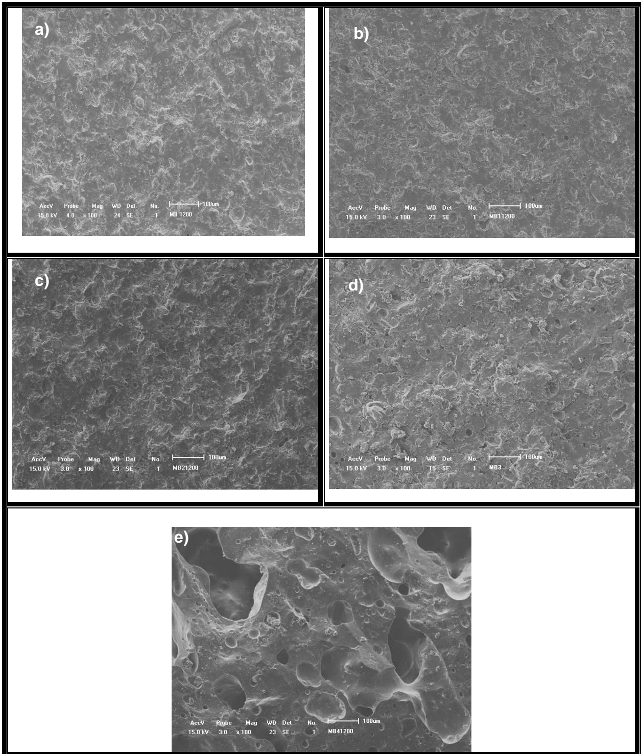
Figura 4.42 – Microestrutura das peças cerâmicas sinterizadas em 1200 °C.
