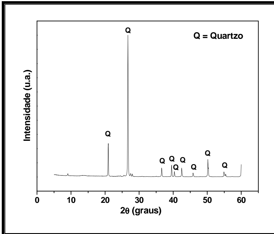
Figura 4.2 – Difratoograma de raios-X do quartzo utilizado.
