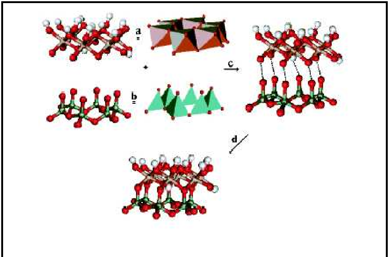
Figura 2.1- Estrutura da Gibsita (a), Sílica (b), O Processo de Montagem da Estrutura Ideal da Caulinita (c) e a Estrutura Final da Caulinita (d). (Gardolinski et. al., 2003).
