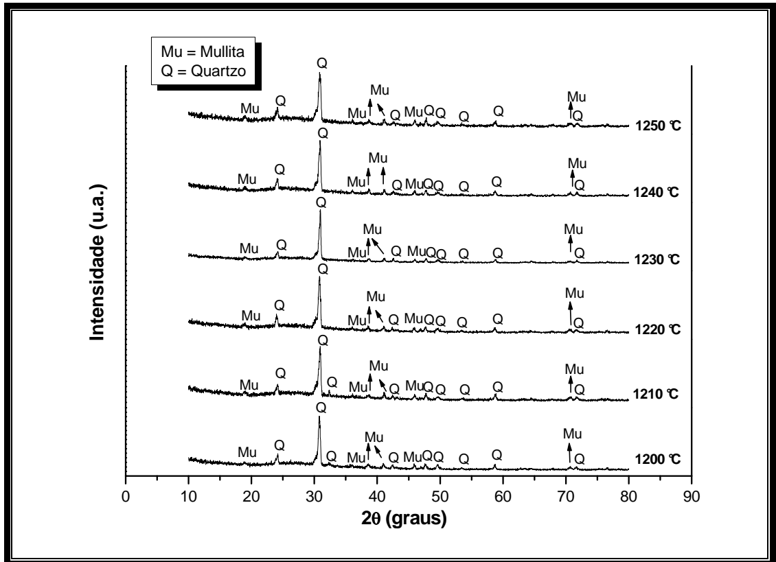
Figura 4.33 – Difratoograma de raios-X para a massa cerâmica MB.
