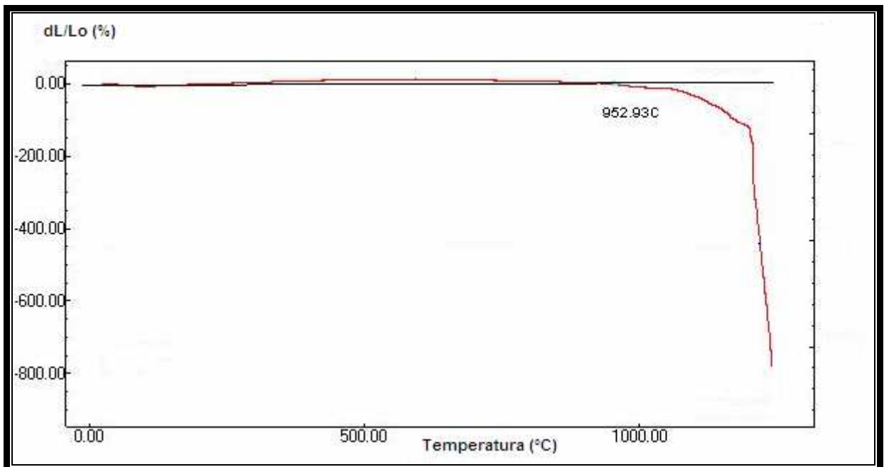
Figura 4.26 – Curva dilatométrica para a massa cerâmica MBIV.
