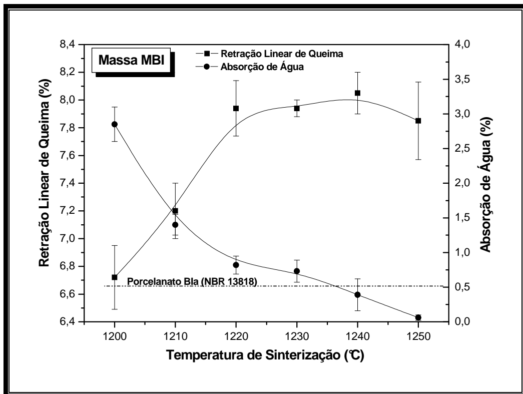
Figura 4.49 – Curva de gresificação para a massa cerâmica MBI.
