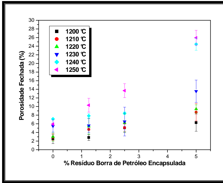
Figura 4.55 – Porosidade fechada em função da adição de resíduo borra de petróleo encapsulada.
