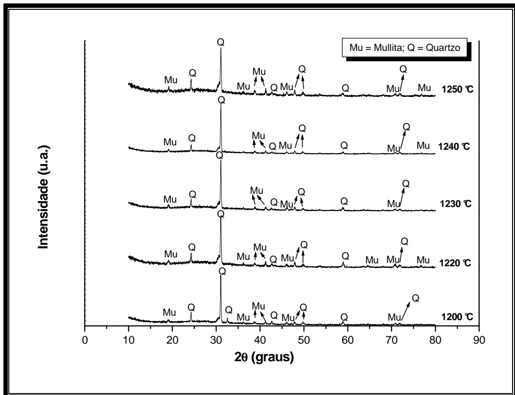
Figura 4.34 – Difratoograma de raios-X para a massa cerâmica MBI.
