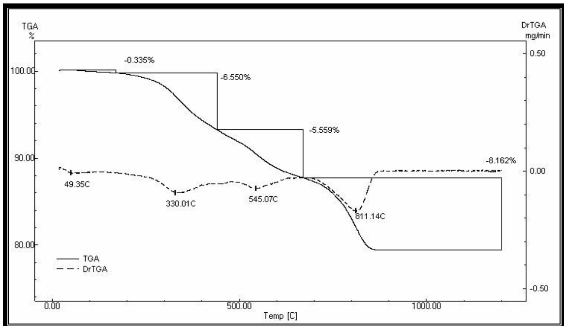
Figura 4.7 – Curvas TGA e DrTGA do resíduo borra de petróleo encapsulada.
