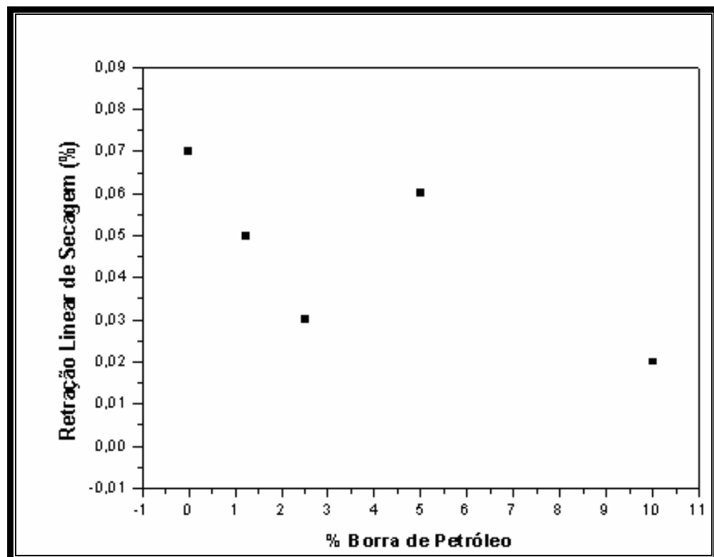
Figura 4.30 – Retração linear de secagem em função da adição de resíduo borra de petróleo encapsulada.
