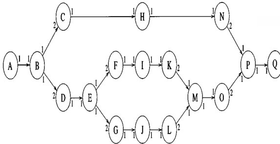
Figura 2.1: Modelo de algoritmo utilizando SDF [BHA 00].
