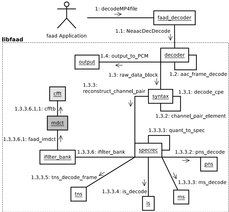
Figura 4.2: Visão geral dos módulos e funções do FAAD2 executadas na decodificação de arquivos AAC LC
