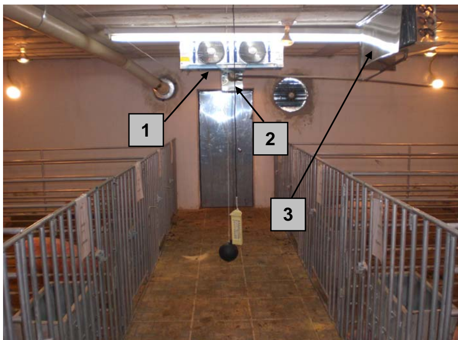
FIGURA 5. Fotos da sala climatizada (1-Aquecedor e refrigerador; 2- umidificador e 3 - Desumidificador)
