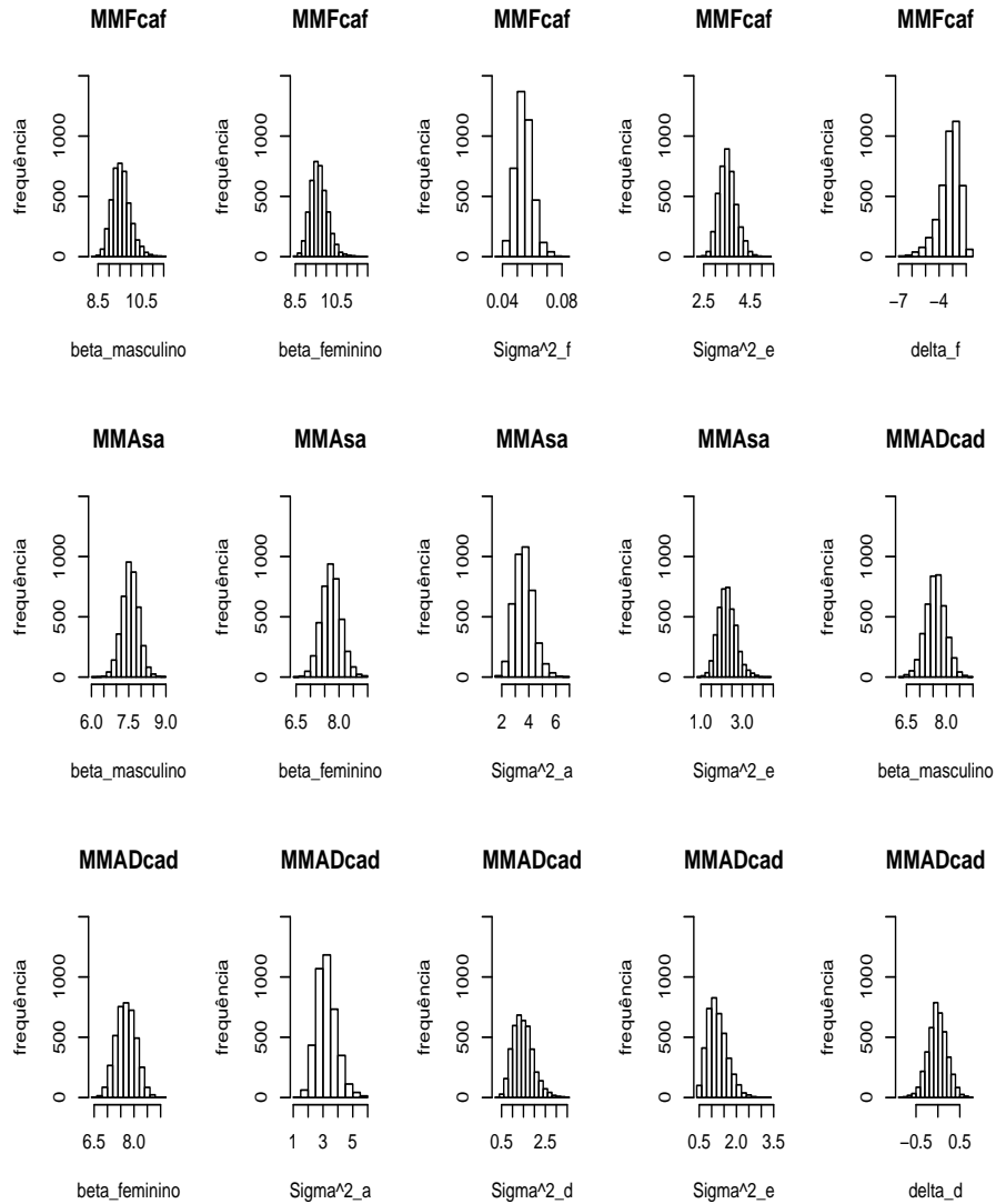
FIGURA 17 Histogramas das amostras a posteriori dos parâmetros \beta (sexo), \sigma^2 (variância) e \delta (assimetria, caso seja suposta no modelo) para os três melhores modelos através do FB, relativos às 16 configurações consideradas para a sonda 1950.
