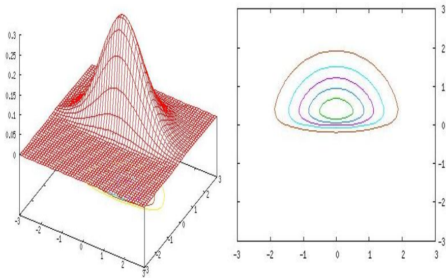
FIGURA 5 Distribuição SN_2((0,0)^T, \text{diag}(1,1), \text{diag}(0,5)) com seu gráfico de contorno.
