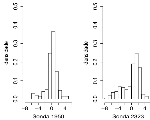
FIGURA 14 Histogramas para os resíduos do ajuste do modelo misto usual para as sondas 1950 e 2323, respectivamente.
