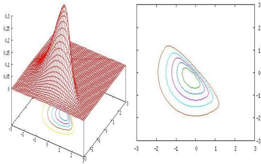
FIGURA 6 Distribuição SN_2((0,0)^\top, \text{diag}(1,1), \text{diag}(-5, -5)) com seu gráfico de contorno.
