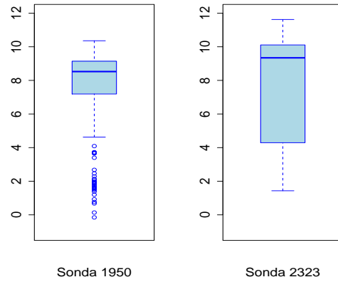
FIGURA 13 Desenhos esquemáticos dos valores observados das intensidades das expressões para as sondas 1950 e 2323, respectivamente.
