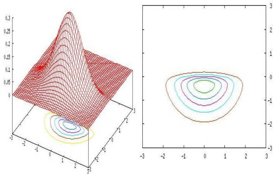
FIGURA 4 Distribuição SN_2((0,0)^T, \text{diag}(1,1), \text{diag}(0,-5)) com seu gráfico de contorno.
