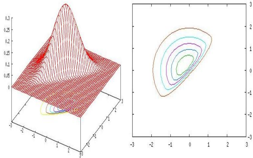
FIGURA 8 Distribuição SN_2((0,0)^\top, \text{diag}(1,1), \text{diag}(-5,5)) com seu gráfico de contorno.
