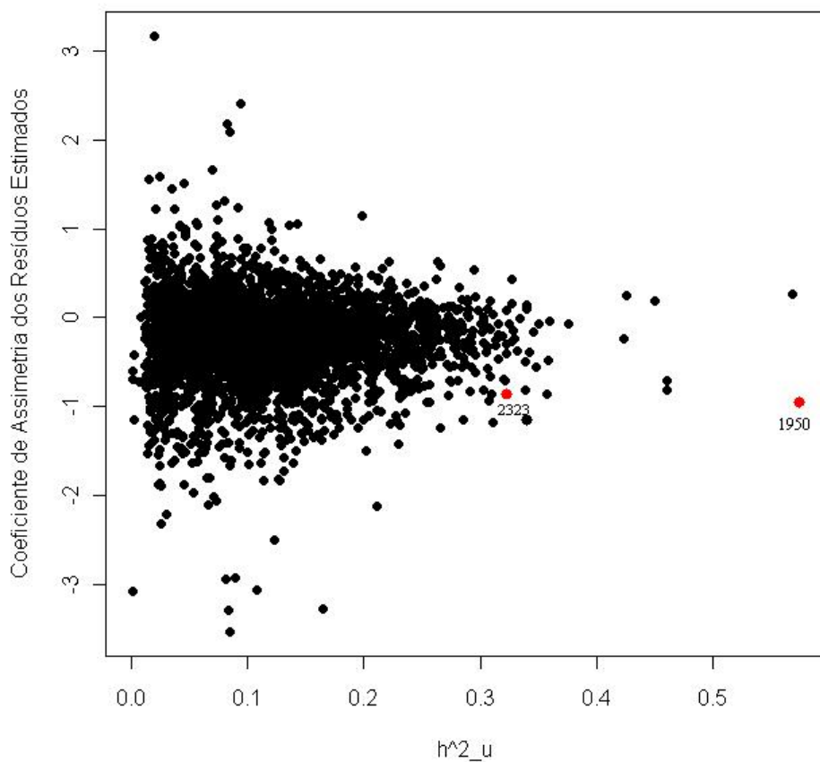
FIGURA 12 Diagrama de dispersão com os valores de \hat{h}_u^2 e os coeficientes de assimetria dos resíduos estimados para as 3554 sondas.
