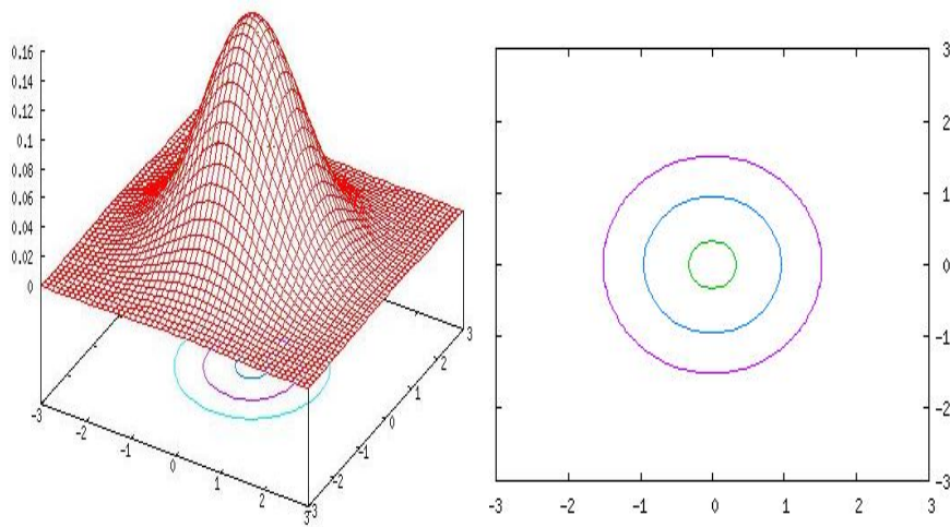
FIGURA 1 Distribuição SN_2((0,0)^\top, \text{diag}(1,1), \text{diag}(0,0)) com seu gráfico de contorno.
