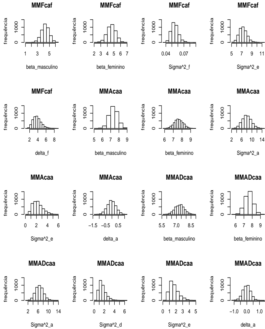
FIGURA 18 Histogramas das amostras a posteriori dos parâmetros \beta (sexo), \sigma^2 (variância) e \delta (assimetria, caso seja suposta no modelo) para os três melhores modelos através do FB, relativos às 16 configurações consideradas para a sonda 2323.
