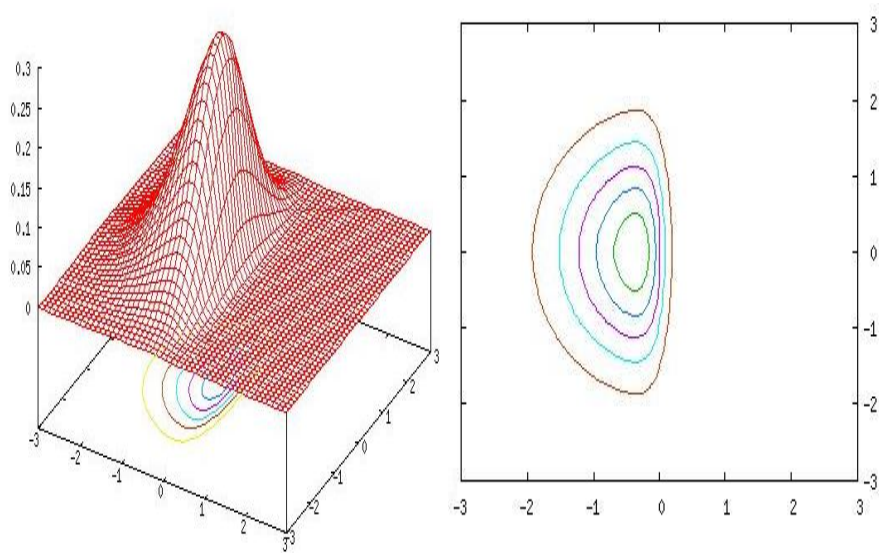
FIGURA 2 Distribuição SN_2((0,0)^\top, \text{diag}(1,1), \text{diag}(-5,0)) com seu gráfico de contorno.
