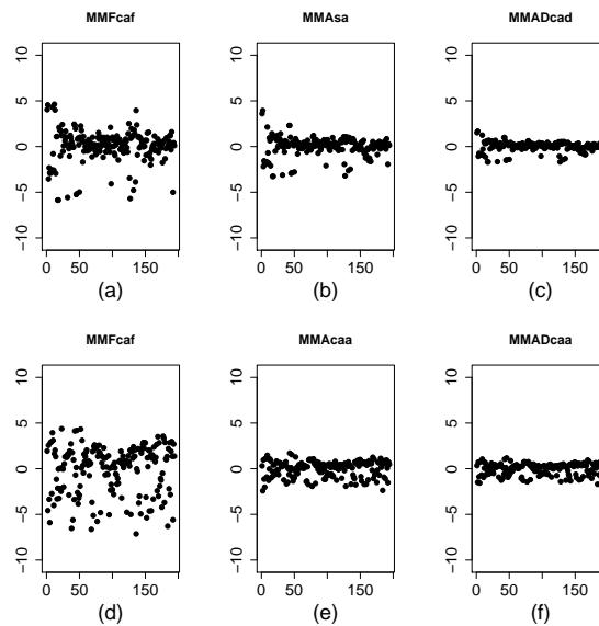
FIGURA 15 Índice das observações no eixo das abscissas versus os resíduos preditos no eixo das ordenadas. Os gráficos (a), (b) e (c) apresentam os resultados para a sonda 1950 e os gráficos (d), (e) e (f), para a sonda 2323.
