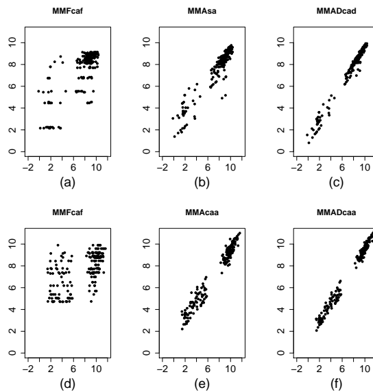
FIGURA 16 Valores observados no eixo das abscissas versus valores preditos no eixo das ordenadas. Os gráficos (a), (b) e (c) apresentam os resultados para a sonda 1950 e os gráficos (d), (e) e (f), para a sonda 2323.
