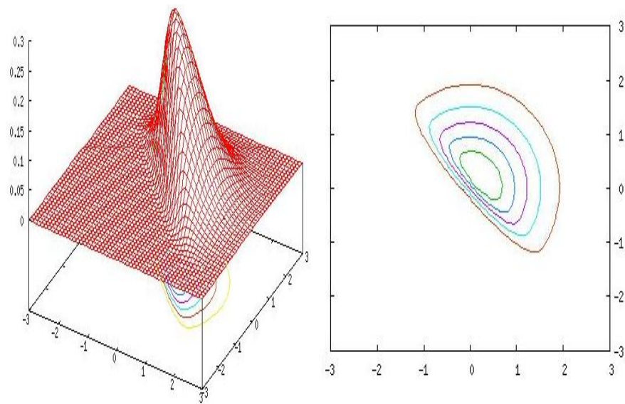
FIGURA 7 Distribuição SN_2((0,0)^\top, \text{diag}(1,1), \text{diag}(5,5)) com seu gráfico de contorno.
