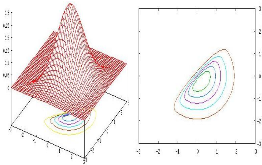
FIGURA 9 Distribuição SN_2((0,0)^\top, \text{diag}(1,1), \text{diag}(5,-5)) com seu gráfico de contorno.
