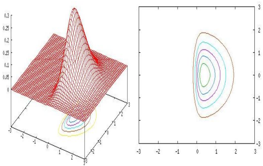
FIGURA 3 Distribuição SN_2((0,0)^\top, \text{diag}(1,1), \text{diag}(5,0)) com seu gráfico de contorno.
