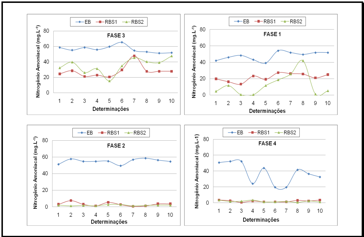
Figura 14 Comportamento da concentração de nitrogênio amoniacal do esgoto bruto e nos efluentes dos reatores.
