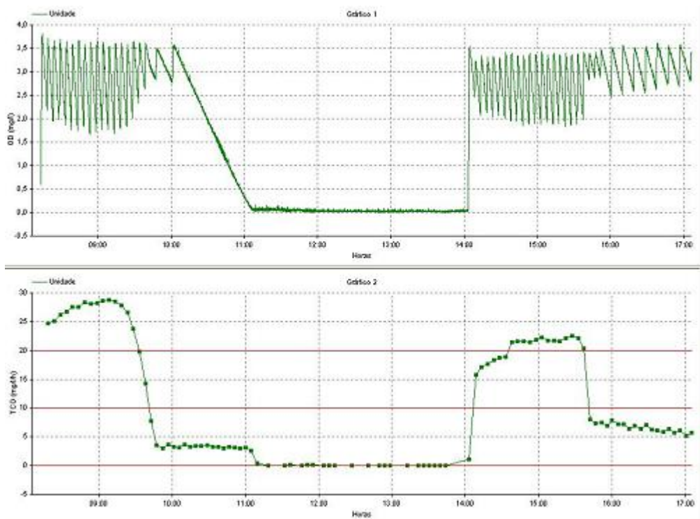
Figura 28 Respirograma obtido no sétimo teste com lodo do RBS1
