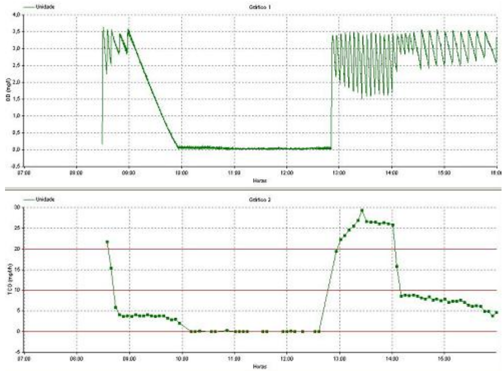
Figura 27 Respirograma obtido no sexto teste com lodo do RBS1.
