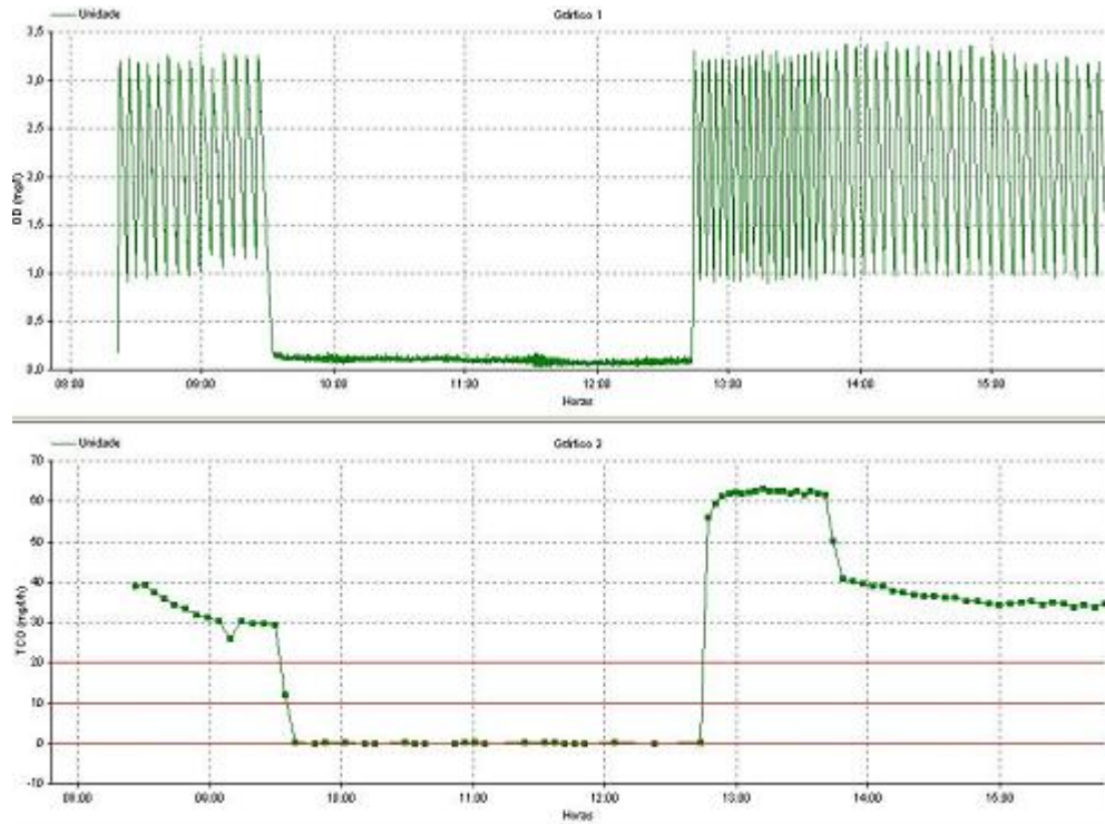
Figura 31 Respirograma obtido no terceiro teste com lodo do RBS2.
