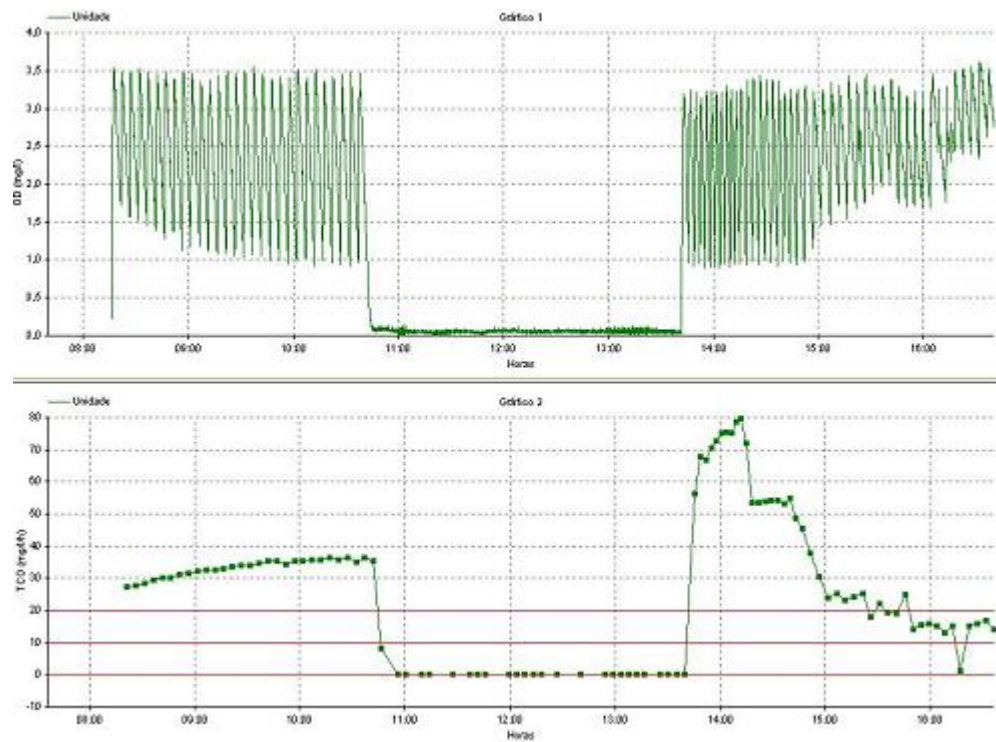
Figura 30 Respirograma obtido no segundo teste com lodo do RBS2.
