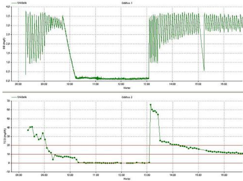
Figura 33 Respirograma obtido no quinto teste com lodo do RBS2.
