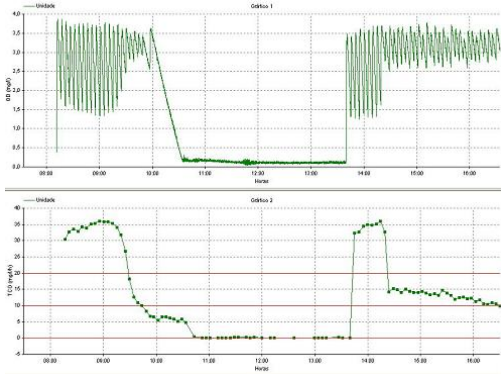
Figura 35 Respirograma obtido no sétimo teste com lodo do RBS2.
