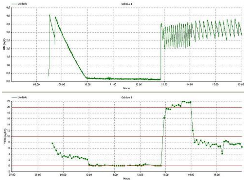
Figura 34 Respirograma obtido no sexto teste com lodo do RBS2
