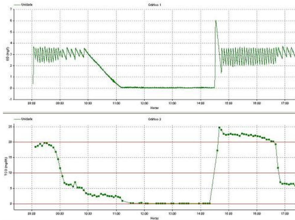
Figura 32 Respirograma obtido no quarto teste com lodo do RBS2
