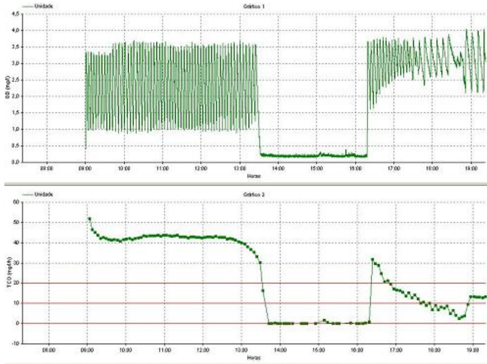
Figura 29 Respirograma obtido no primeiro teste com lodo do RBS2.
